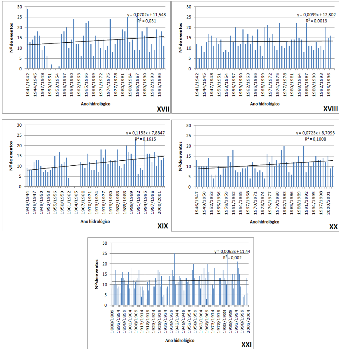
Figura 61: Número de eventos anual maiores que 30 mm/dia. I) Guarulhos; II) Cachoeira da Graça; III) Franco da Rocha; IV) Guararema; V) Itaquaquecetuba; VI) Mairiporã; VII) Pedro Beith; VIII) Barueri; IX) Salesópolis; X) Santa Isabel; XI) Usina Salesópolis; XII) IAG; XIII) Perus; XIV) Santana; XV) Santo Amaro; XVI) Água Branca; XVII) Barrocada; XVIII) Engordador; XIX) Instituto Biológico; XX) Congonhas Aeroporto e XXI) Estação da Luz. Fonte: Autor, 2011.
