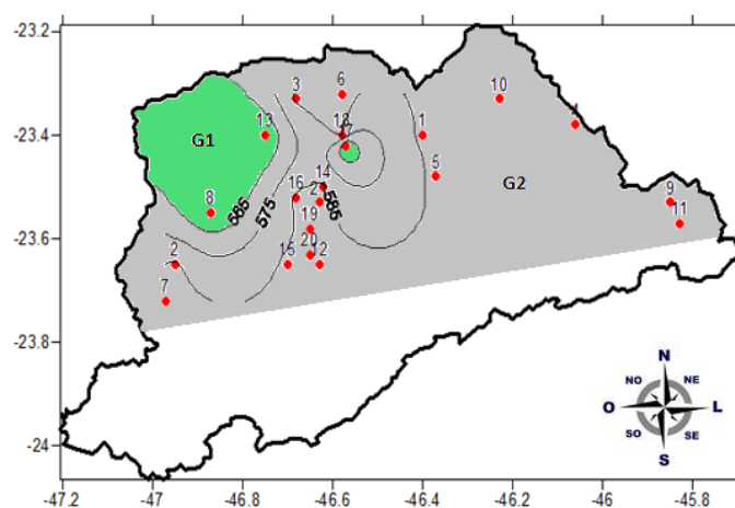
Figura 18: Isolinhas do total médio anual de precipitação da classe moderada. Fonte: Autor, 2011.
