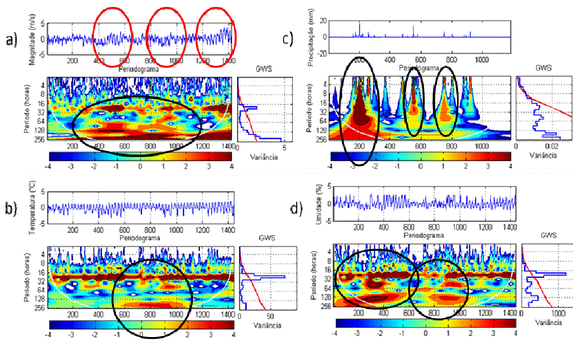
Figura 24 – Espectro de ondeleta no período de transição chuvoso-seco para as variáveis a) Magnitude do vento; b) Temperatura do ar; c) Precipitação; d) UR.
