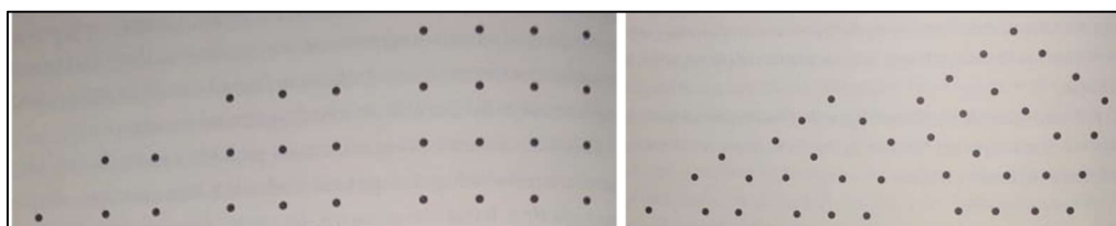
Figura 2: Números quadrados e Números pentagonais
