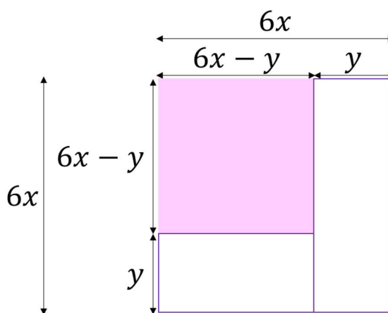
Figura 62: Representação geométrica de (6x - y)^2
