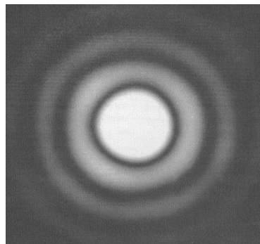
Figura 2.5 — Padrão de difração de Fraunhofer de uma abertura circular
