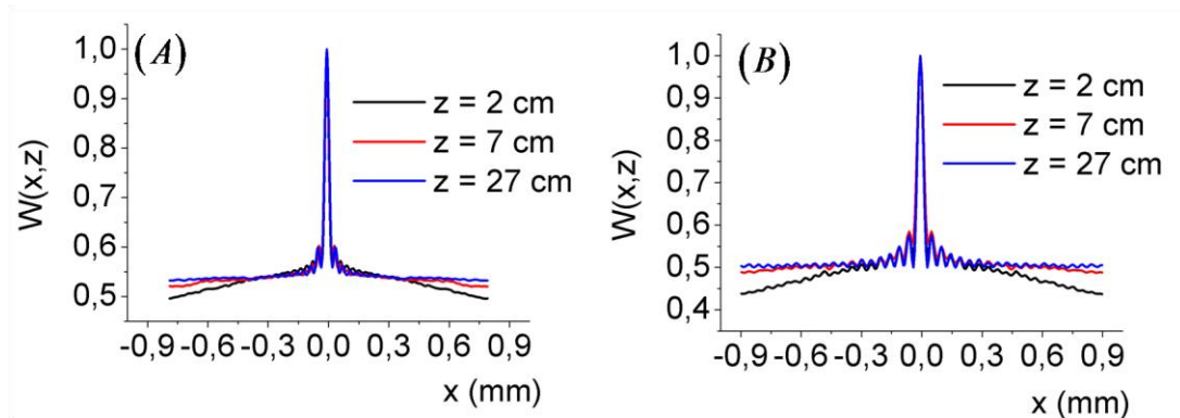
Figura 4.4-2 – Perfis das medidas de autocorrelação ao longo de diferentes distâncias de propagação com obstáculo para o feixe Bessel parcialmente coerente: experimento (A) e simulação (B).
