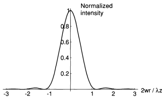
Figura 2.4 — Seção transversal do padrão de difração de Fraunhofer de uma abertura circular.
