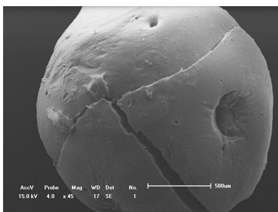
(e) Esfera de quitosana glutaraldeído. Aumento de 45x.
