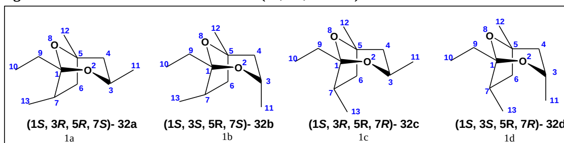
Figura 4 – Estereoisômeros da sordidina (1a, 1b, 1c e 1d)
