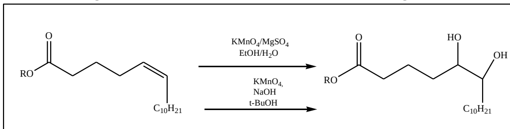
Figura 12 – Metodologia de diidroxilação utilizando Permanganato de Potássio
