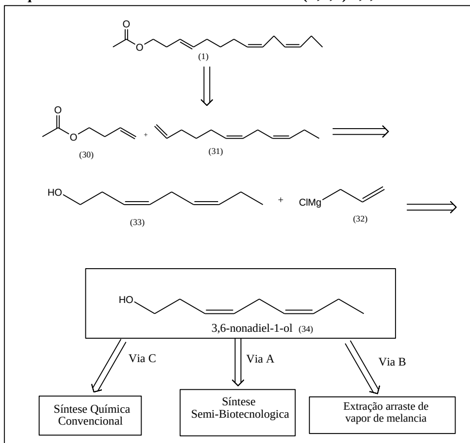
Figura 6 – Esquema da análise retrossíntese do acetato de ( E,Z,Z )-3,8,11-tetradecatrienila
