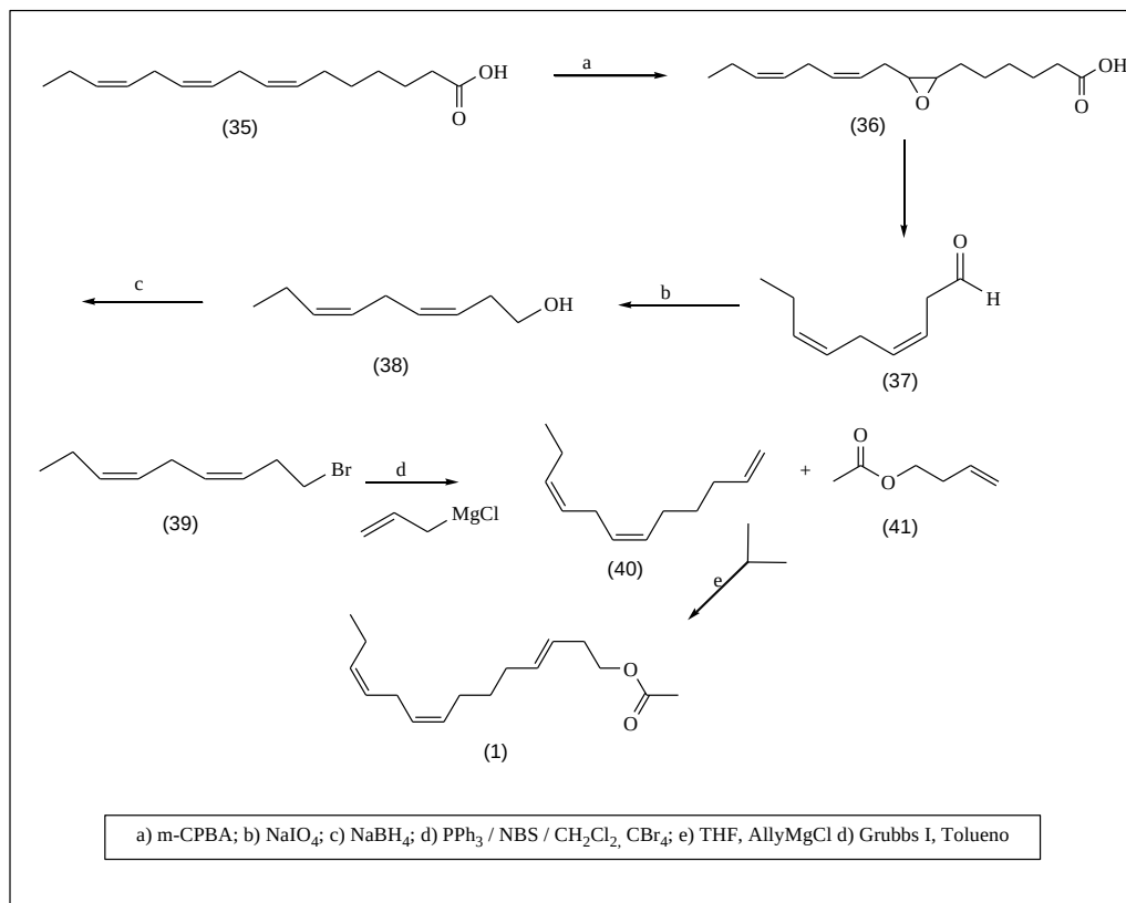
Figura 7 – Esquema da síntese semi-biotecnológica usando óleo de linhaça como material de partida
