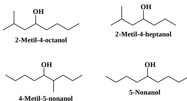
Figura 2 – Moléculas constituintes do feromônio do M. hemipterus
