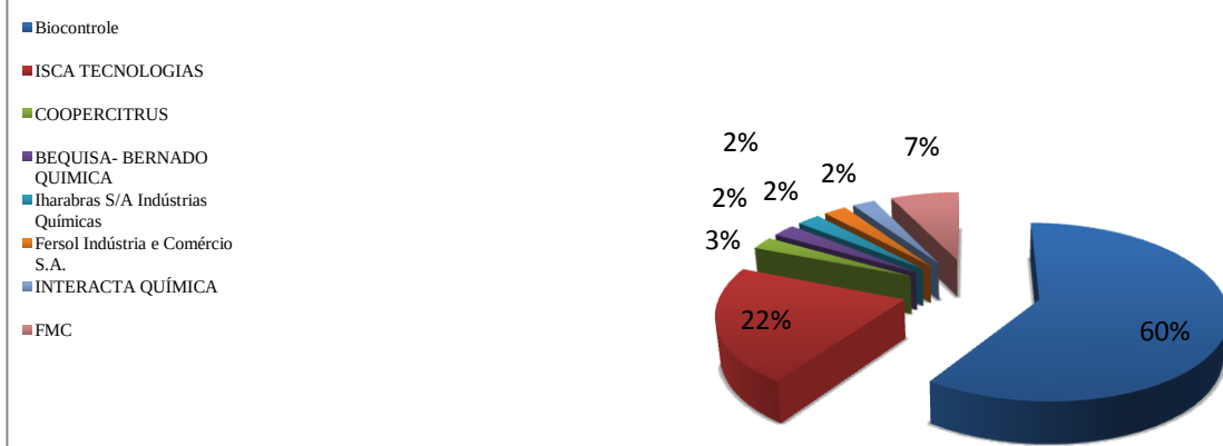
Figura 4 – Empresas responsáveis pela comercialização de feromônios
