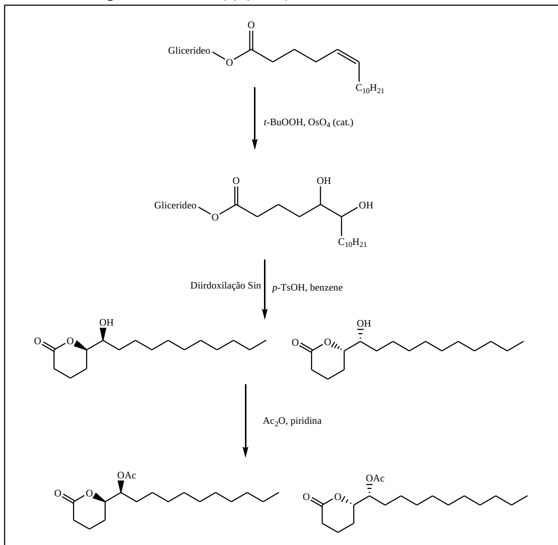
Figura 4 – Esquema de síntese do (-)-(5 R ,6 S )-6-acetoxi-5-hexadecanolídeo e seu enantiômero biologicamente inativo (+)-(5 S ,6 R )-6-acetoxi-5-hexadecanolídeo.
