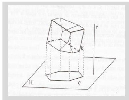
Figura 17 - A região iluminada e a região sombria.
