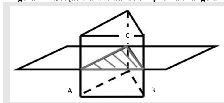
Figura 22 - Secção transversal de um prisma triangular.
