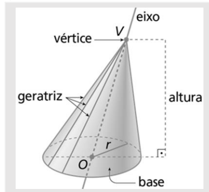
Figura 35: Elementos do cone circular
