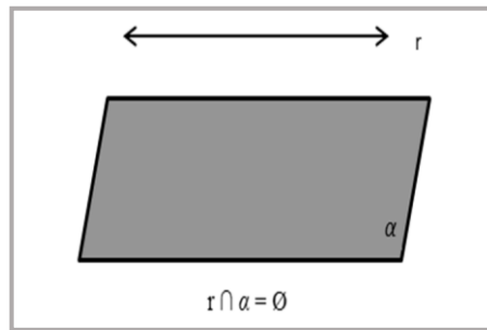
Figura 9 - Reta paralela ao plano.
