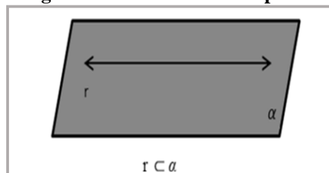
Figura 11 - Reta contida no plano.
