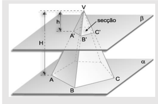
Figura 27 - Secção transversal de uma pirâmide pentagonal.
