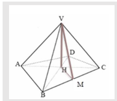
Figura 29: Apótema da pirâmide regular e apótema da base.
