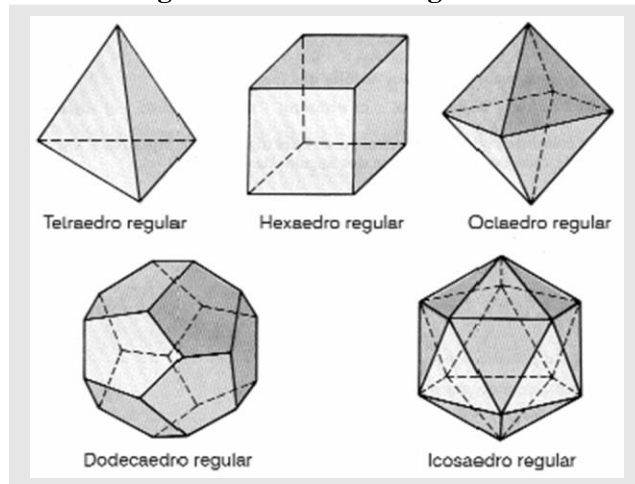
Figura 19 - Poliedros regulares.
