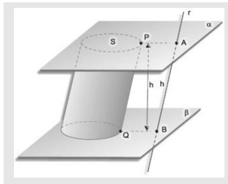
Figura 30 - Cilindro.
