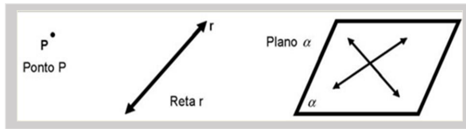
Figura 1 - Representação de ponto, reta e plano.
