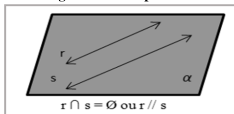
Figura 2- Retas paralelas.
