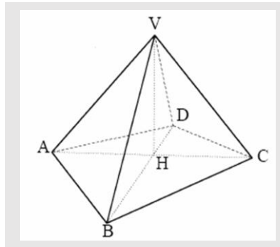
Figura 28 - Pirâmide quadrangular regular.
