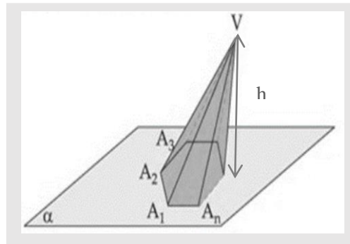
Figura 25 - Pirâmide.
