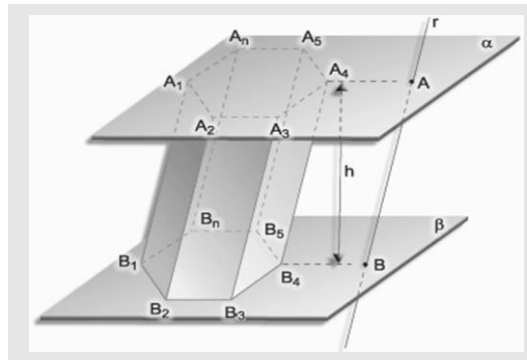
Figura 20 - Prisma.
