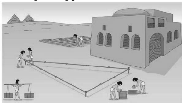
Figura - Egípcios medindo a terra
