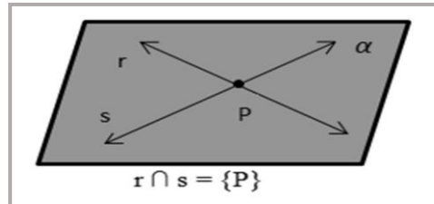
Figura 3 - Retas concorrentes.
