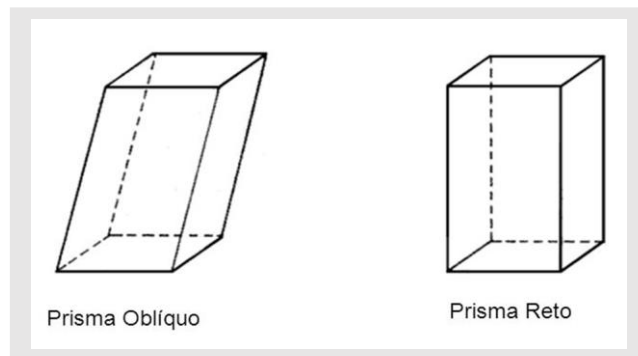
Figura 23 - Prisma obluo e prisma reto.
