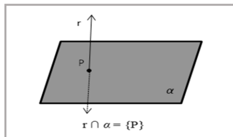
Figura 10 - Reta secante ao plano.
