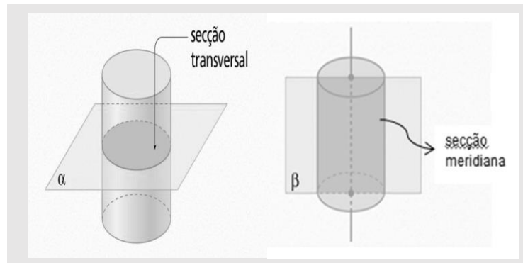
Figura 32 - Secção transversal e secção meridiana de um cilindro.
