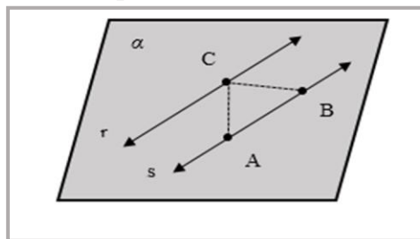
Figura 8 - Duas retas paralelas distintas determinam um plano.
