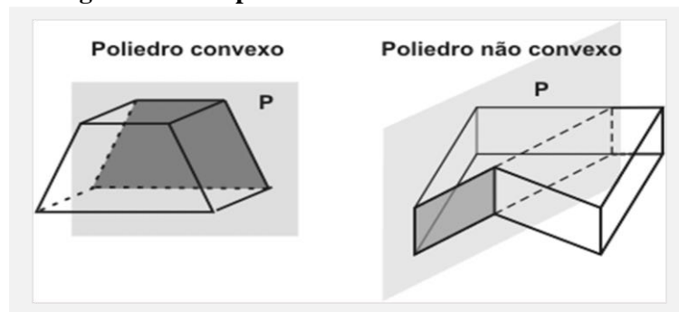
Figura 16 - Um poliedro convexo e um não convexo.
