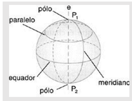
Figura 38 - Elementos da Esfera
