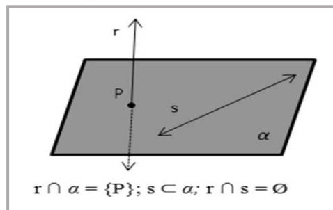
Figura 4 - Retas reversas.
