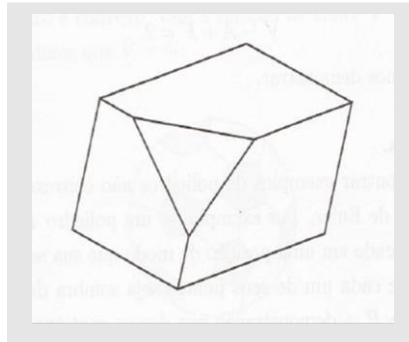
Figura 18 - A sombra das faces iluminadas.
