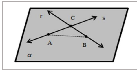
Figura 7 - Duas retas concorrentes determinam um plano.
