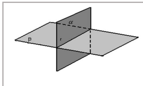
Figura 13 - Planos secantes.
