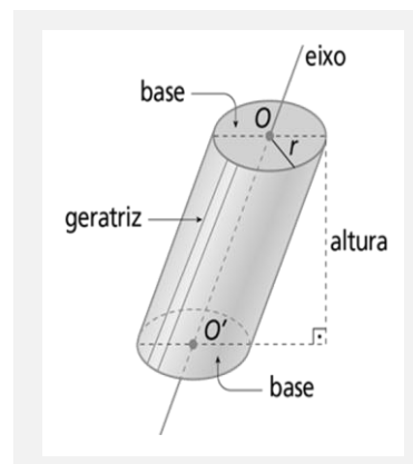
Figura 31 - Elementos do cilindro.
