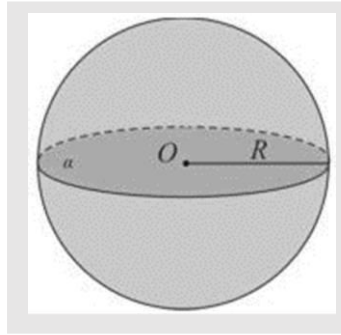
Figura 37 - Esfera.
