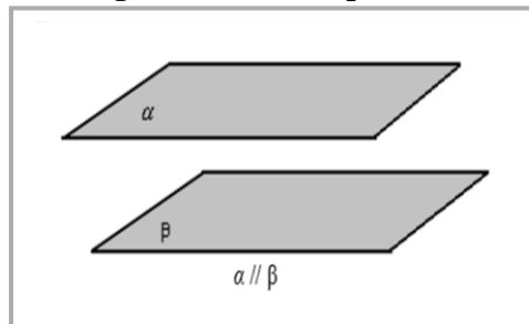
Figura 12 - Planos paralelos.
