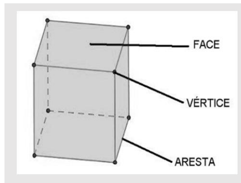
Figura 14 - Face, aresta e vértice de um cubo.
