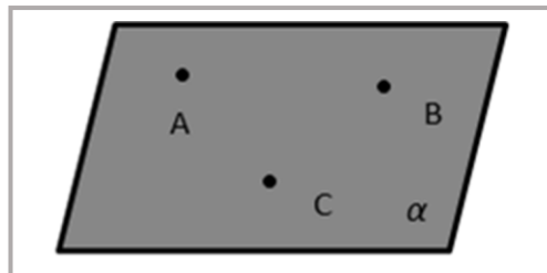
Figura 5 - Três pontos não colineares determinam um plano.
