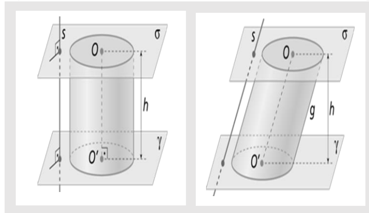
Figura 33 - Cilindro circular reto e cilindro circular oblíquo.
