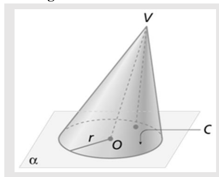
Figura 34 - Cone circular.
