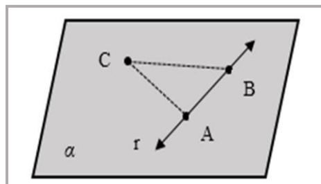
Figura 6 - Uma reta e um ponto não pertencente a ela determinam um plano.
