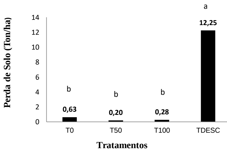
Figura 5. Análise de variância para perdas de água em um Argissolo Amarelo, cultivado com cana de açúcar sob diferentes proporções de palhada em superfície.
