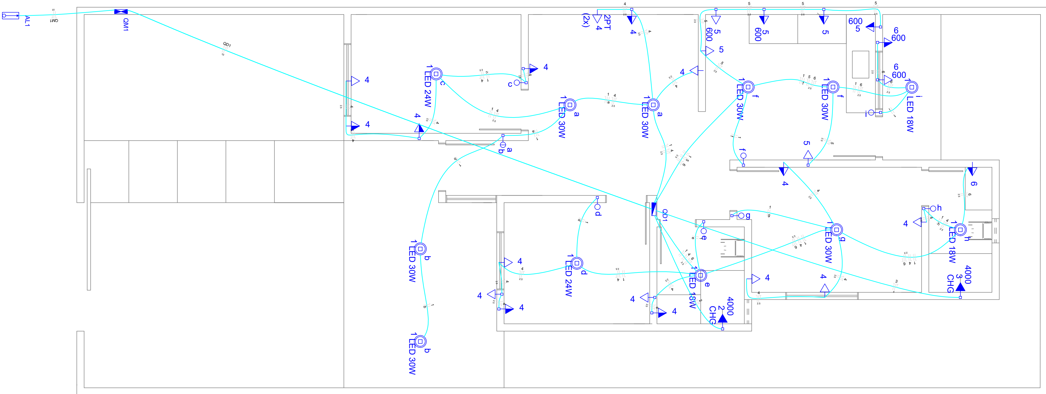
01 PLANTA BAIXA - ESQUEMA GERAL ELÉTRICO Escala 1/100
