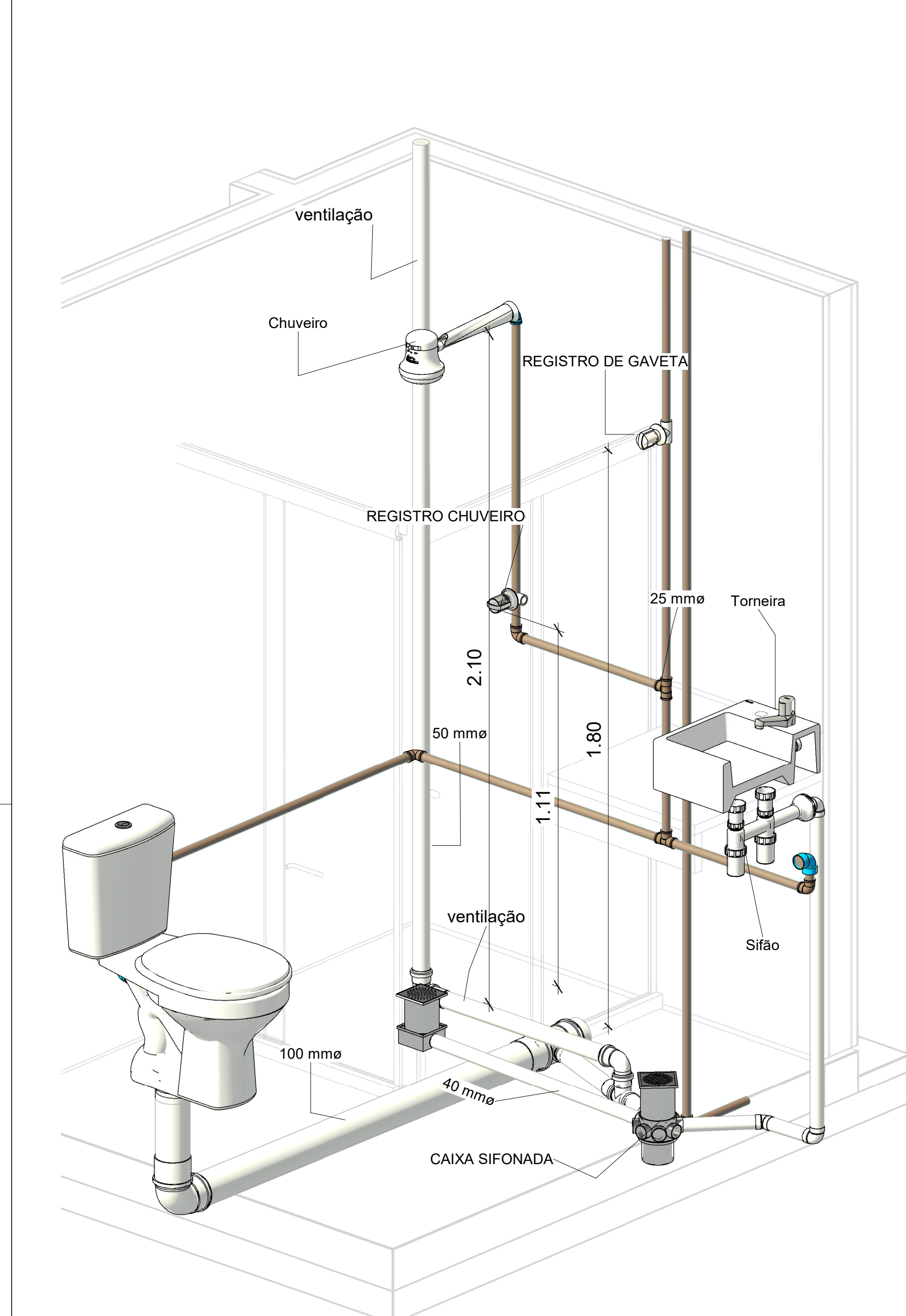
1 ISOMÉTRICO - BANHO 1
