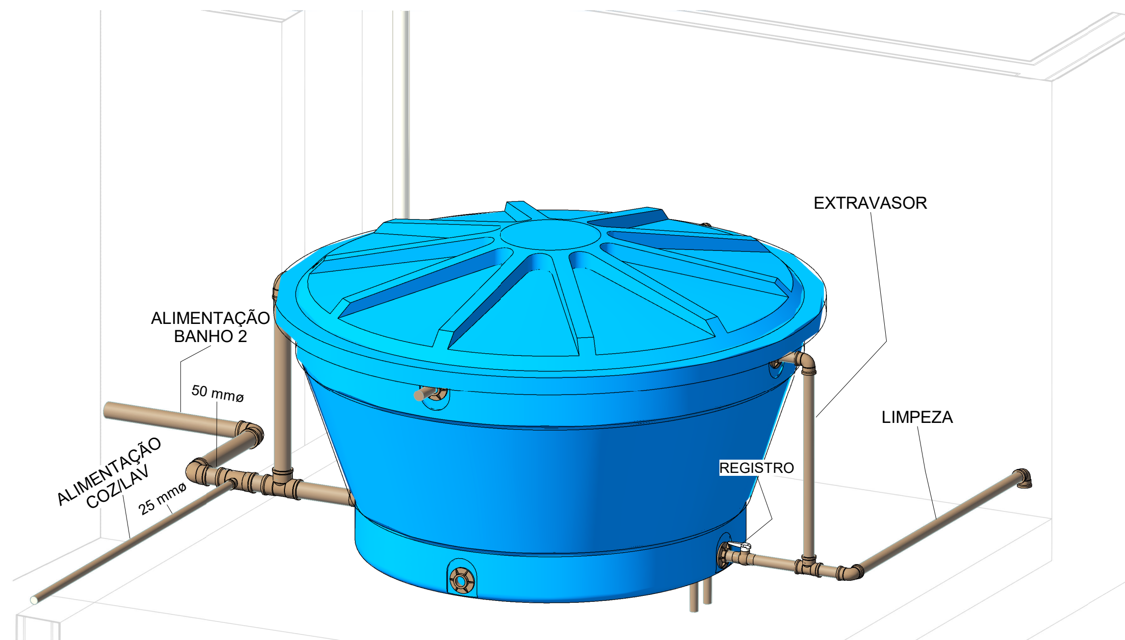
6 ISOMÉTRICO CAIXA D'ÁGUA 2
