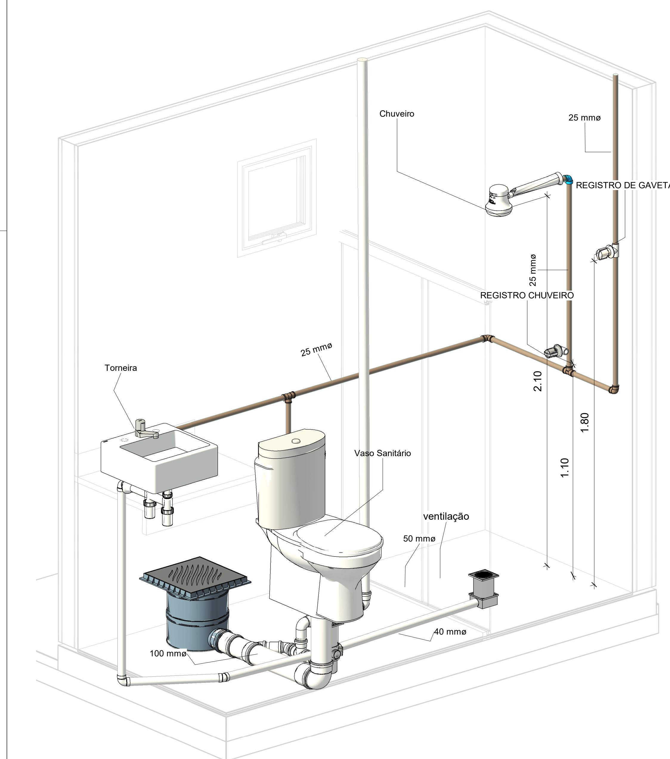
2 ISOMÉTRICO - BANHO 2
