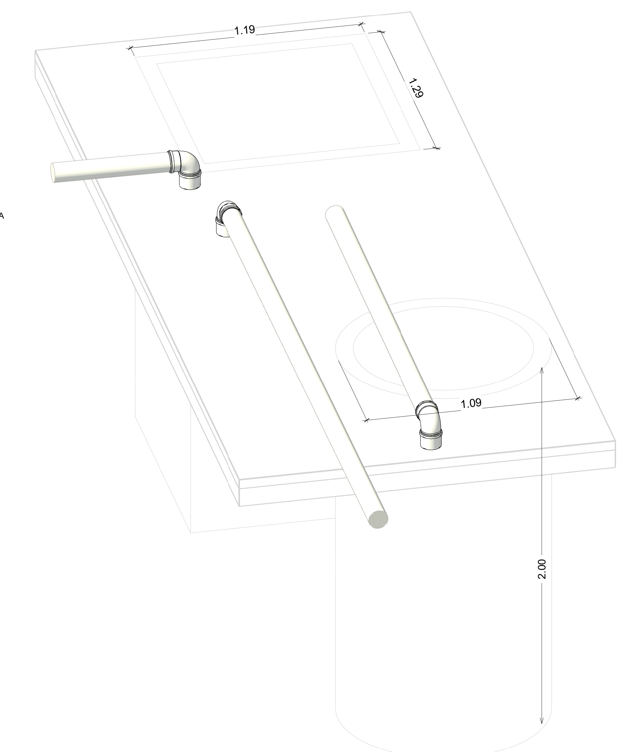
4 ISOMÉTRICO VISTA FOSSA E SUMIDOURO
