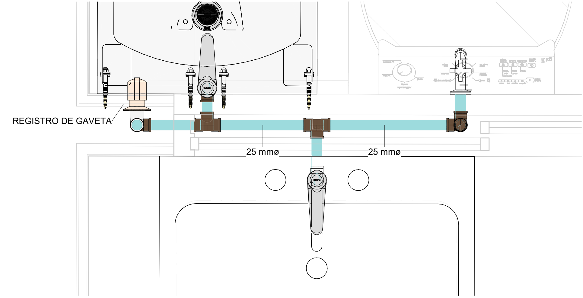
7 DETALHE - LAV/COZ 1 : 5
