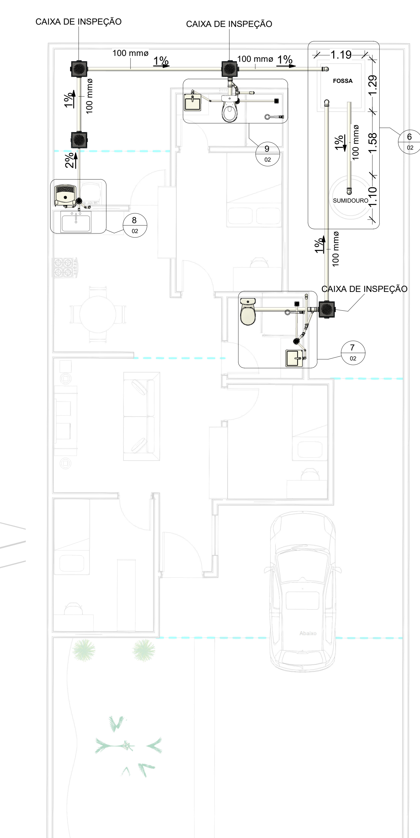
5 ESGOTO - TÉRREO
