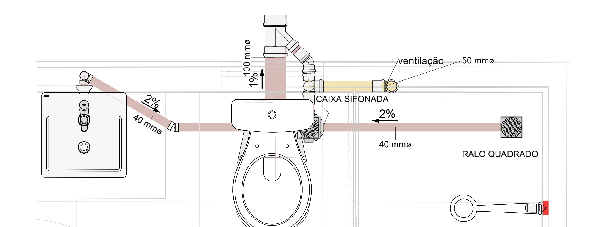
9 ESGOTO - DETALHE BANHO 2
