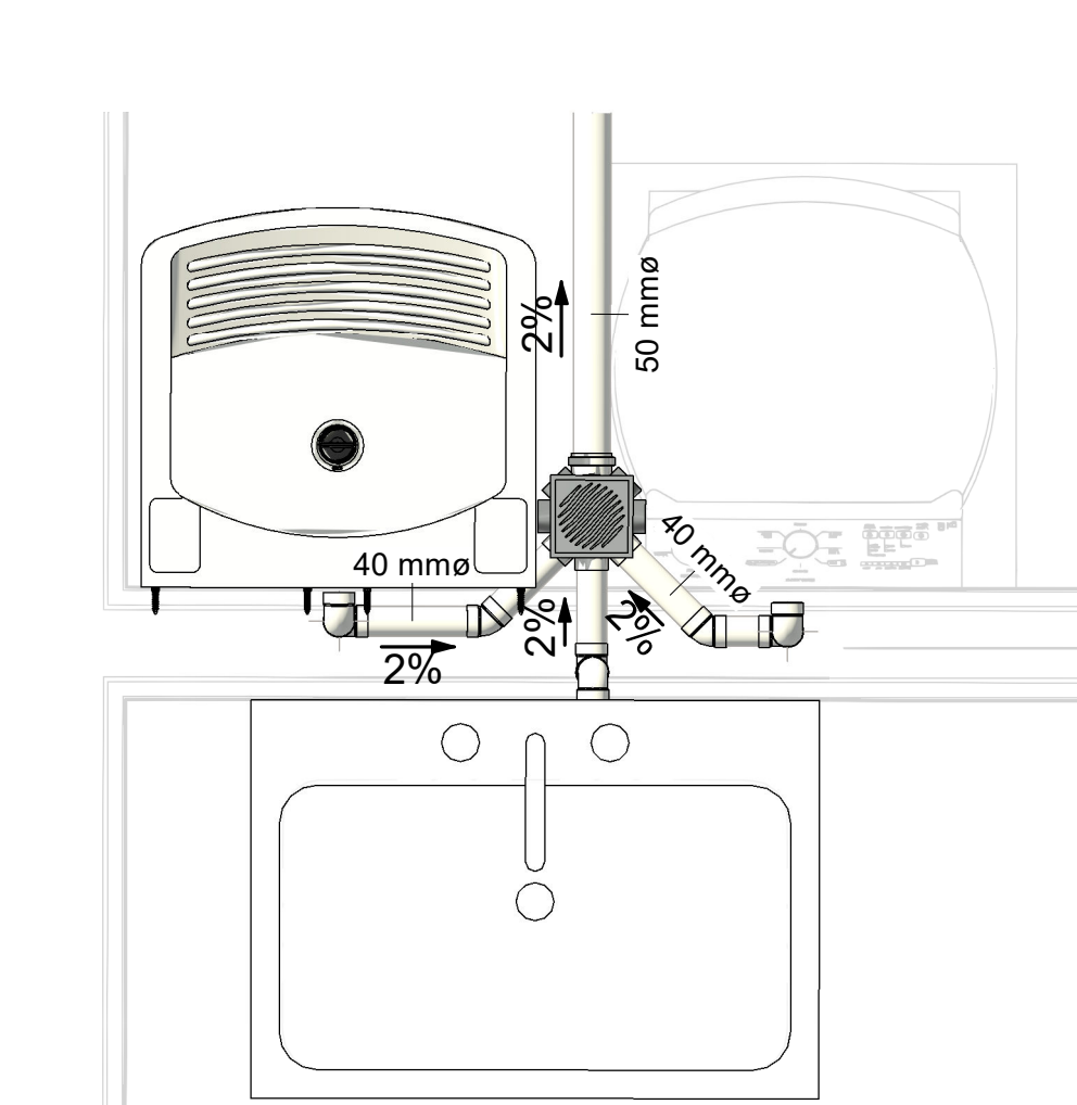
8 ESGOTO - DETALHE LAV/COZ
