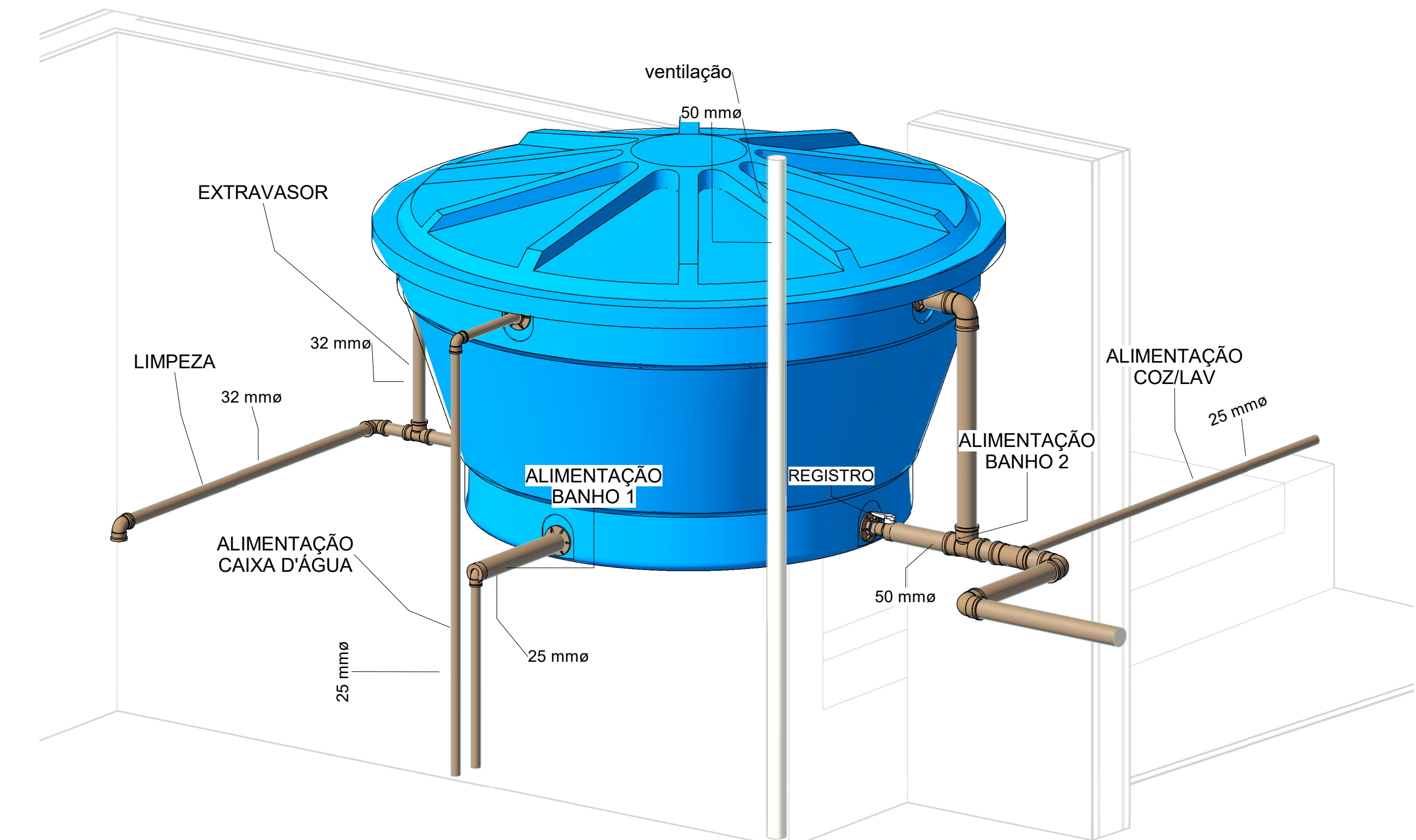
5 ISOMÉTRICO CAIXA D'ÁGUA
