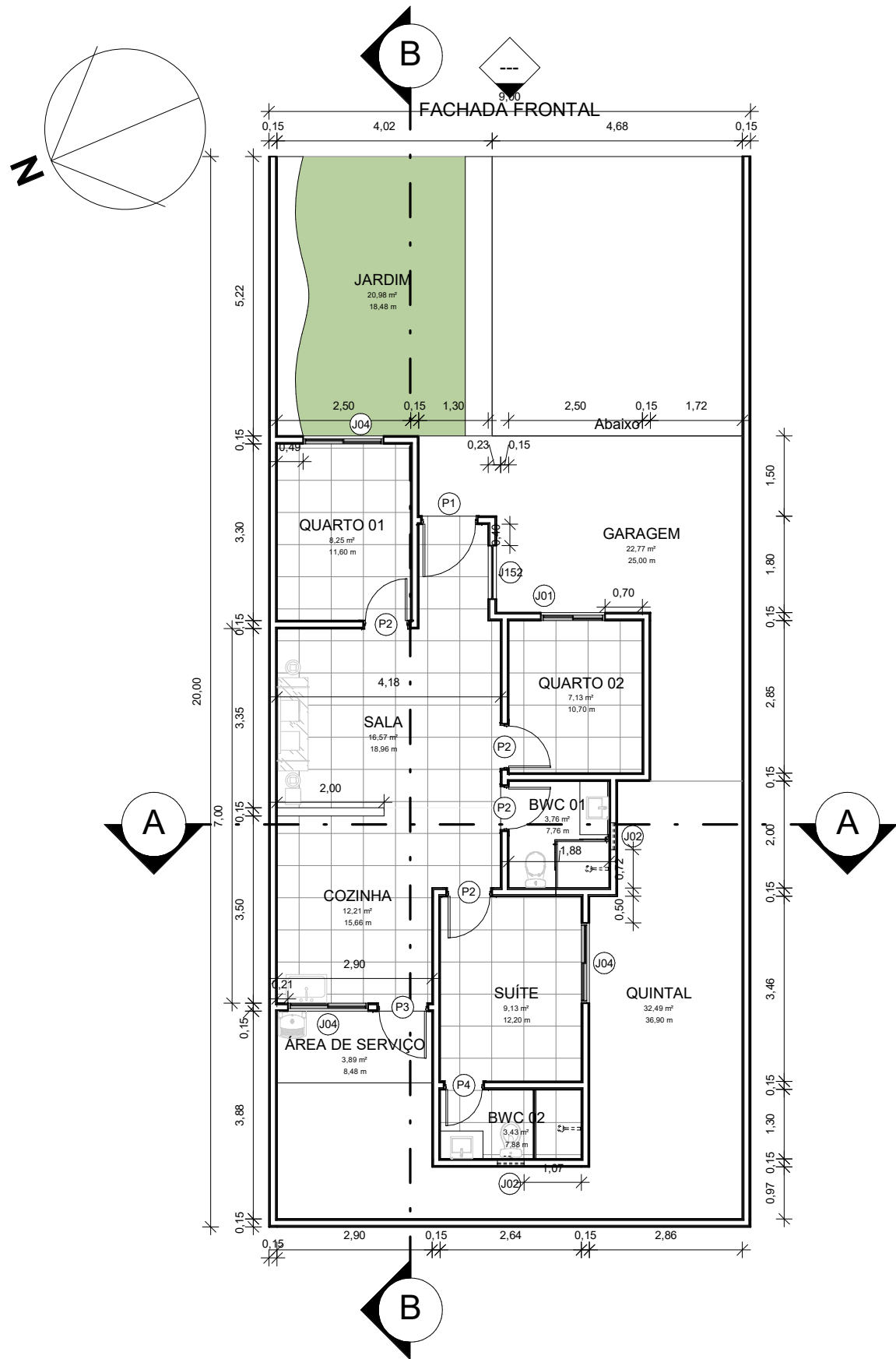
3 PLANTA - TÉRREO Escala: 1 : 100
