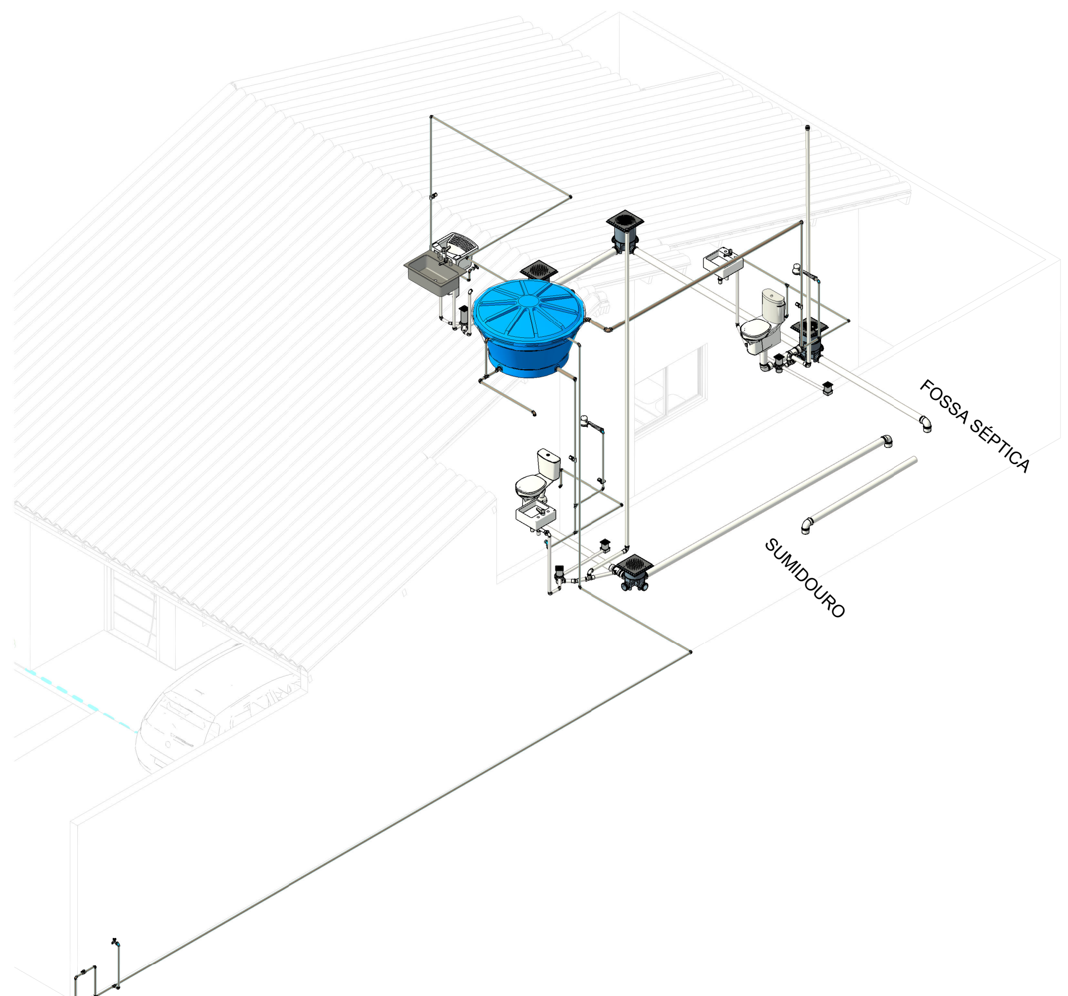
2 GERAL - ISOMÉTRICO VISTA 1
