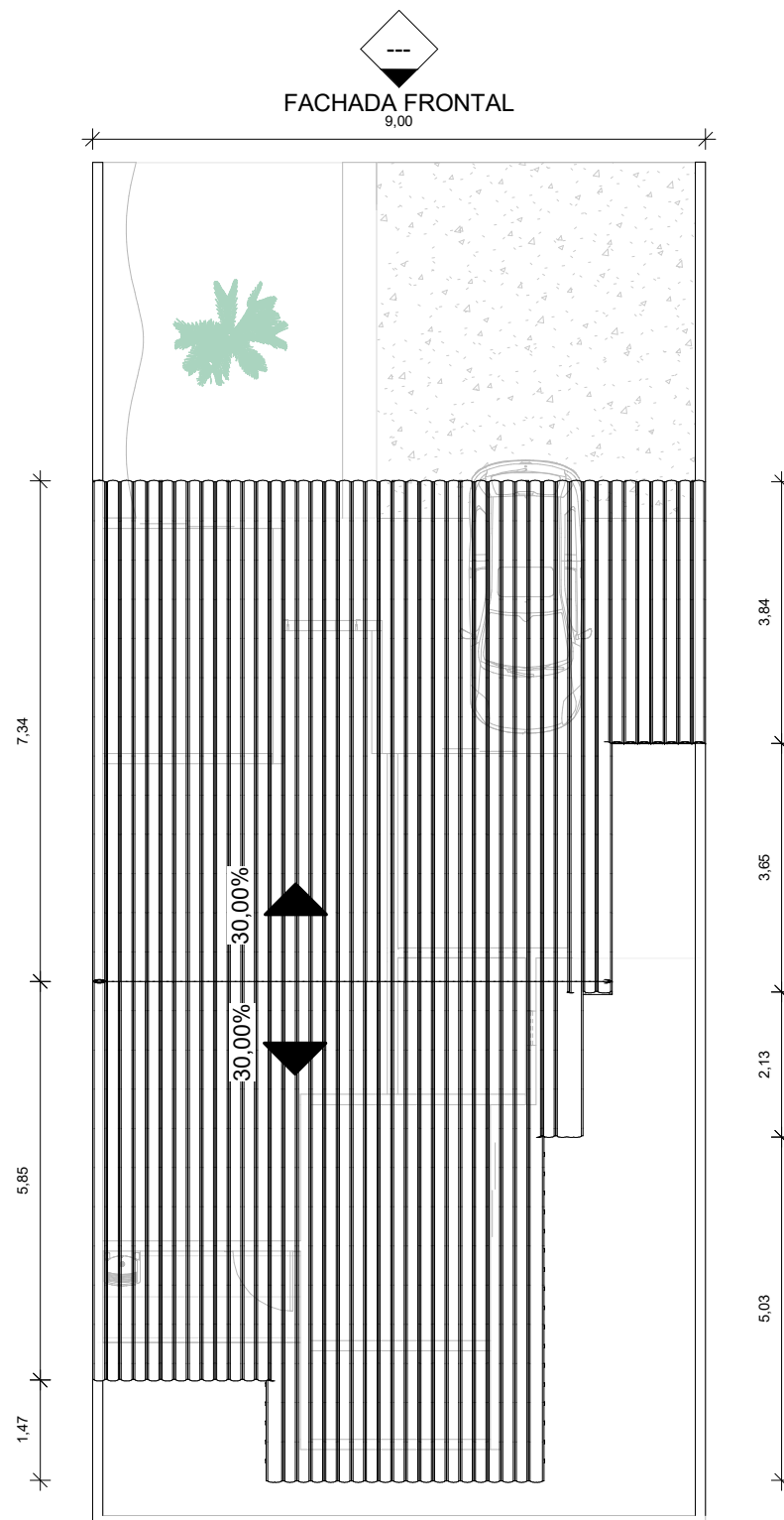
5 PLANTA DE IMPLANTAÇÃO E COBERTA Escala: 1 : 100
