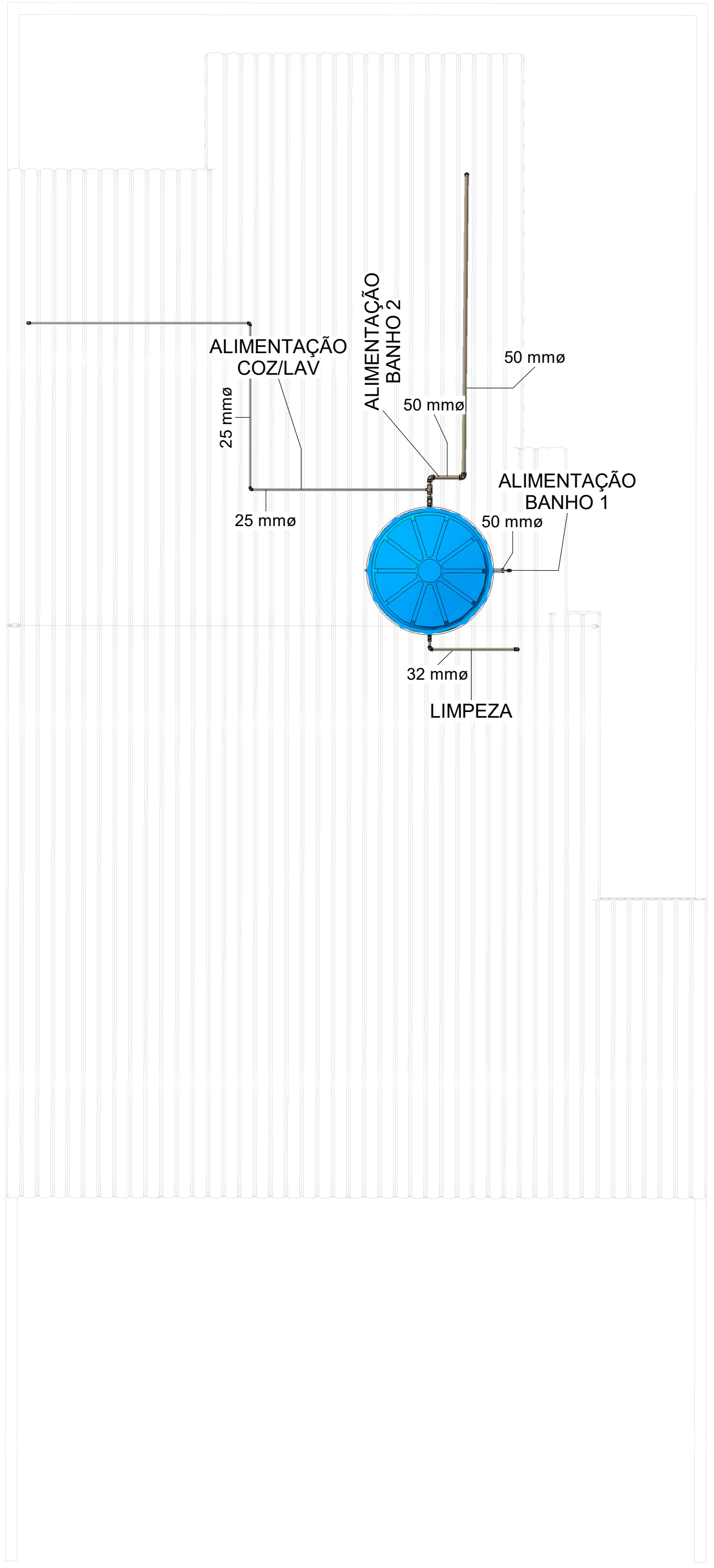
3 NÍVEL 2 (AF) 1 : 50
