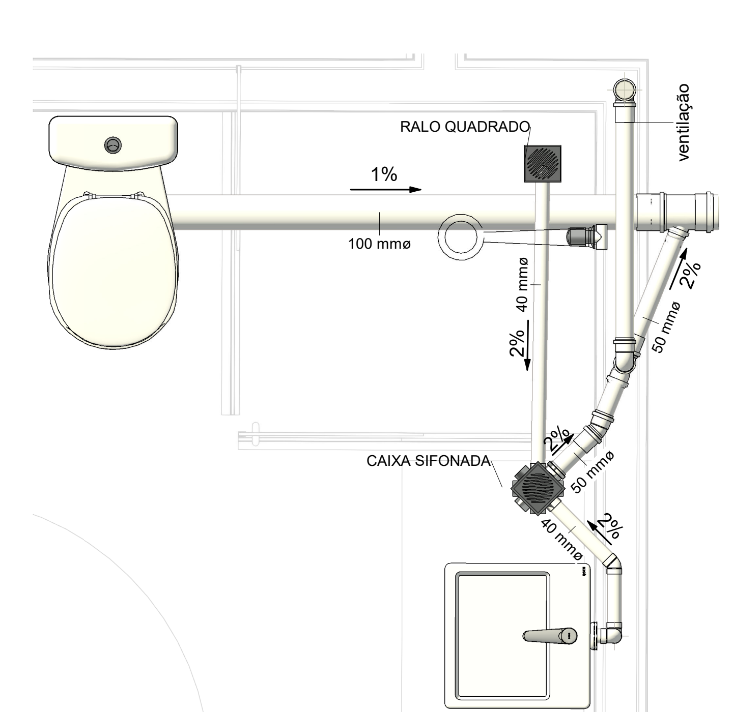
7 DETALHE - BANHO 1
