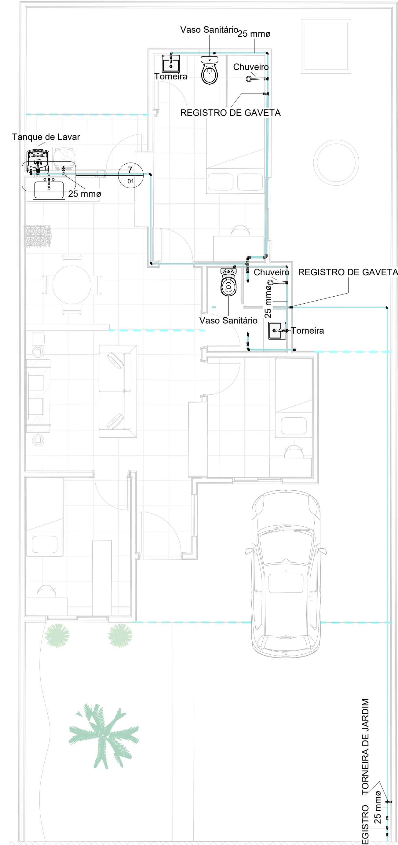
1 ÁGUA FRIA - TÉRREO 1 : 50
