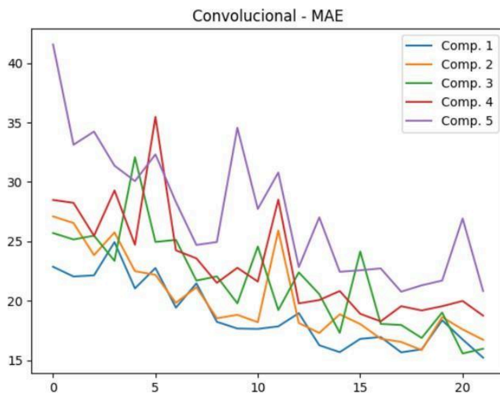
Figura 5.1: Gráfico de convergência do modelo convolutacional
