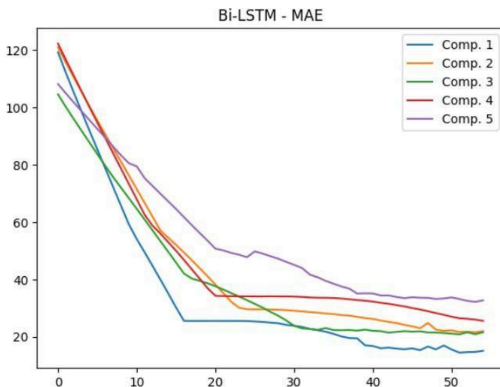
Figura 5.2: Gráfico de convergência do modelo recorrente LSTM Bidirecional
