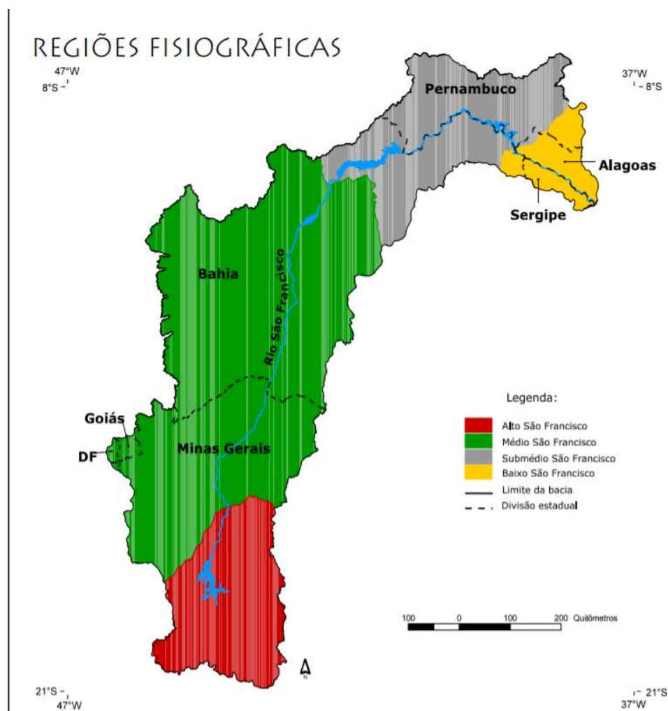
Figura 1 - Unidades hidrográficas de referência e divisão fisiográfica da Bacia do Rio São Francisco
