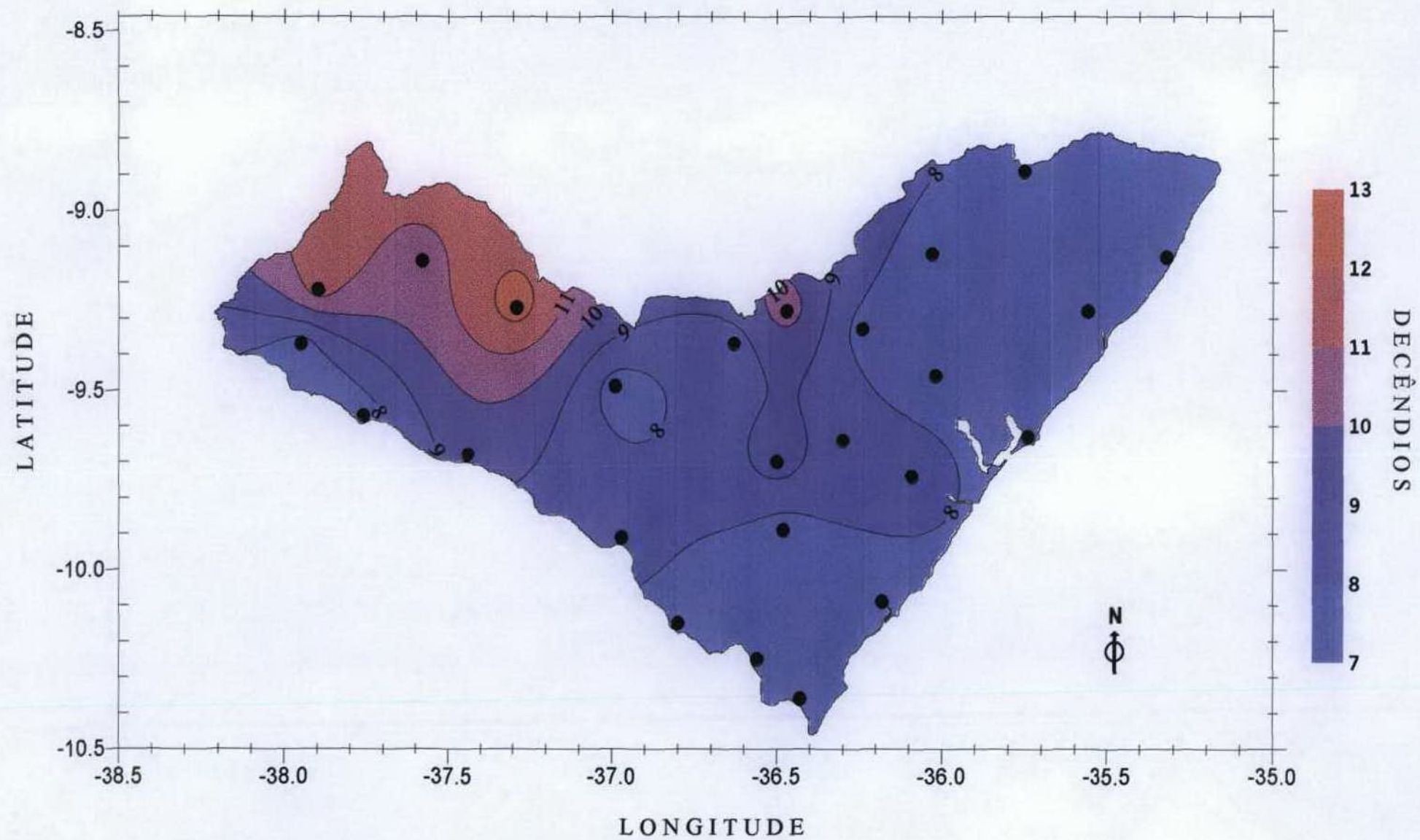
Figura 7 - Início da estação de cultivo referente ao método médio para o período de 1913 a 1985.
