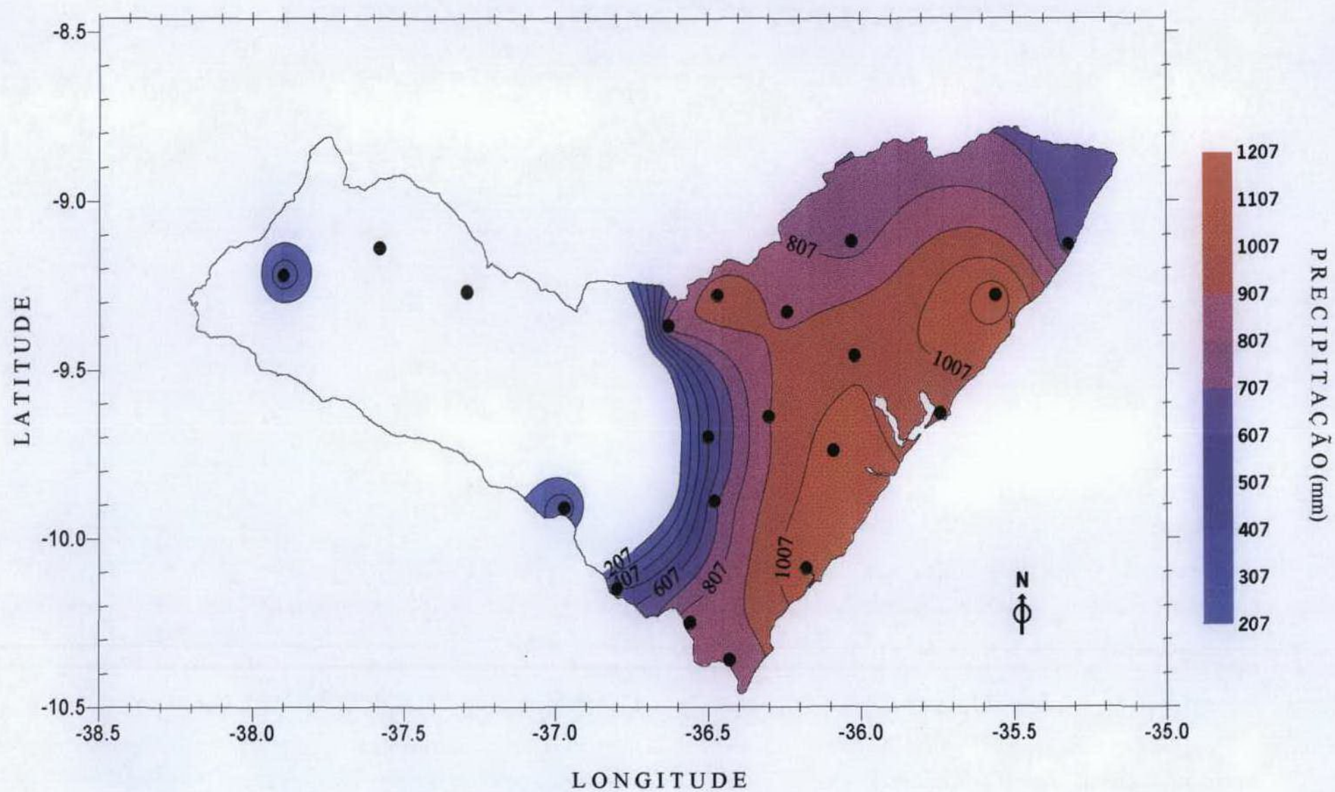
Figura 56 - Precipitação total média da estação de cultivo referente ao método da precipitação provável a 75 % de probabilidade e evapotranspiração para o período de 1913 a 1959.
