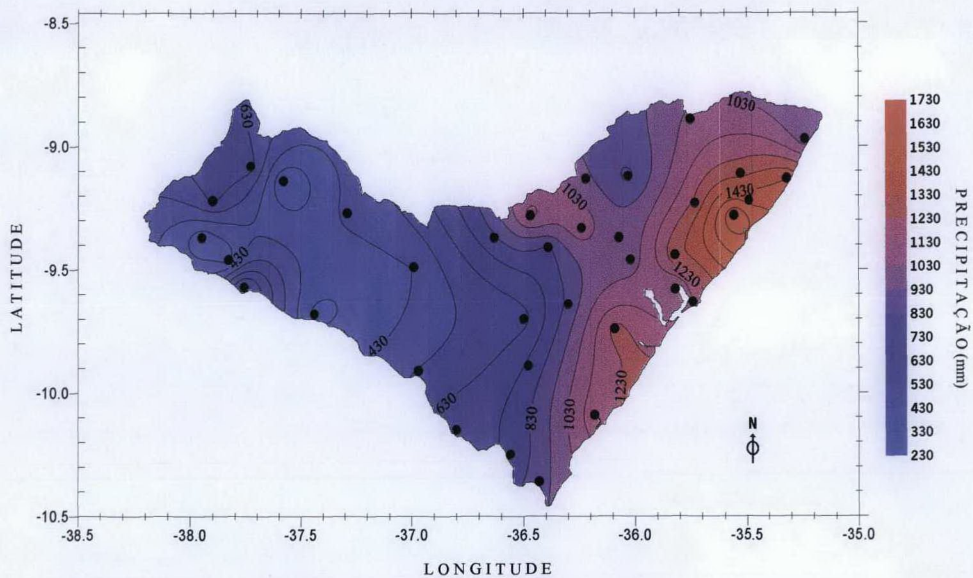
Figura 47 - Precipitação anual referente a 50 % (mediana) para o período de 1960 a 1985.
