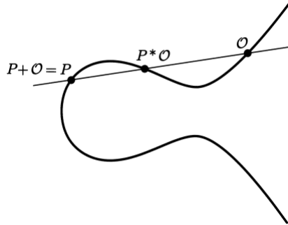
Figura 2 – Elemento Neutro
