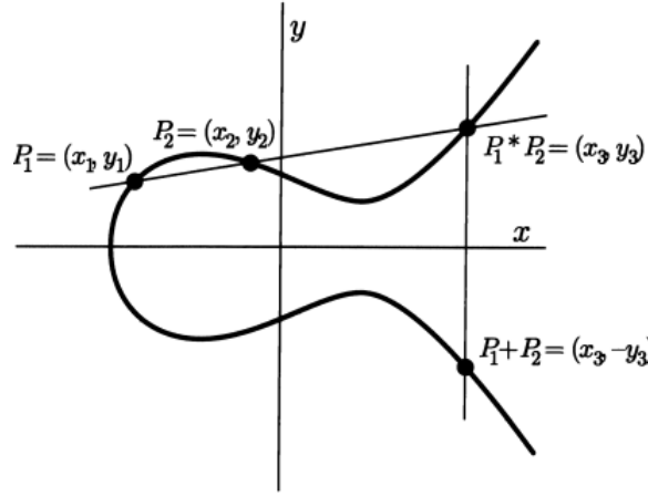
Figura 7 – Derivando a fórmula para a lei de adição
