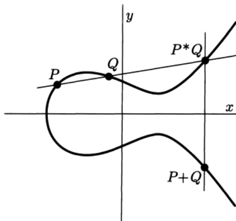
Figura 5 – Adicionando pontos na forma normal de Weierstrass
