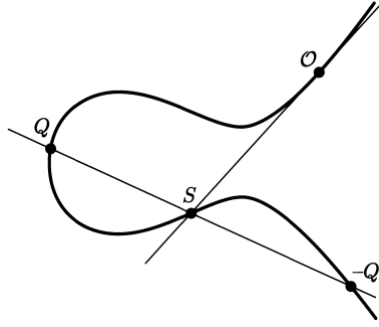
Figura 3 – Inverso
