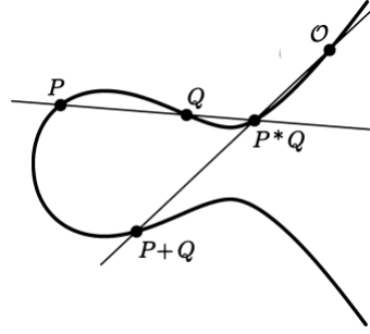
Figura 1 – Comutatividade
