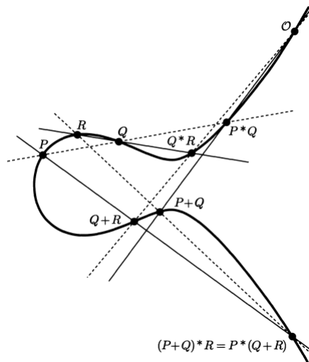
Figura 4 – Associatividade
