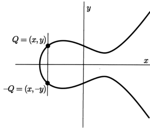
Figura 6 – O ponto negativo
