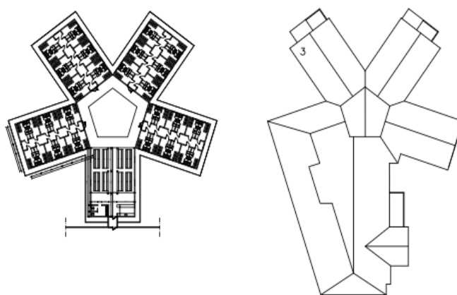
FIGURA 9 - Planta da Casa de Albergado antes e depois de se tornar o EPFSL. Fonte: Arquivo pessoal de Suzann Cordeiro. Autoria do desenho: Núcleo de Pesquisas sobre Projetos Especiais - NIJPPES. FAUJ-UFAL. 2013.
