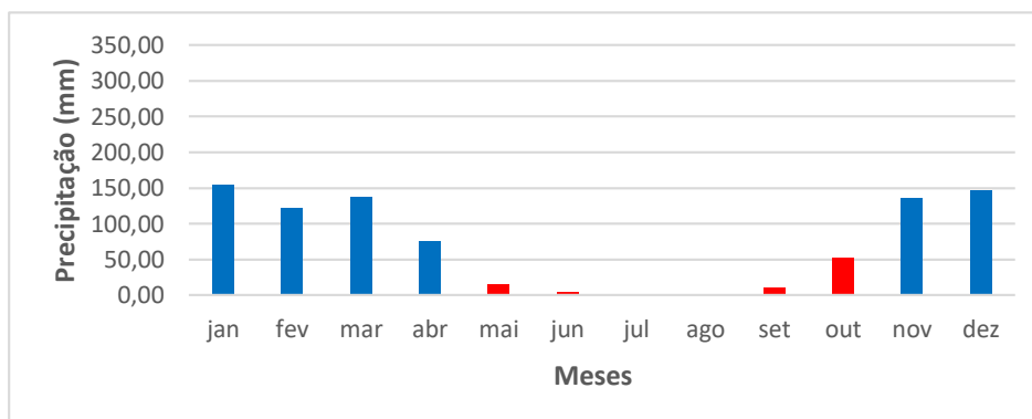
Figura 7: Média climatológica para o MSF de 1968 a 2020.
