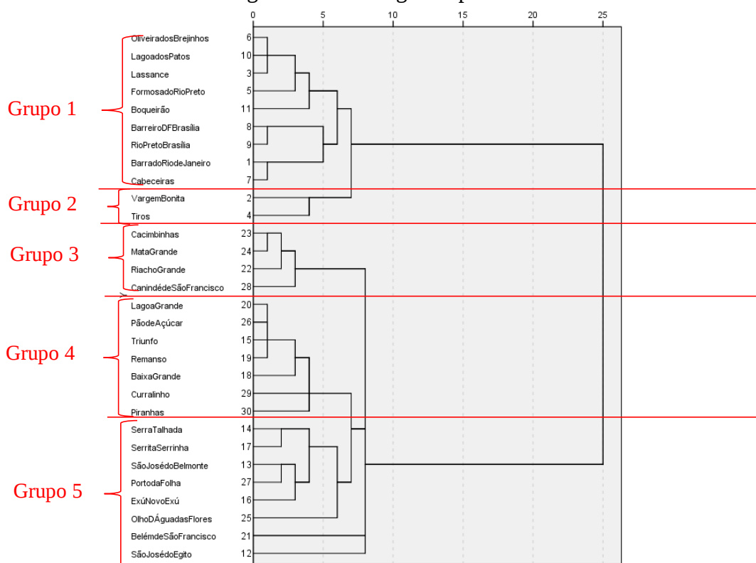
Figura 32: Dendrograma para o inverno.
