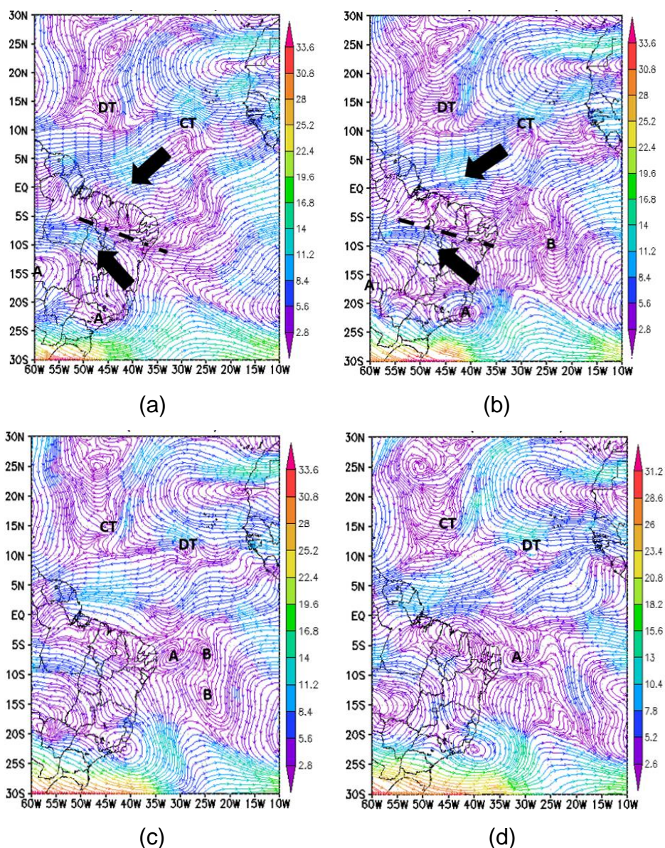
Figura 60 - Mapas de linhas de corrente e magnitude do vento ( m s^{-1} ), no nível de 500hPa, para o dia 16 de setembro de 2015 às 12Z (a) e 18Z (b), e o dia 17 às 00Z (c) e 06Z (d). Linha tracejada pontilhada (Convergência). Siglas: CT (Ciclone Tropical), DT (Distúrbio Tropical), B (Baixa Pressão) e A (Anticiclone).
