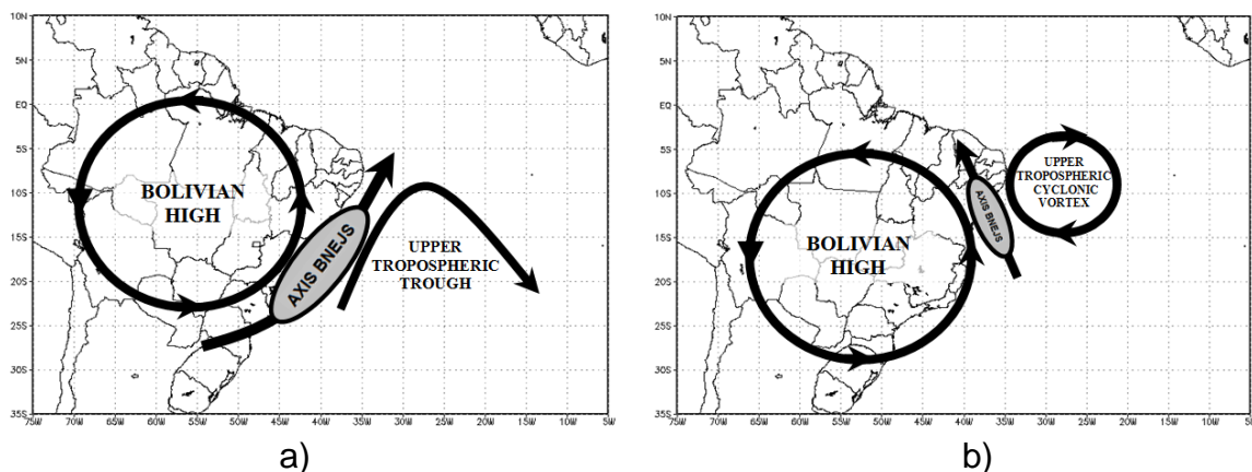
Figura 26 - Tipos de CJNEB: a, b - Tipo I, CJNEB de sul entre a alta da bolívia e o cavado (a) /VCAN (b) (a - jatos de sudoeste, b - jatos de sudeste e sul); c, d - Tipo II, CJNEB de norte entre a Alta subtropical e o cavado (c) / VCAN (d) (d - jatos de noroeste, c – jatos de norte); e - Tipo III, CJNEB de oeste entre VCAN no NH e o cavado no HS.
