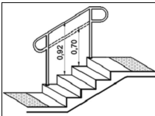
Figura 4.80 – Altura recomendada para o corrimão
