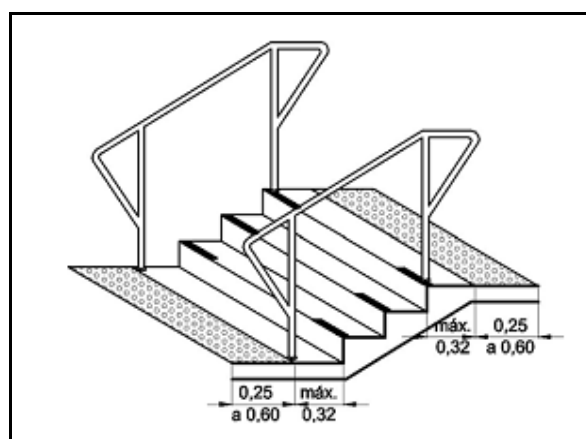
Figura 4.65 – Sinalização alerta segundo a norma
