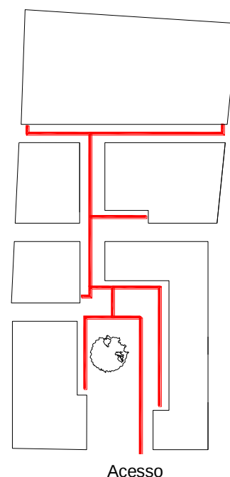
Figura 6.2 – Esquema da rota do piso tátil na escola Floriano Peixoto
