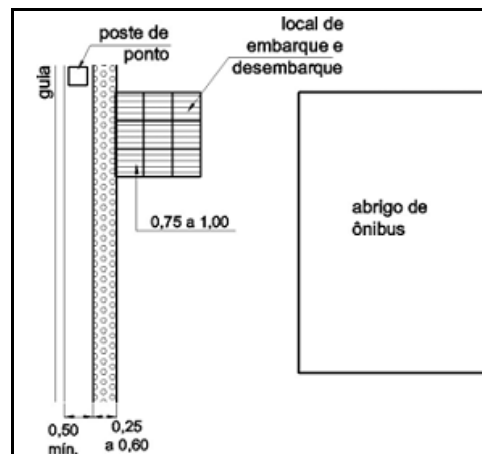
Figura 2.7 – Sinalização no ponto de ônibus
