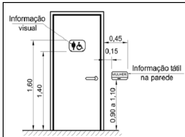
Figura 4.12 – Sinalização visual e tátil/NBR9050
