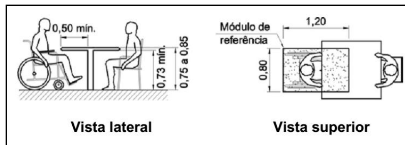
Figura 4.35 – Altura das mesas
