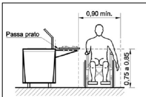
Figura 4.42 – Balcão de autoatendimento
