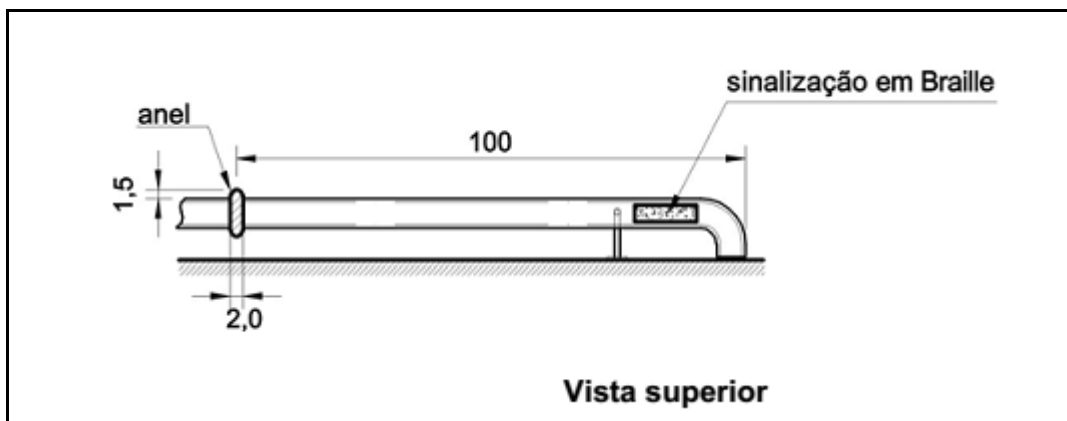
Figura 4.81 – Sinalização no corrimão
