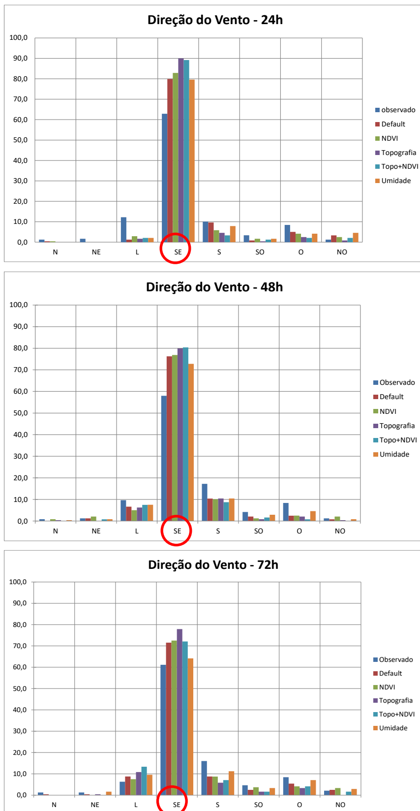
Figura 16 - Gráficos das simulações da Direção do Vento com dados observados e simulados para previsões de 24h/48h/72h.
