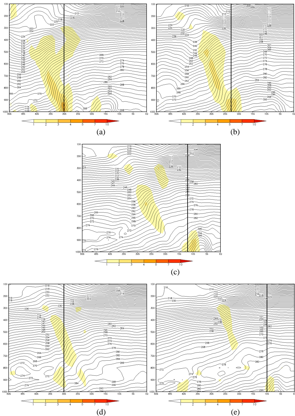
FIGURA 4.54 - Seção Vertical de Temperatura para os dias: a) 25/09/2012 às 00Z (lon 51°W) - POA; b) 26/09/2012 às 00Z (lon 46°W) - SP; c) 27/09/2012 às 12Z (lon 38°W) - SALV; d) 28/09/2012 às 00Z (lon 30°W) - regeneração e e) 29/09/2012 às 18Z (lon 36°W) - MCZ. FONTE: dados de reanálise do ECMWF.
