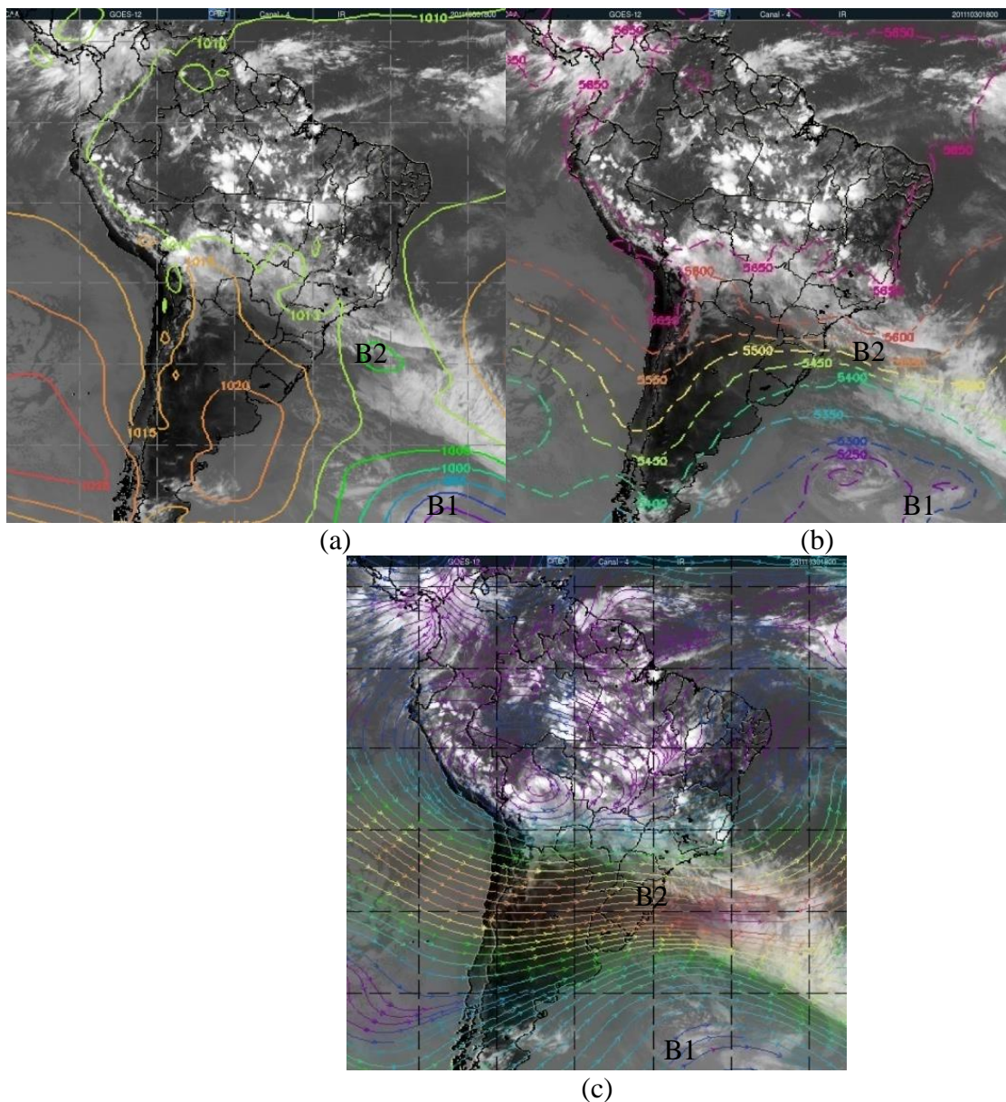
FIGURA 4.18 - Imagem de satélite do canal infravermelho para o dia 30/10/2011 18Z sobreposta com: (a) campo de PNM (b) campo de espessura da camada 500/1000hPa (c) campo de linha de corrente em 200hPa. FONTE: Adaptada de CPTEC/INPE e ECMWF
