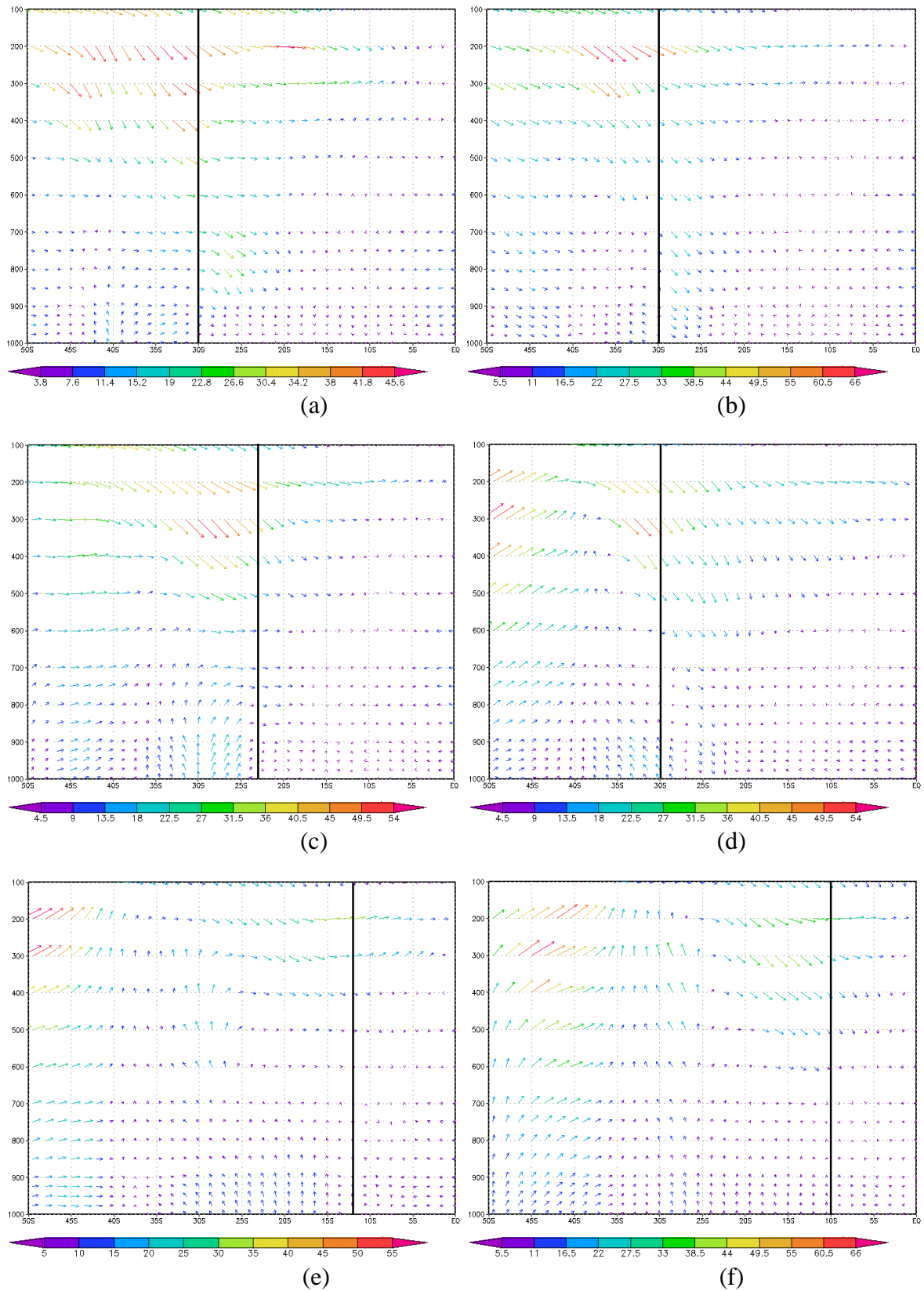
FIGURA 4.21 - Seção Vertical de Linha de Corrente para os dias: a) 19/05/2002 às 06Z (lon 51°W) - POA; b) 21/05/2002 às 06Z (lon 47°W) - ciclogênese; c) 21/05/2002 às 12Z (lon 46°W) - SP; d) 23/05/2002 às 12Z (lon 30°W) - regeneração; e) 24/05/2002 às 00Z (lon 38°W) - SALV e f) 26/05/2002 às 00Z (lon 36°W) - MCZ. FONTE: dados de reanálise do ECMWF.
