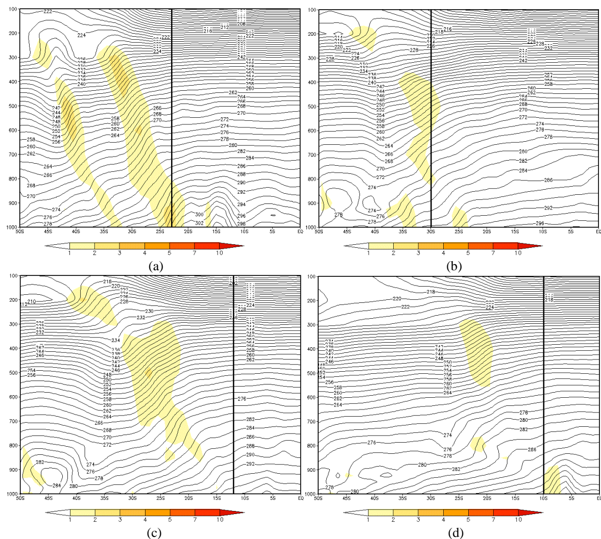
FIGURA 4.71 - Seções Verticais de Temperatura para os dias: a) 30/10/2011 às 18Z (lon 46°W) - SP; b) 01/11/2011 às 12Z (lon 30°W) - regeneração; c) 02/11/2011 às 00Z (lon 38°W) - SALV e d) 04/11/2011 às 18Z (lon 36°W) - MCZ. FONTE: dados de reanálise do ECMWF
