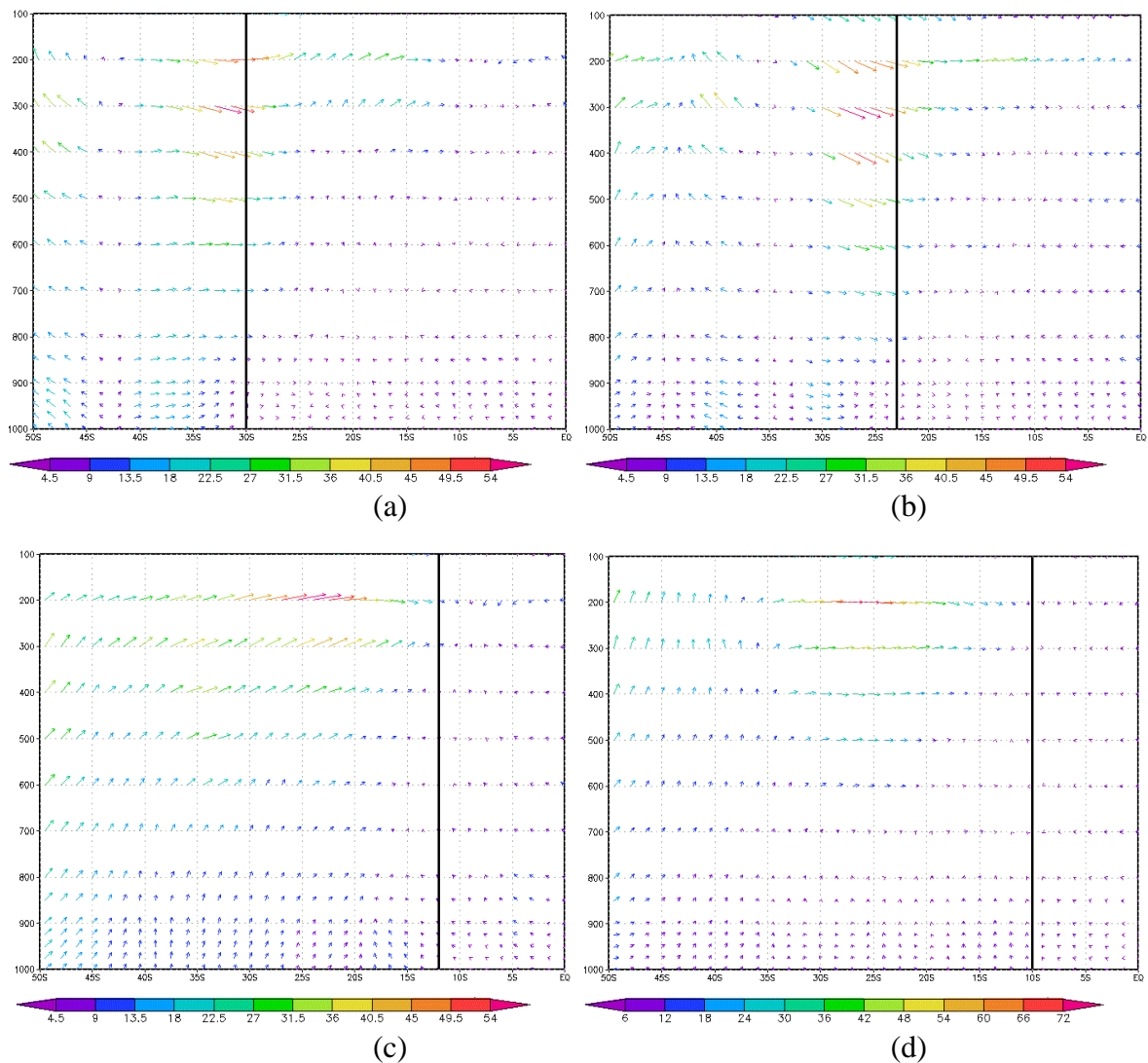
FIGURA 4.32 - Seção Vertical de Vento para os dias: a) 30/04/2006 às 12Z (lon 51°W) - POA; b) 02/05/2006 às 18Z (lon 46°W) - SP; c) 06/5/2006 às 00Z (lon 38°W) - SALV e d) 07/05/2006 às 18Z (lon 36°W) - MCZ. FONTE: Dados de Reanálises do ECMWF.
