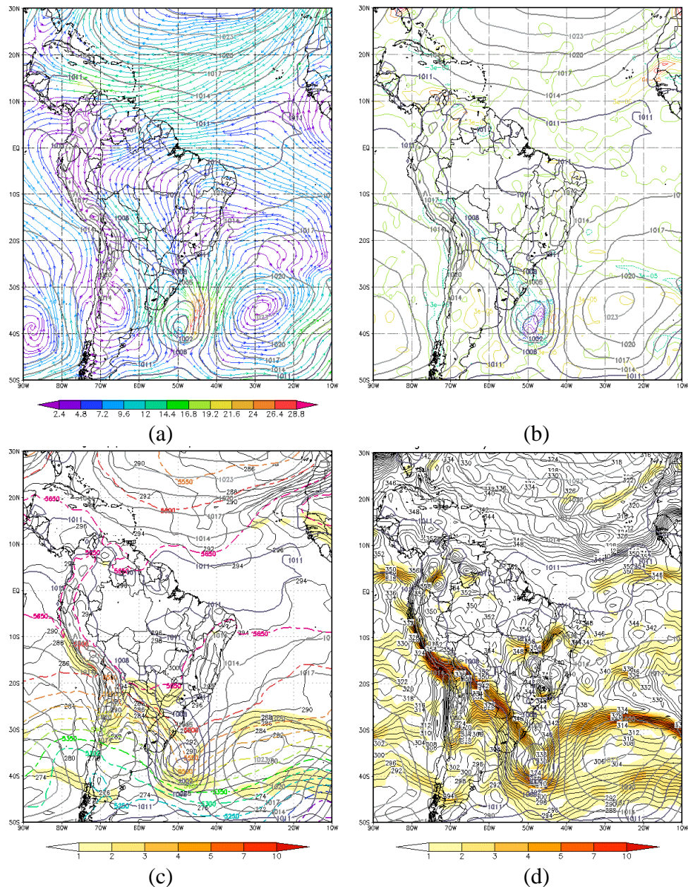
FIGURA 4.1 - Campos meteorológicos em baixos níveis sobrepostos no campo de PNM no dia 19/05/2002 às 06Z: (a) Vento em 925hPa (em cores); (b) Vorticidade Relativa em 925hPa (em cores); (c) Temperatura e Espessura 500/1000hPa (pontilhada) e (d) Temperatura Potencial Equivalente. FONTE: dados de reanálise do ECMWF
