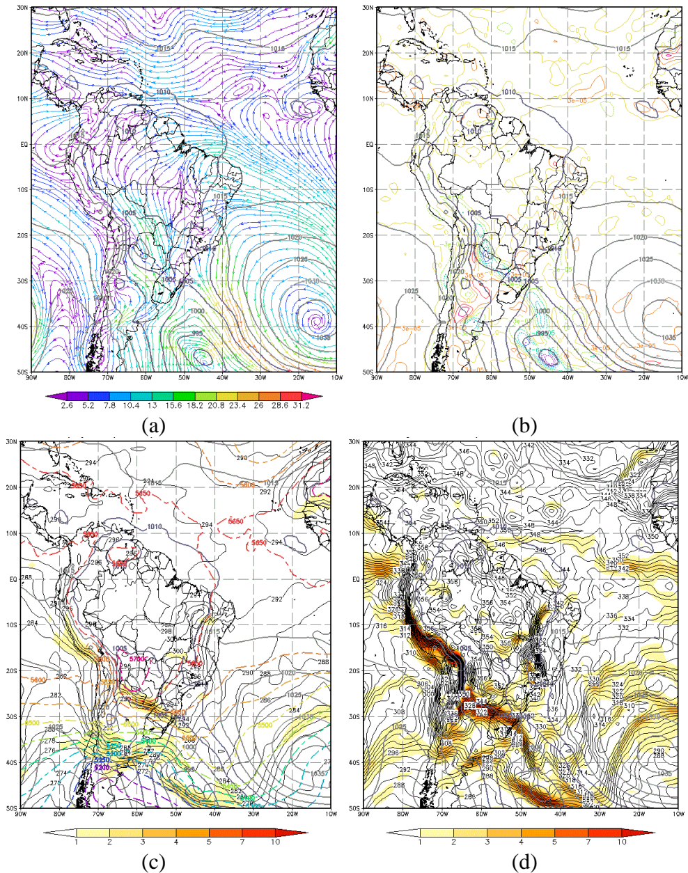
FIGURA 4.7- Campos meteorológicos em baixos níveis sobrepostos no campo de PNM no dia 09/10/2003 às 06Z: (a) Vento em 925hPa (em cores); (b) Vorticidade Relativa em 925hPa (em cores); (c) Temperatura e Espessura 500/1000hPa (pontilhada) e (d) Temperatura Potencial Equivalente. FONTE: dados de reanálise do ECMWF
