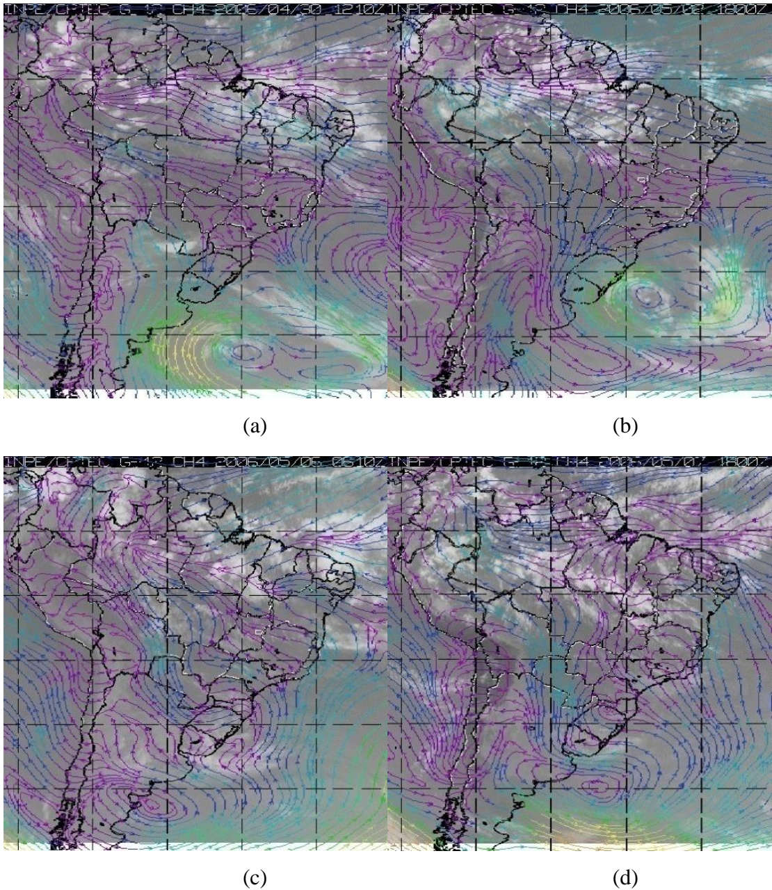
FIGURA 4.31 - Imagens de satélite do canal infravermelho sobreposta com linhas de correntes em 925hPa para os dias: a) 30/04/2006 às 12Z; b) 02/05/2006 às 18Z; c) 06/05/2006 às 00Z e d) 07/05/2006 às 18Z. FONTE: Adaptada de CPTEC/INPE e ECMWF
