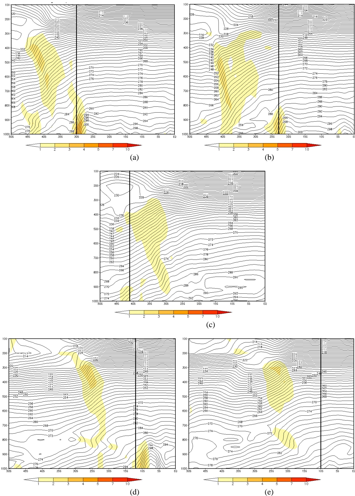
FIGURA 4.47 - Seção Vertical de Temperatura para os dias: a) 15/10/2006 às 18Z (lon 51°W) - POA; b) 17/10/2006 às 18Z (lon 46°W) - SP; c) 20/10/2006 às 06Z (lon 21°W) - regeneração; d) 21/10/2006 às 18Z (lon 38°W) - SALV e d) 23/10/2006 às 00Z (lon 36°W) - MCZ. FONTE: dados de reanálise do ECMWF
