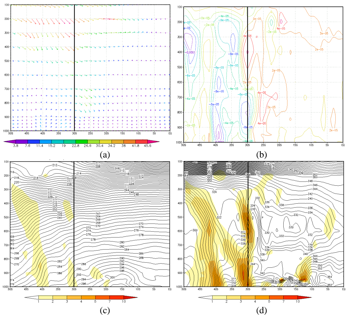
FIGURA 4.3 - Seção Vertical sobre a longitude de Porto Alegre 51^{\circ}\text{W} no dia 19/05/2002 às 06Z de: (a) vento; (b) vorticidade relativa; (c) temperatura e (d) temperatura potencial equivalente. FONTE: de dados de reanálise do ECMWF
