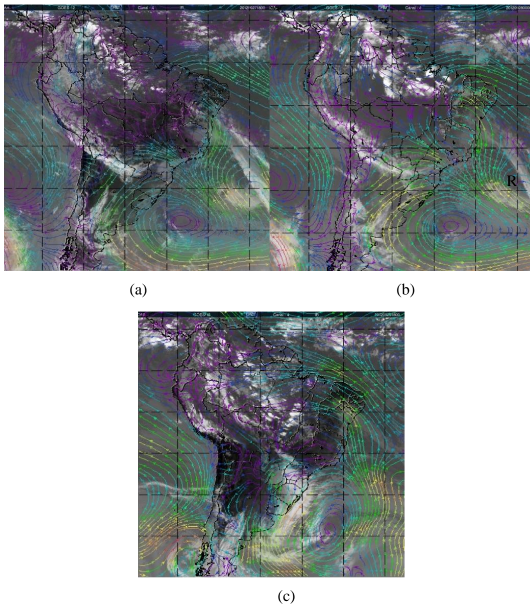
FIGURA 4.51 - Imagem de satélite do canal infravermelho sobreposta com linhas de correntes em 925hPa para os dias: a) 27/09/2012 às 12Z e b) 29/09/2012 às 18Z. FONTE: Adaptada de CPTEC/INPE e ECMWF
