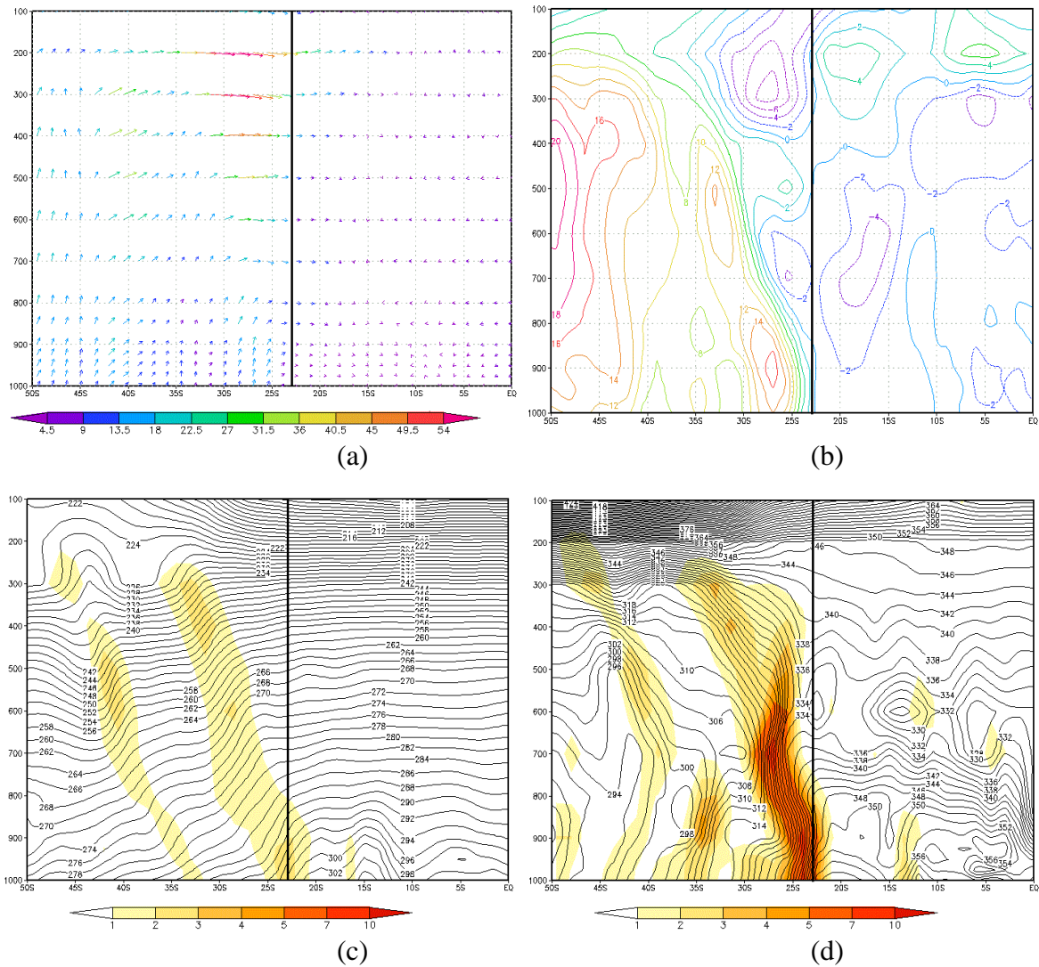
FIGURA 4.19 - Seção Vertical sobre a longitude de São Paulo 46°W no dia 30/10/2011 às 18Z de: (a) vento; (b) vorticidade relativa; (c) temperatura e (d) temperatura potencial equivalente. FONTE: de dados de reanálise do ECMWF.
