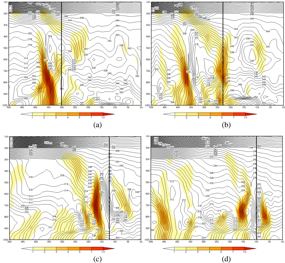
FIGURA 4.26 - Seção Vertical de Temperatura Potencial Equivalente para os dias: a) 19/04/2000 às 06Z (lon 51°W) - POA; b) 20/04/2000 às 06Z (lon 46°W) - SP; c) 23/04/2000 às 12Z (lon 38°W) - SALV e d) 24/04/2000 às 12Z (lon 36°W) - MCZ. FONTE: dados de reanálise do ECMWF.
