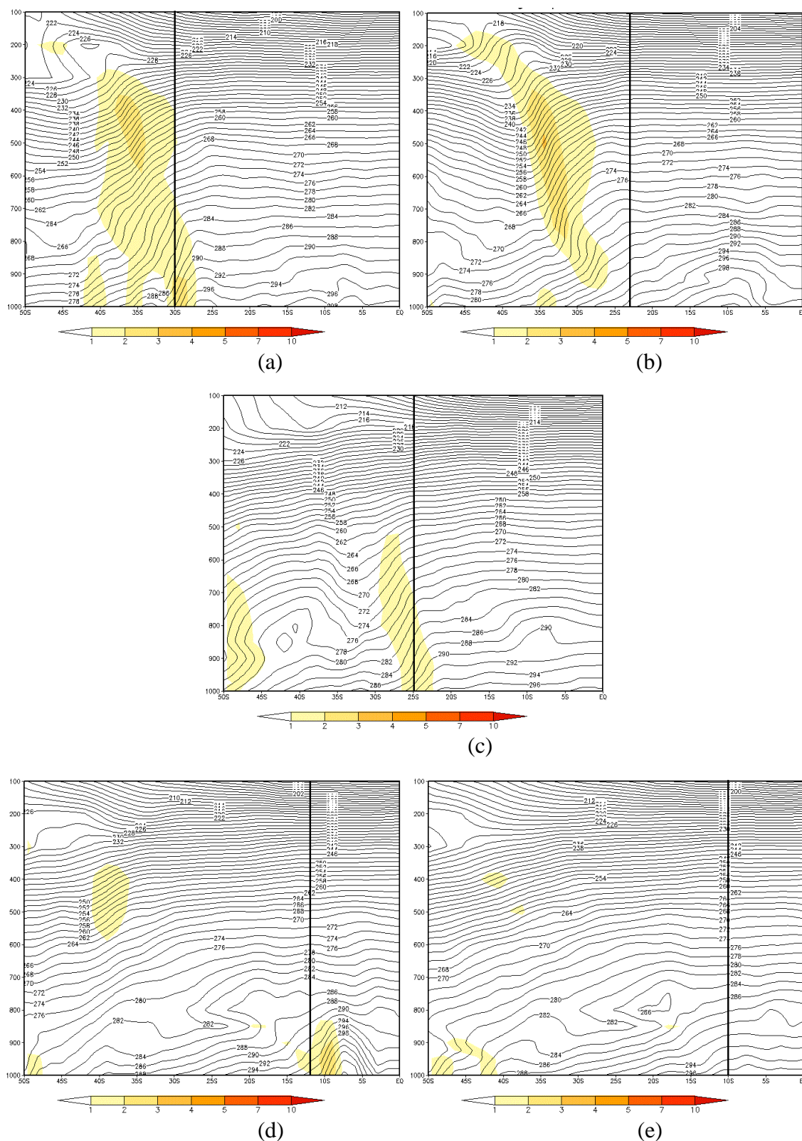
FIGURA 4.58 - Seção Vertical de Temperatura para os dias: a) 01/12/2005 às 12Z (lon 51°W) - POA; b) 02/12/2005 às 0Z (lon 46°W) - SP; c) 04/12/2005 às 00Z (lon 21°W) - regeneração; d) 04/12/2005 às 18Z (lon 38°W) - SALV e e) 05/12/2005 às 00Z (lon 36°W) - MCZ. FONTE: dados de reanálise do ECMWF.
