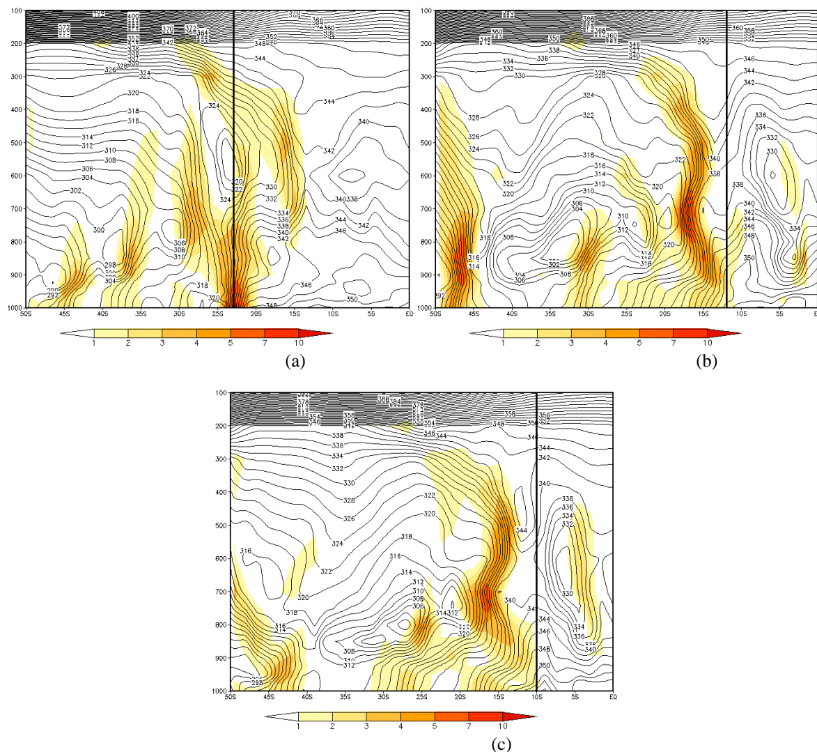
FIGURA 4.74 - Seções Verticais de Temperatura Potencial Equivalente para os dias: a) 30/04/2005 às 12Z (lon 46°W) - SP; b) 02/05/2005 às 06Z (lon 38°W) - SALV; c) 03/05/2005 às 00Z (lon 36°W) - MCZ. FONTE: dados de reanálise do ECMWF.
