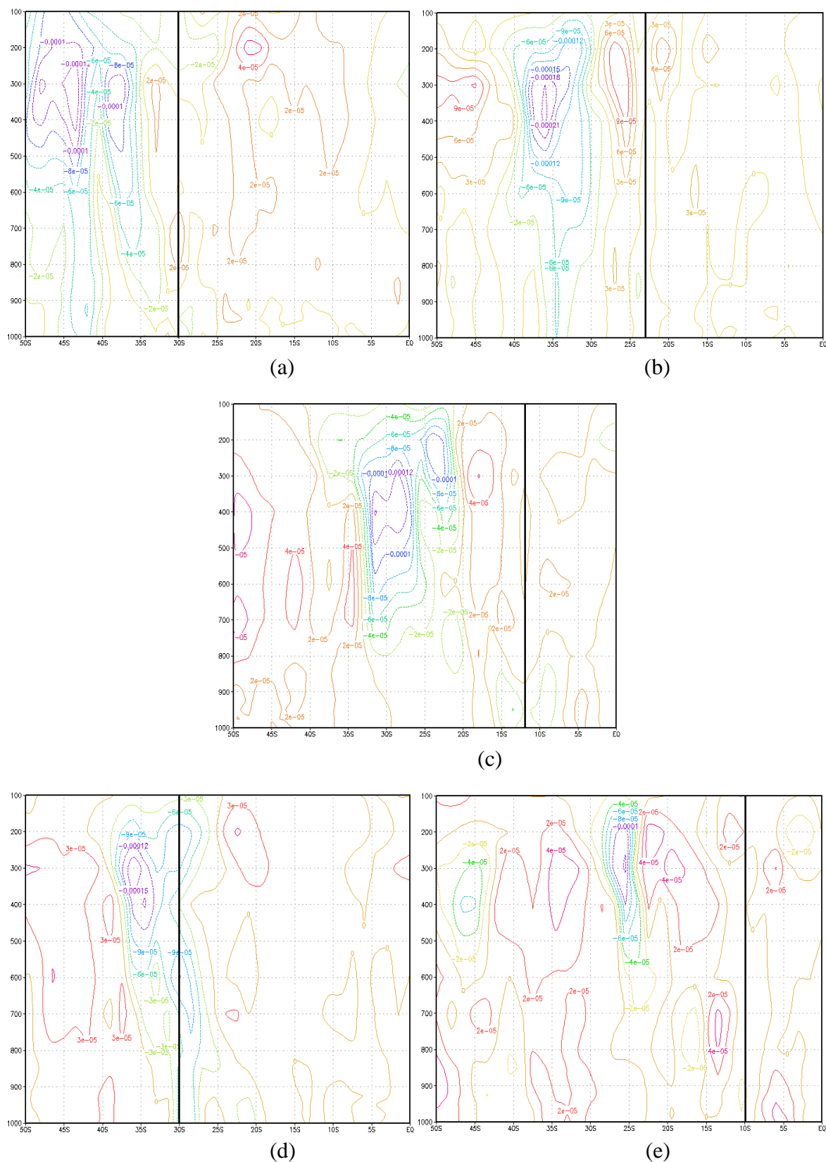
FIGURA 4.53 - Seção Vertical de Vorticidade Relativa para os dias: a) 25/09/2012 às 00Z (lon 51°W) - POA; b) 26/09/2012 às 00Z (lon 46°W) - SP; c) 27/09/2012 às 12Z (lon 38°W) - SALV; d) 28/09/2012 às 00Z (lon 30°W) - regeneração e e) 29/09/2012 às 18Z (lon 36°W) - MCZ. FONTE: dados de reanálise do ECMWF.
