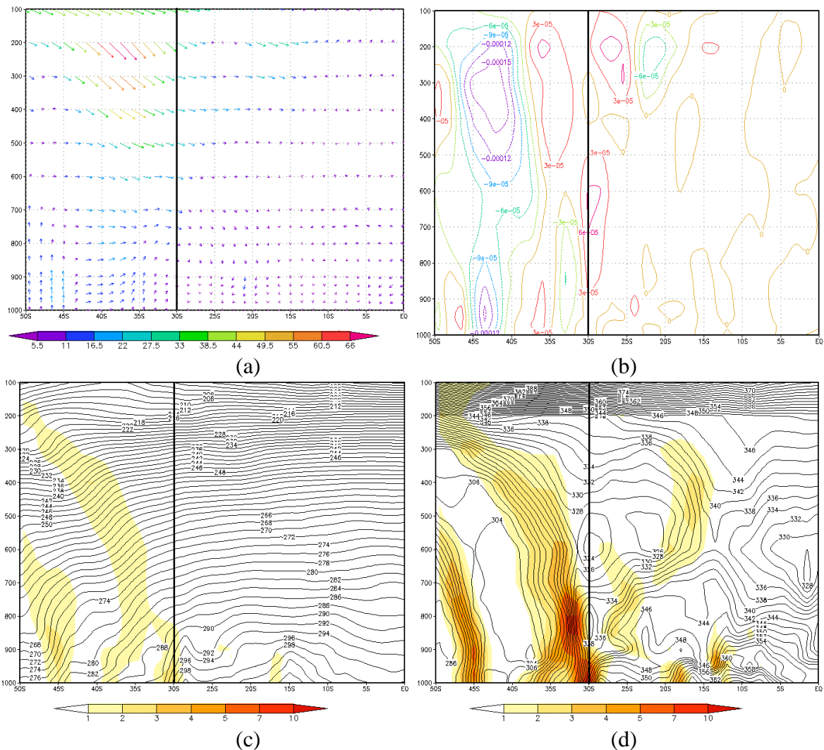
FIGURA 4.9 – Seção Vertical sobre a longitude de Porto Alegre 51°W no dia 09/10/2003 às 06Z de: (a) vento; (b) vorticidade relativa; (c) temperatura e (d) temperatura potencial equivalente. FONTE: de dados de reanálise do ECMWF.
