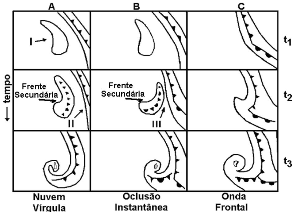
FIGURA 2.7 - Descrição esquemática das três sequências básicas de desenvolvimento de vórtices através de imagens de satélite: a) desenvolvimento de nuvem vírgula inteiramente dentro do ar frio; b) desenvolvimento de uma oclusão instantânea; c) desenvolvimento de uma onda frontal. Os algarismos romanos I, II e III indica respectivamente uma região de forte convecção, uma banda de nuvens em decaimento e uma banda de nuvens convectiva mergindo com uma banda de nuvens frontal. FONTE: adaptada de BROWNING (1986), citada por BONATTI (1988).
