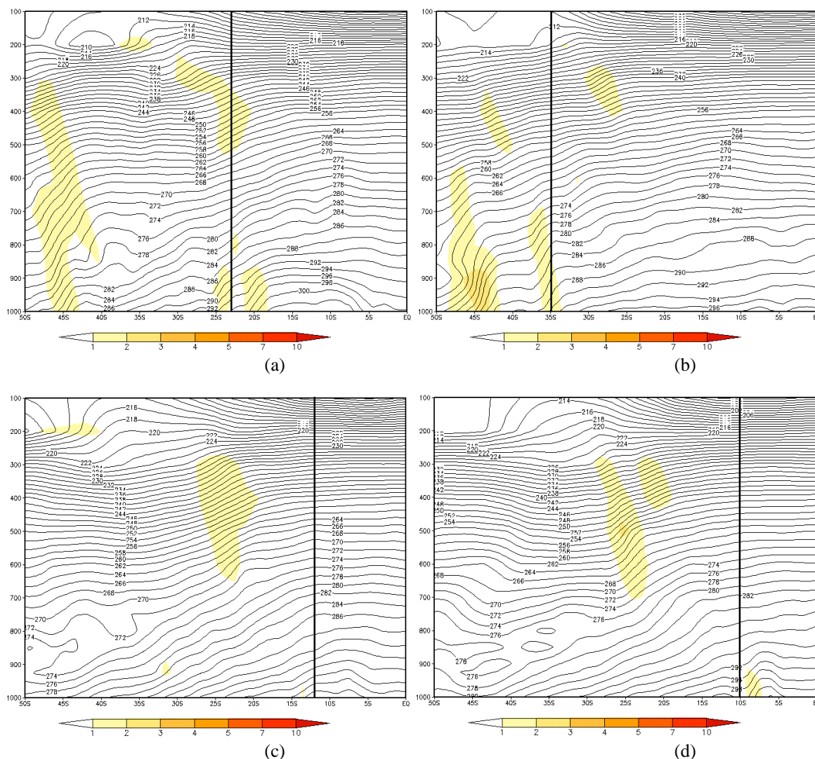
FIGURA 4.75 - Seções Verticais de Temperatura para os dias: a) 10/05/2006 às 18Z (lon 46°W) - SP; b) 13/05/2006 às 06Z (lon 25°W) - regeneração; c) 13/05/2006 às 18Z (lon 38°W) - SALV e d) 15/05/2006 às 18Z (lon 36°W) - MCZ. FONTE: dados de reanálise do ECMWF.
