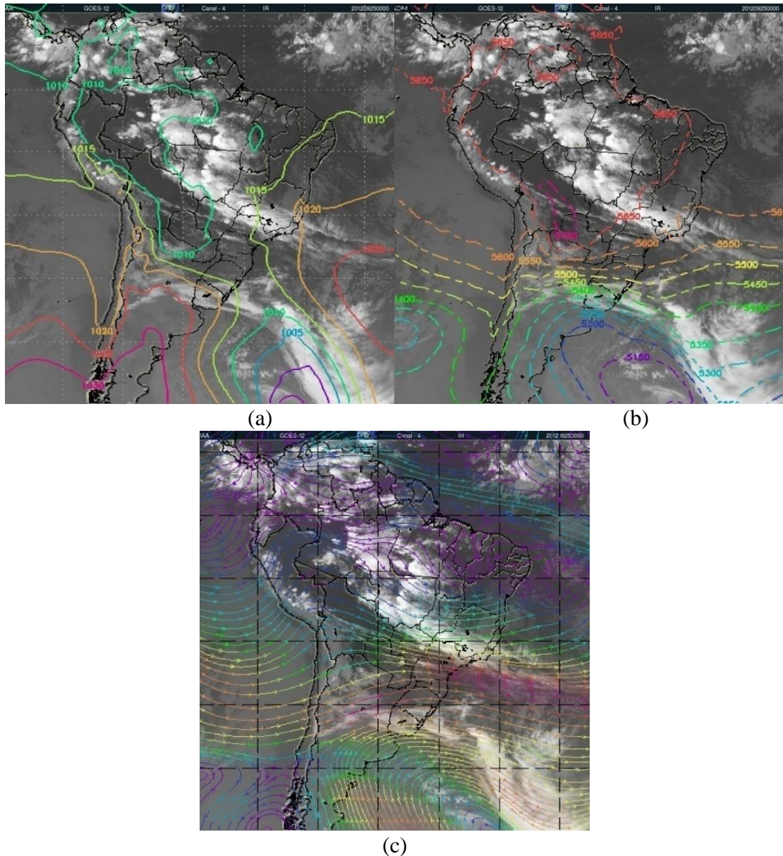
FIGURA 4.11 - Imagem de satélite do canal infravermelho para o dia 25/09/2012 00Z sobreposta com: (a) campo de PNM (b) campo de espessura da camada 500/1000hPa (c) campo de linha de corrente em 200hPa. FONTE: Adaptada de CPTEC/INPE e ECMWF
