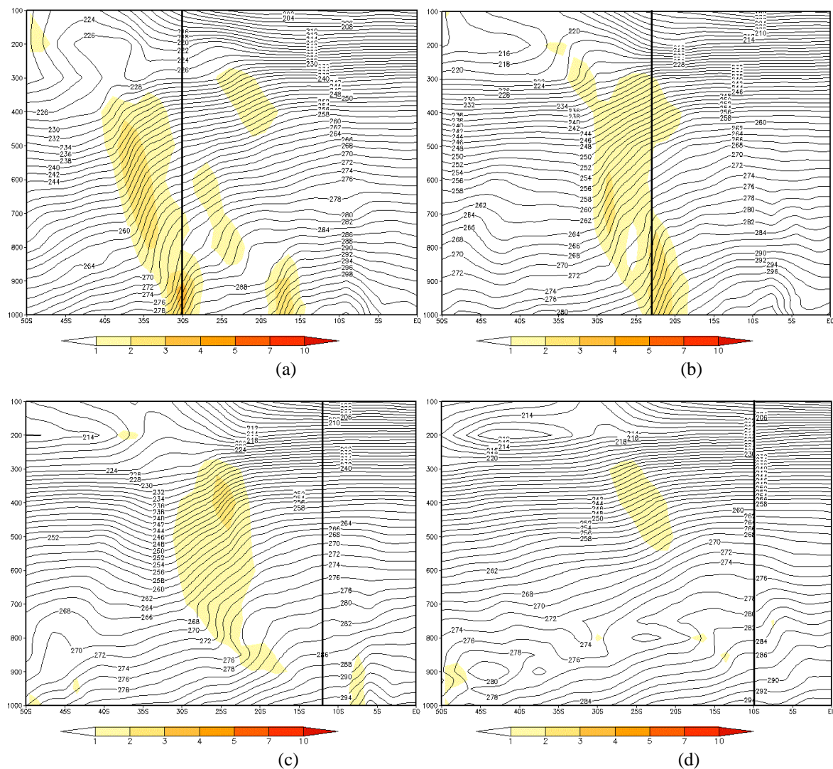
FIGURA 4.63 - Seção Vertical de Temperatura para os dias: a) 27/07/2007 às 18Z (lon 51°W) - POA; b) 29/07/2007 às 00Z (lon 46°W) - SP; c) 30/07/2007 às 00Z (lon 38°W) - SALV e d) 31/07/2007 às 12Z (lon 36°W) - MCZ. FONTE: dados de reanálise do ECMWF.
