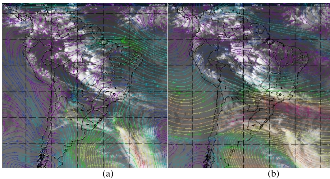
FIGURA 4.49 - Imagem de satélite do canal infravermelho sobreposta com linhas de correntes para o dia 25/09/2012 às 00Z em: a) 925hPa e b) 200hPa. FONTE: Adaptada de CPTEC/INPE e ECMWF
