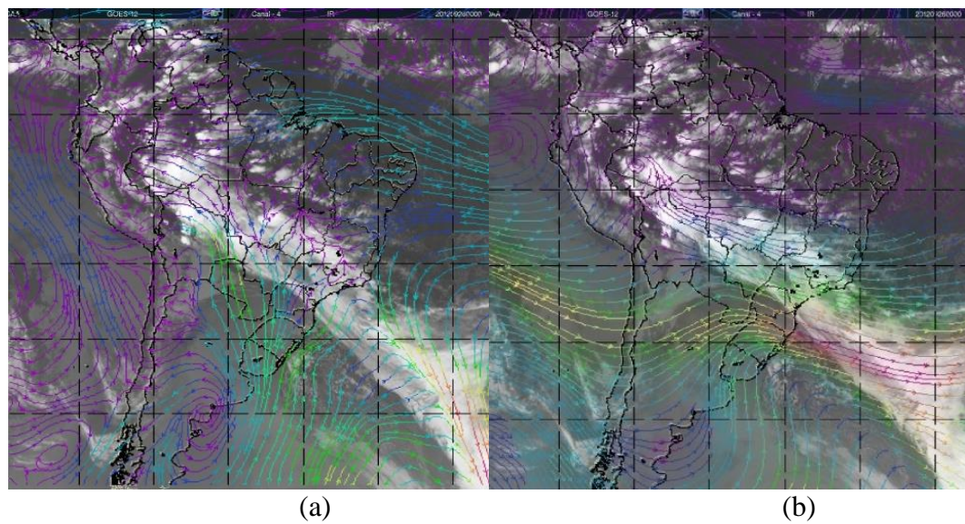
FIGURA 4.50 - Imagem de satélite do canal infravermelho sobreposta com linhas de correntes para o dia 26/09/2012 às 00Z em: a) 925hPa e b) 200hPa. FONTE: Adaptada de CPTEC/INPE e ECMWF
