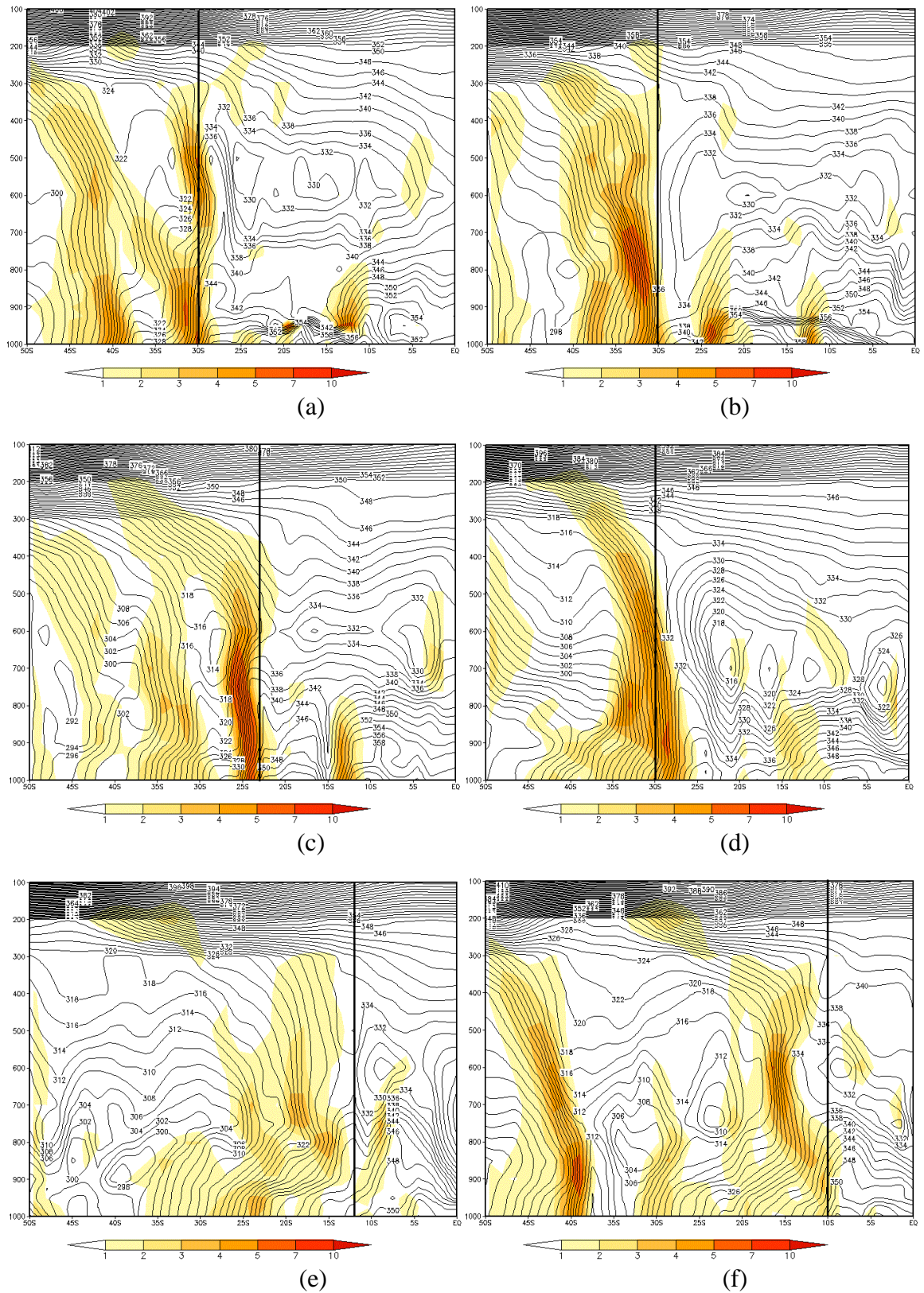
FIGURA 4.24 - Seção Vertical de Temperatura Potencial Equivalente para os dias: a) 19/05/2002 às 06Z (lon 51°W) - POA; b) 21/05/2002 às 06Z (lon 47°W) - ciclogênese; c) 21/05/2002 às 12Z (lon 46°W) - SP; d) 23/05/2002 às 12Z (lon 30°W) - regeneração; e) 24/05/2002 às 00Z (lon 38°W) - SALV e f) 26/05/2002 às 00Z (lon 36°W) - MCZ. FONTE: dados de reanálise do ECMWF.
