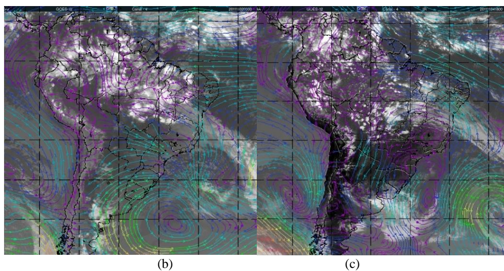
FIGURA 4.68 - Imagens de satélites do campo infravermelho sobrepostos com linhas de correntes em 925hPa para os dias: a) 01/11/2011 às 12Z; b) 02/11/2011 às 00Z e c) 04/11/2011 às 18Z. FONTE: Adaptada de CPTEC/INPE e ECMWF
