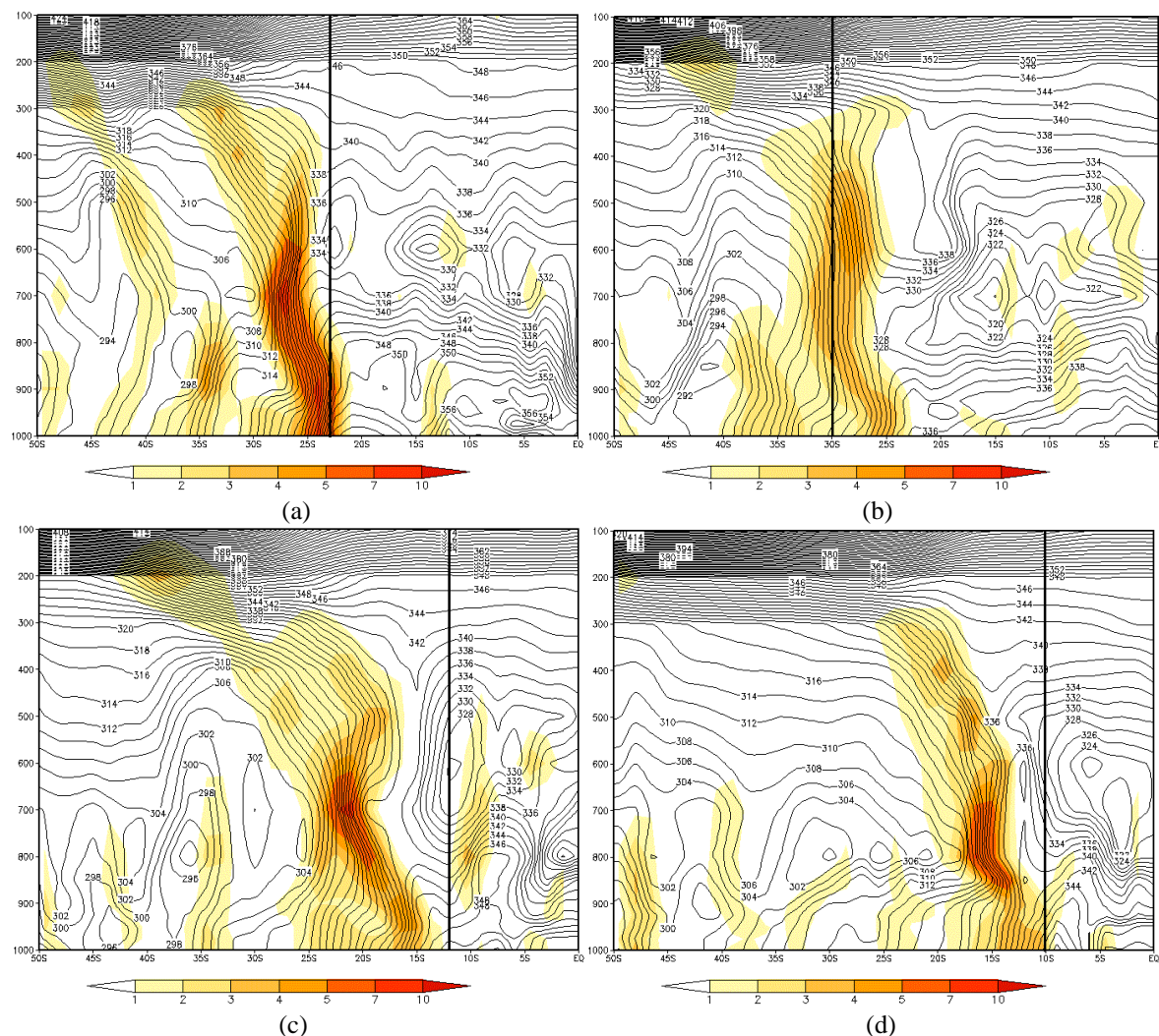
FIGURA 4.72 - Seções Verticais de Temperatura Potencial Equivalente para os dias: a) 30/10/2011 às 18Z (lon 46°W) - SP; b) 01/11/2011 às 12Z (lon 30°W) - regeneração; c) 02/11/2011 às 00Z (lon 38°W) - SALV e d) 04/11/2011 às 18Z (lon 36°W) - MCZ. FONTE: dados de reanálise do ECMWF
