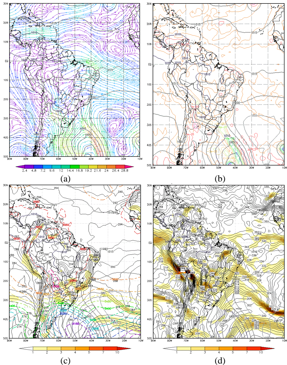
FIGURA 4.10 - Campos meteorológicos em baixos níveis sobrepostos no campo de PNM no dia 25/09/2012 às 00Z: (a) Vento em 925hPa (em cores); (b) Vorticidade Relativa em 925hPa (em cores); (c) Temperatura e Espessura 500/1000hPa (pontilhada) e (d) Temperatura Potencial Equivalente. FONTE: dados de reanálise do ECMWF.
