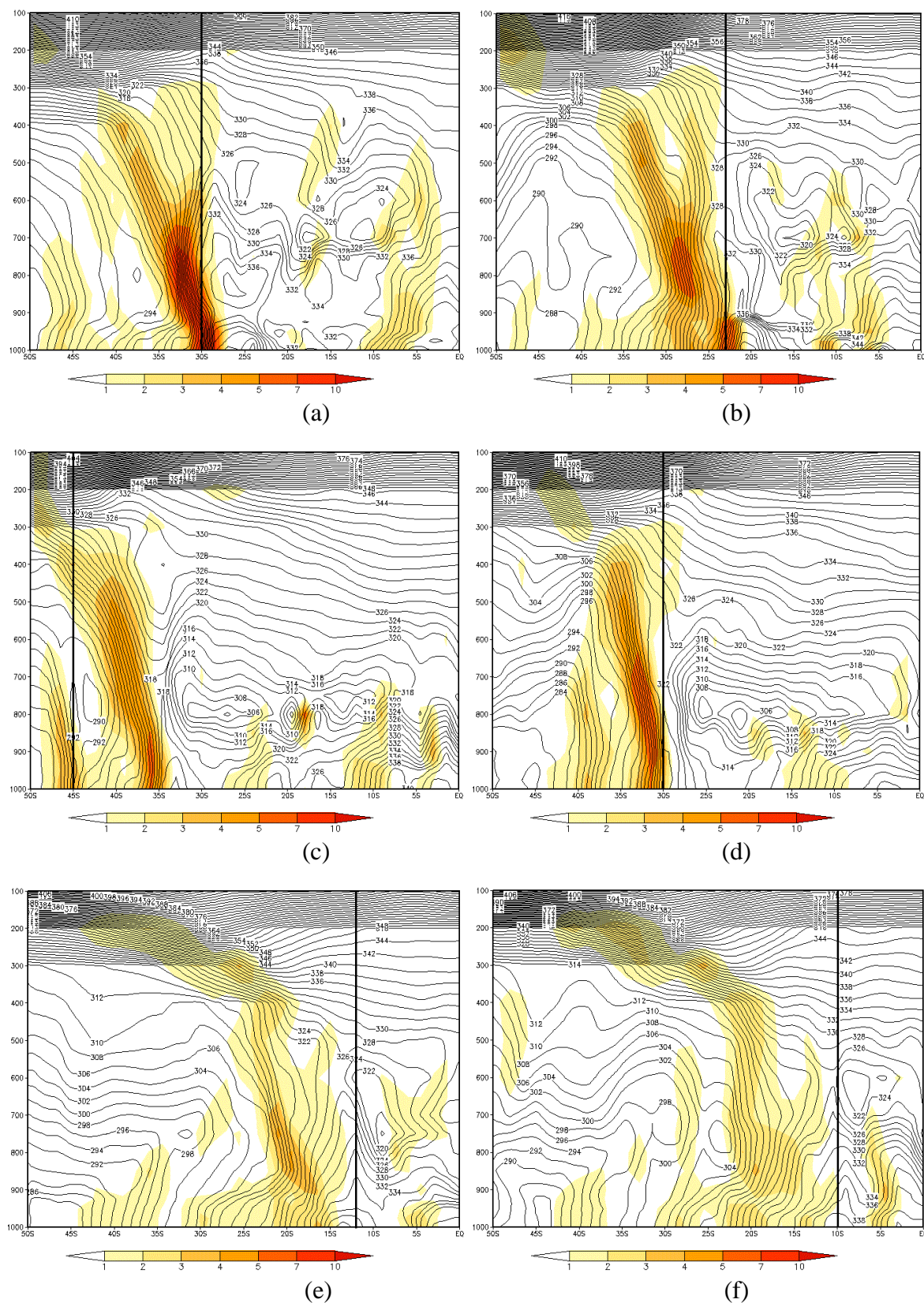
FIGURA 4.46 - Seção Vertical de Temperatura Potencial Equivalente para os dias: a) 15/07/2004 às 12Z (lon 51°W) - POA; b) 17/07/2004 às 06Z (lon 46°W) - SP; c) 17/07/2007 às 12Z (lon 25°W) - regeneração; d) 20/07/2007 às 06Z (lon 12°W) - regeneração; e) 21/07/2004 às 12Z (lon 38°W) - SALV e d) 22/07/2004 às 06Z (lon 36°W) - MCZ. FONTE: dados de reanálise do ECMWF
