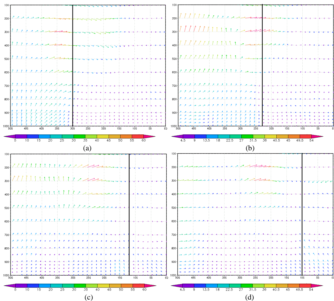
FIGURA 4.61 - Seção Vertical de Linhas de Correntes para os dias: a) 27/07/2007 às 18Z (lon 51°W) - POA; b) 29/07/2007 às 00Z (lon 46°W) - SP; c) 30/07/2007 às 00Z (lon 38°W) - SALV e d) 31/07/2007 às 12Z (lon 36°W) - MCZ. FONTE: dados de reanálise do ECMWF.
