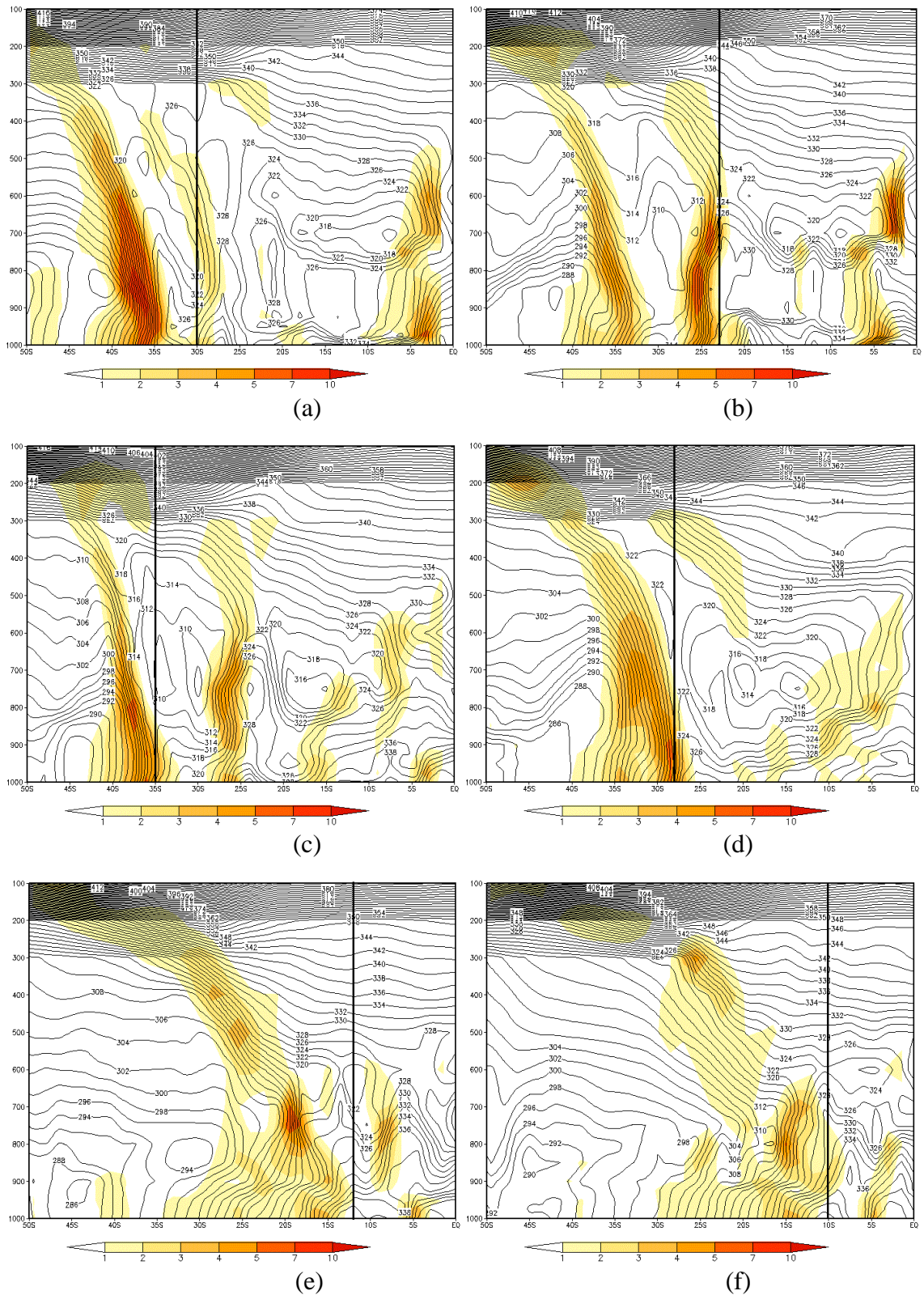
FIGURA 4.30 - Seção Vertical de Temperatura Potencial Equivalente para os dias: a) 13/08/2010 às 06Z (lon 51°W) - POA; b) 14/08/2010 às 00Z (lon 46°W) - SP; c) 14/08/2010 às 06Z (lon 40°W) - regeneração; d) 17/08/2010 às 00Z (lon 22°W) - regeneração; e) 17/08/2010 às 00Z (lon 38°W) - SALV e f) 17/08/2010 às 18Z (lon 36°W) - MCZ. FONTE: dados de reanálise do ECMWF.
