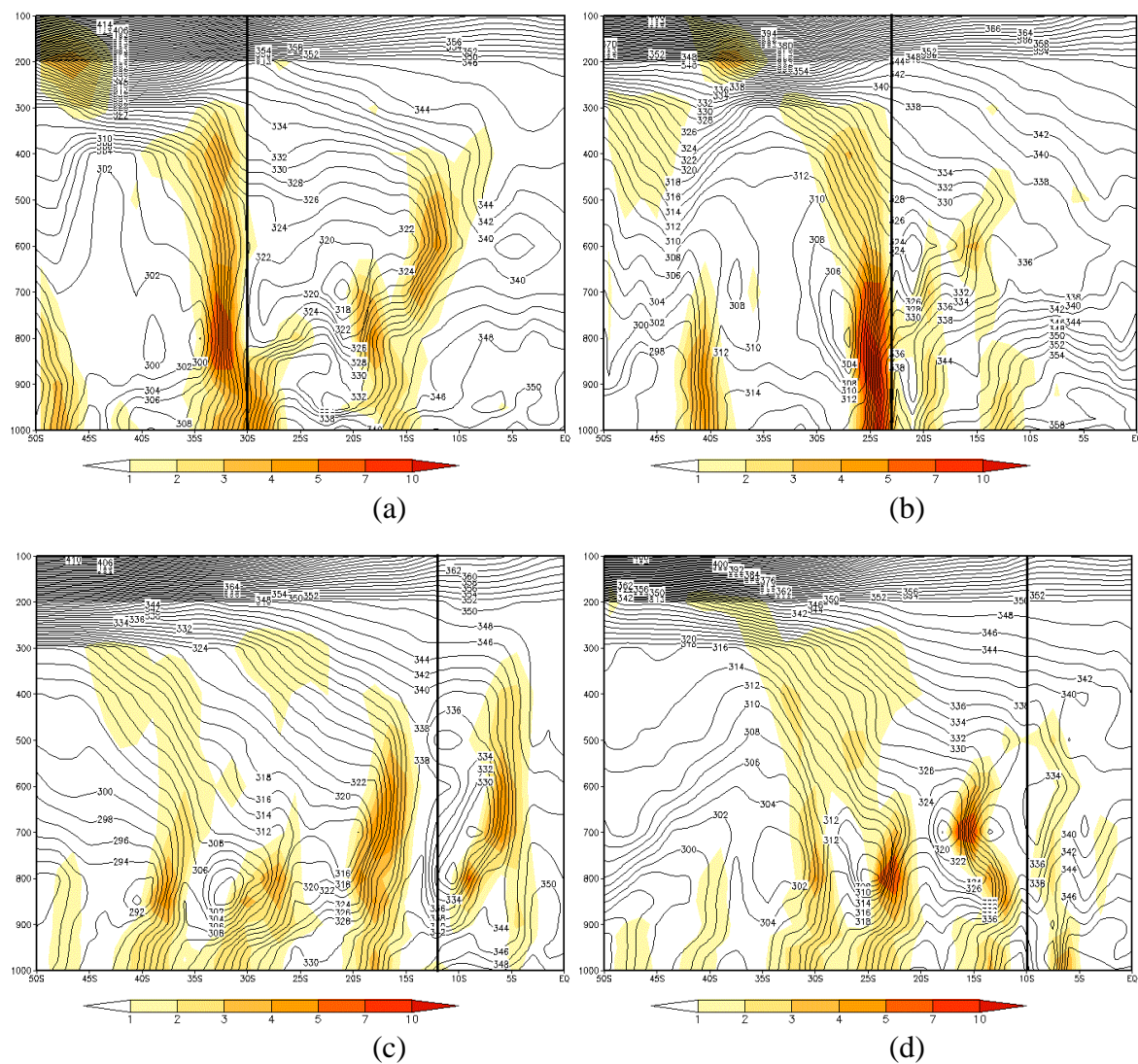
FIGURA 4.35 - Seção Vertical de Temperatura Potencial Equivalente para os dias: a) 30/04/2006 às 12Z (lon 51^\circ\text{W} ) - POA; b) 02/05/2006 às 18Z (lon 46^\circ\text{W} ) - SP; c) 06/05/2006 às 00Z (lon 38^\circ\text{W} ) - SALV e d) 07/05/2006 às 18Z (lon 36^\circ\text{W} ) - MCZ. FONTE: Dados de Reanálises do ECMWF.
