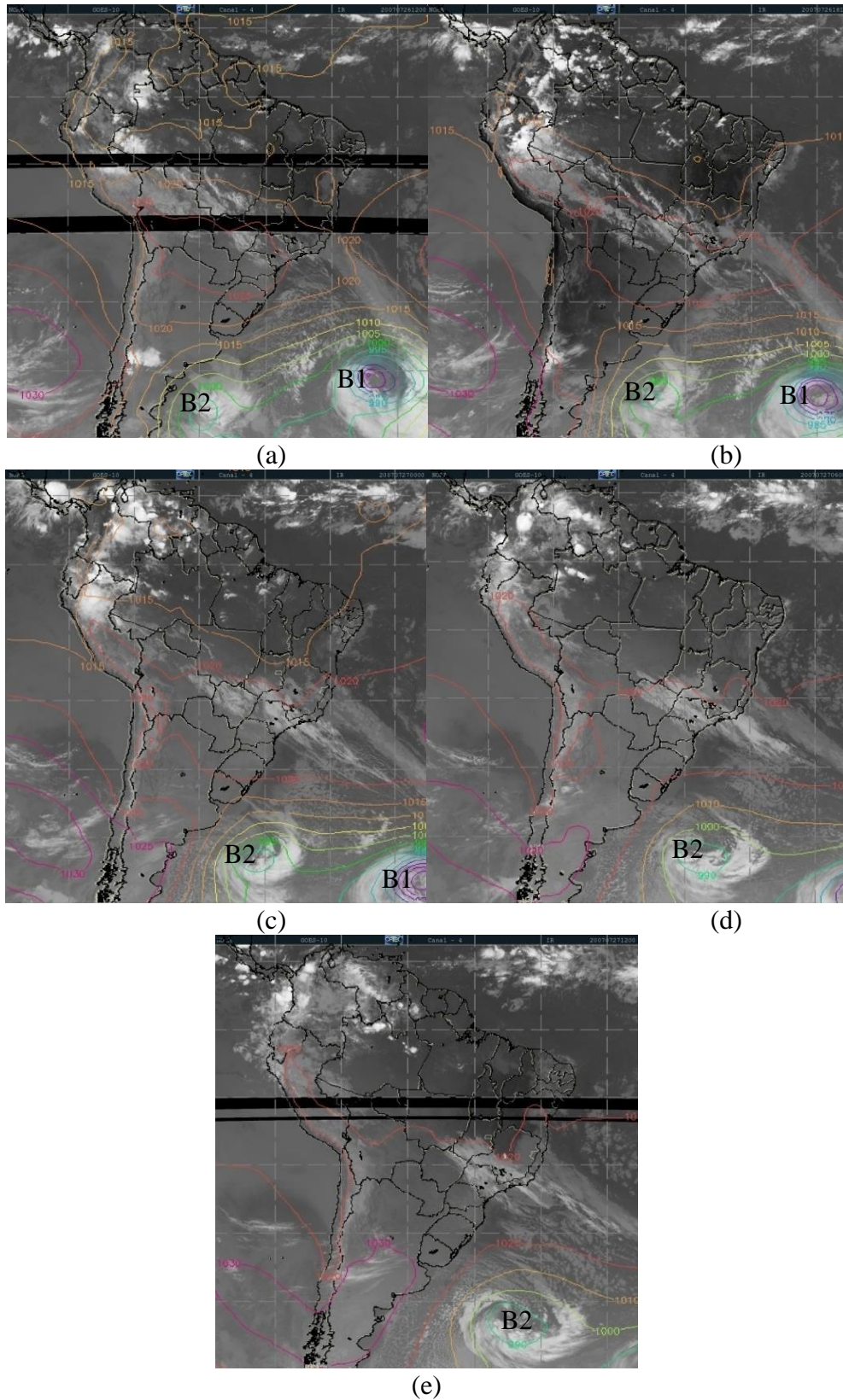
FIGURA 4.13 - Imagens do satélite GOES-10 do canal infravermelho entre os dias 26/07/2007 e 27/07/2007: (a) 26/07/2007 às 12Z; (b) 26/07/2007 às 18Z; (c) 27/07/2007 às 00Z; (d) 27/07/2007 às 06Z e (e) 27/07/2007 às 12Z. FONTE: Adaptada de CPTEC/INPE e ECMWF
