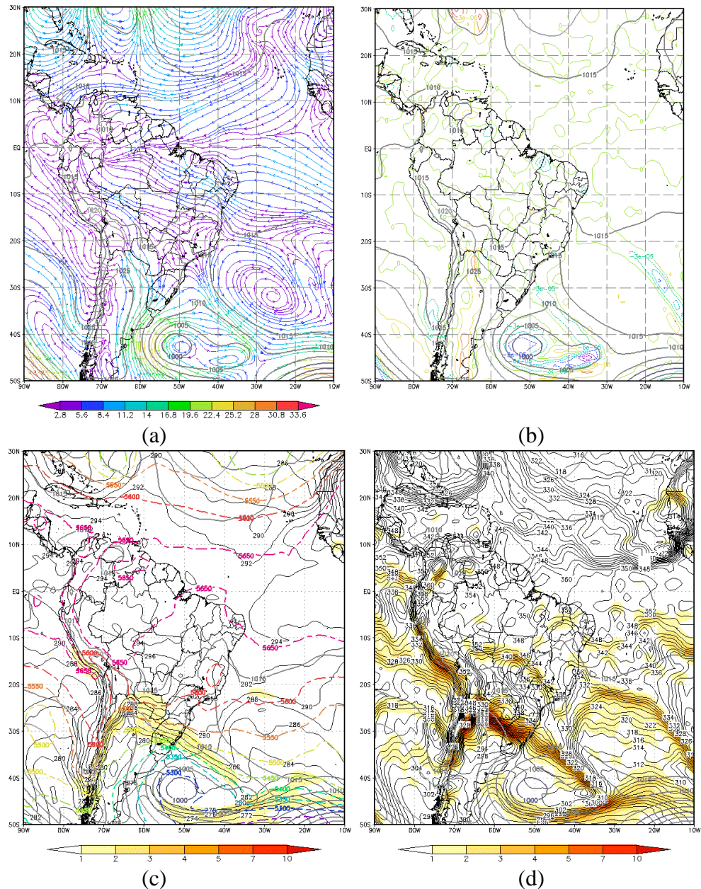
FIGURA 4.4 - Campos meteorológicos em baixos níveis sobrepostos no campo de PNM no dia 30/04/2006 às 12z: (a) Vento em 925hPa (em cores); (b) Vorticidade Relativa em 925hPa (em cores); (c) Temperatura e Espessura 500/1000hPa (pontilhada) e (d) Temperatura Potencial Equivalente. FONTE: dados de reanálise do ECMWF
