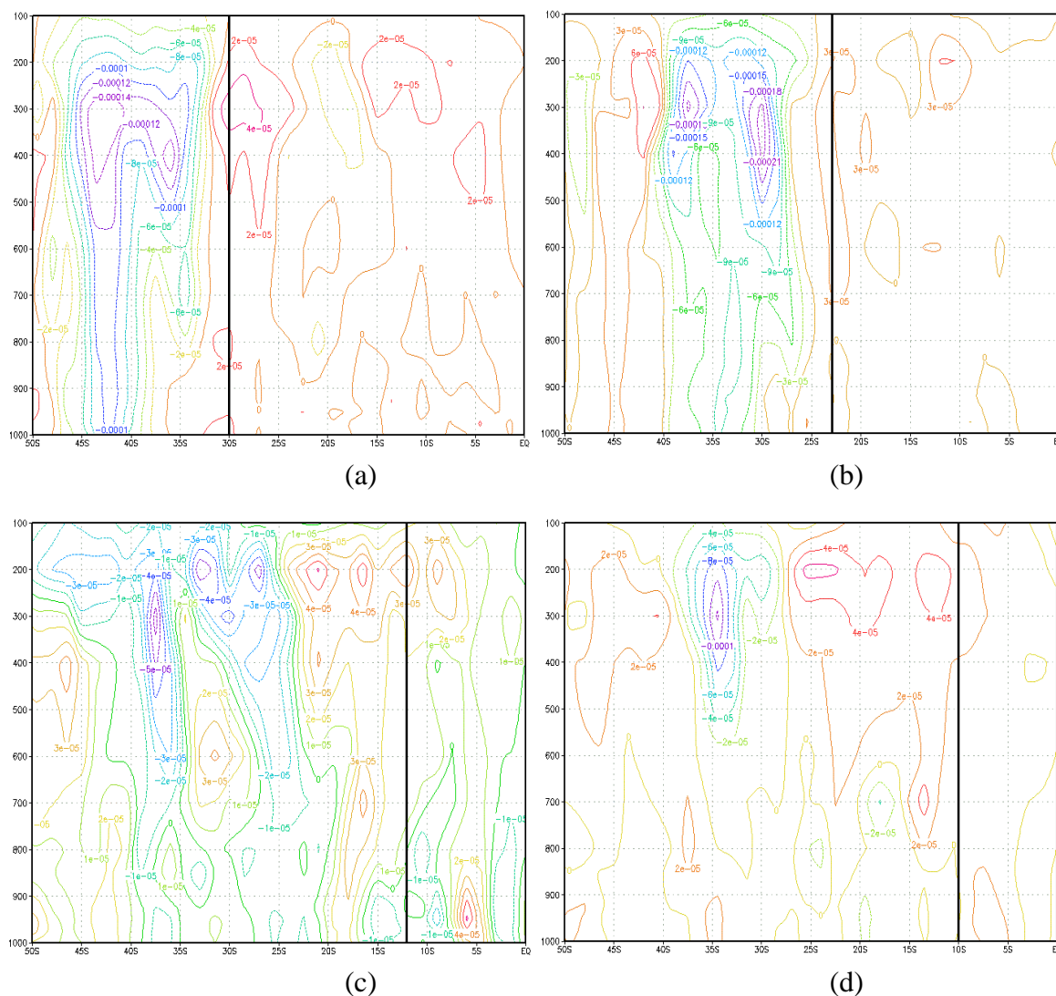
FIGURA 4.33 - Seção Vertical de Vorticidade Relativa para os dias: a) 30/04/2006 às 12Z (lon 51°W) - POA; b) 02/05/2006 às 18Z (lon 46°W) - SP; c) 06/05/2006 às 00Z (lon 38°W) - SALV e d) 07/05/2006 às 18Z (lon 36°W) - MCZ. FONTE: Dados de Reanálises do ECMWF.
