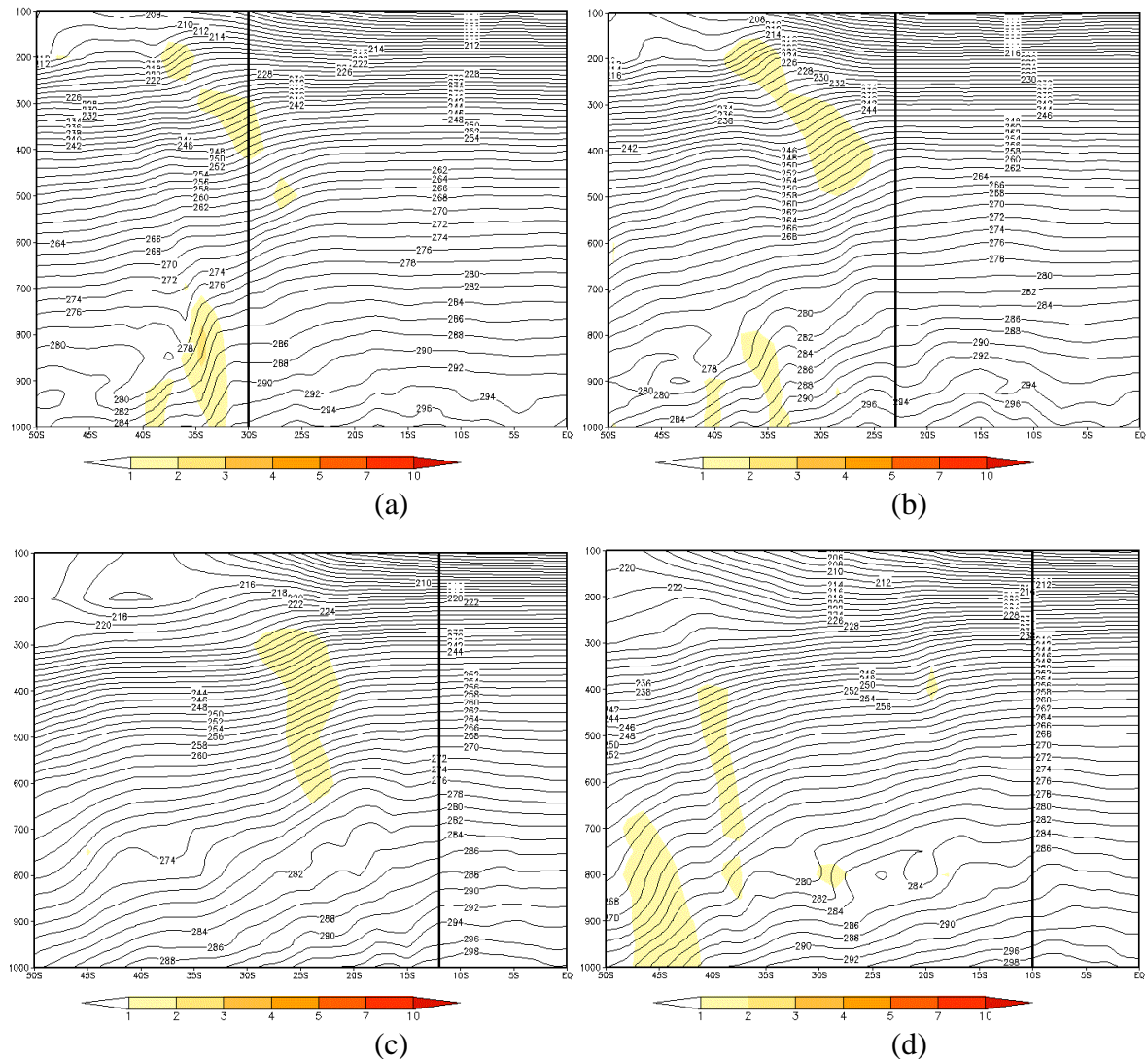
FIGURA 4.25 - Seção Vertical de Temperatura para os dias: a) 19/04/2000 às 06Z (lon 51°W) - POA; b) 20/04/2000 às 06Z (lon 46°W) - SP; c) 23/04/2000 às 12Z (lon 38°W) - SALV e d) 24/04/2000 às 12Z (lon 36°W) - MCZ. FONTE: dados de reanálise do ECMWF.
