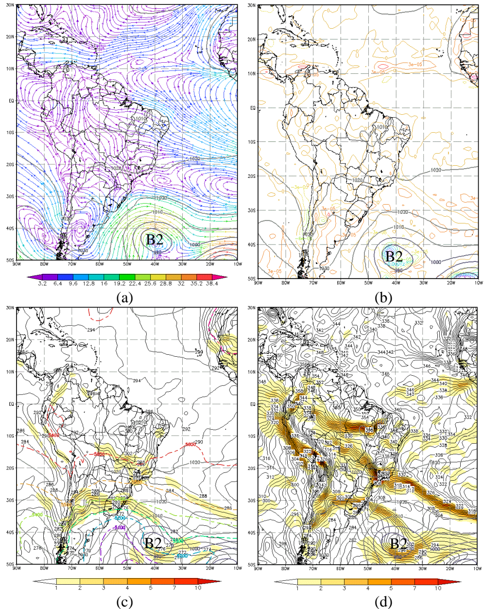
FIGURA 4.14 - Campos meteorológicos em baixos níveis sobrepostos no campo de PNM no dia 27/07/2007 às 18Z: (a) Linhas de Corrente em 925hPa (em cores); (b) Vorticidade Relativa em 925hPa (em cores); (c) Advecção de Temperatura Potencial Equivalente (em cores) e Espessura 500/1000hPa (pontilhada) e (d) Temperatura. FONTE: dados de reanálise do ECMWF.
