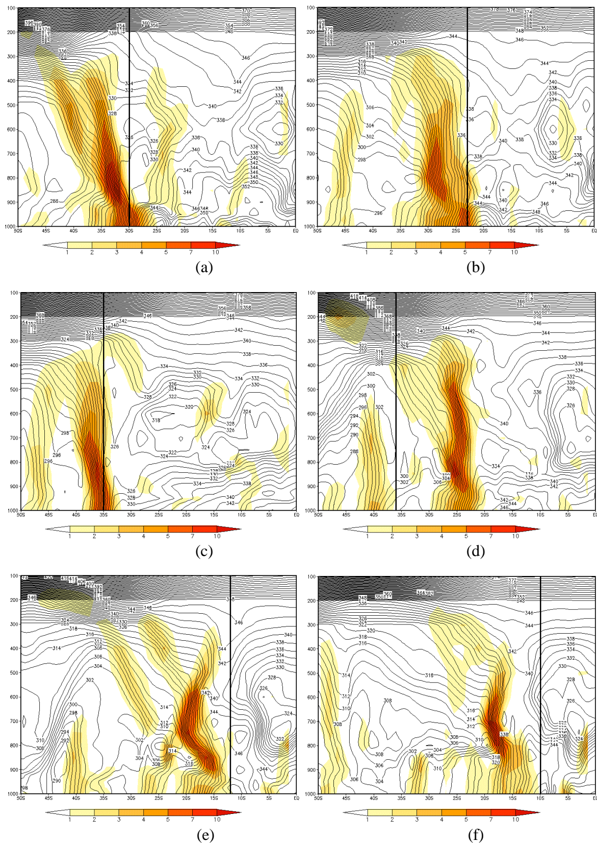
FIGURA 4.44 - Seção Vertical de Temperatura Potencial Equivalente para os dias: a) 01/11/2003 às 06Z (lon 51°W) - POA; b) 02/11/2003 às 06Z (lon 46°W) - SP; c) 03/11/2003 às 00Z (lon 30°W) - regeneração; d) 03/11/2003 às 12Z (lon 36°W) - regeneração; e) 04/11/2003 às 12Z (lon 38°S) - SALV e f) 05/11/2003 às 18Z (lon 36°S) - MCZ. FONTE: dados de reanálise do ECMWF.
