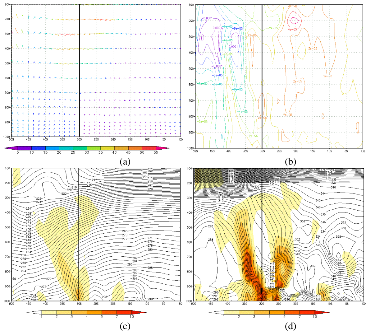
FIGURA 4.12 - Seção Vertical sobre a longitude de Porto Alegre 51°W no dia 25/09/2012 às 00Z de: (a) vento; (b) vorticidade relativa; (c) temperatura e (d) temperatura potencial equivalente. FONTE: de dados de reanálise do ECMWF.
