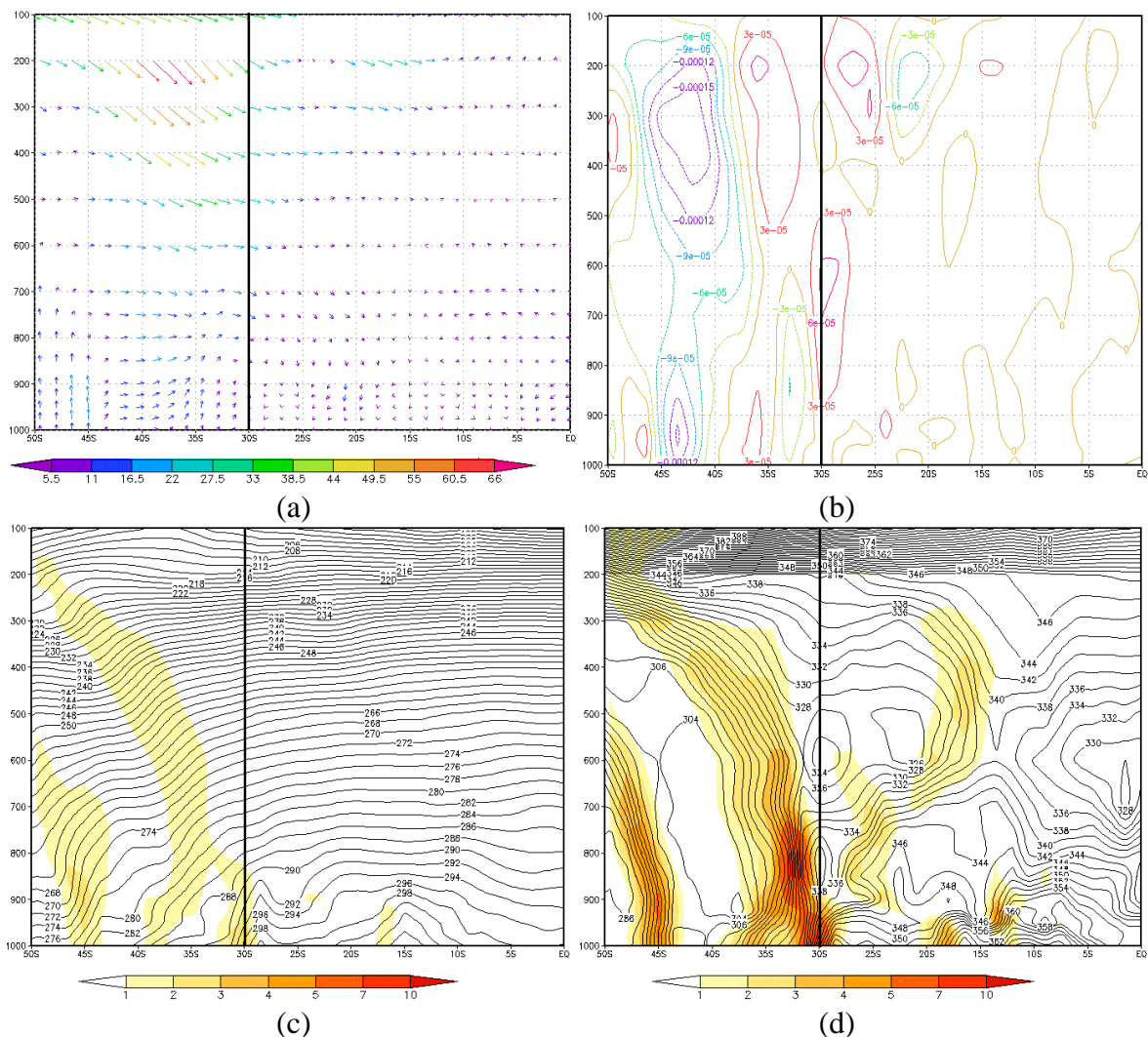
FIGURA 3.3 - Seção Vertical para a cidade de Porto Alegre: a) vento; b) vorticidade relativa; c) temperatura e d) temperatura potencial equivalente. FONTE: dados de reanálise do ECMWF.
