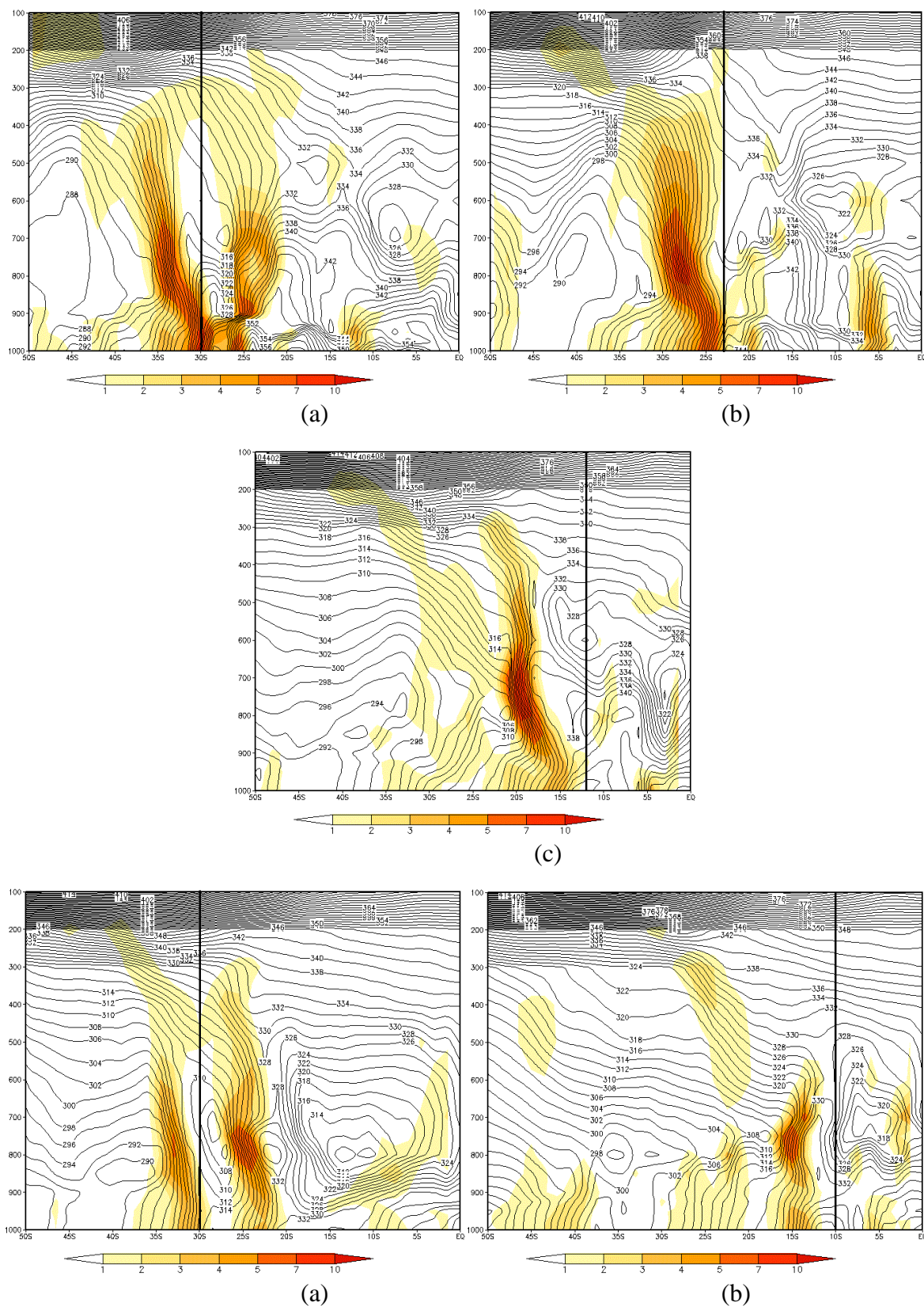
FIGURA 4.55 - Seção Vertical de Temperatura Potencial Equivalente para os dias: a) 25/09/2012 às 00Z (lon 51°W) - POA; b) 26/09/2012 às 00Z (lon 46°W) - SP; c) 27/09/2012 às 12Z (lon 38°W) - SALV; d) 28/09/2012 às 00Z (lon 30°W) - regeneração e e) 29/09/2012 às 18Z (lon 36°W) - MCZ. FONTE: dados de reanálise do ECMWF.
