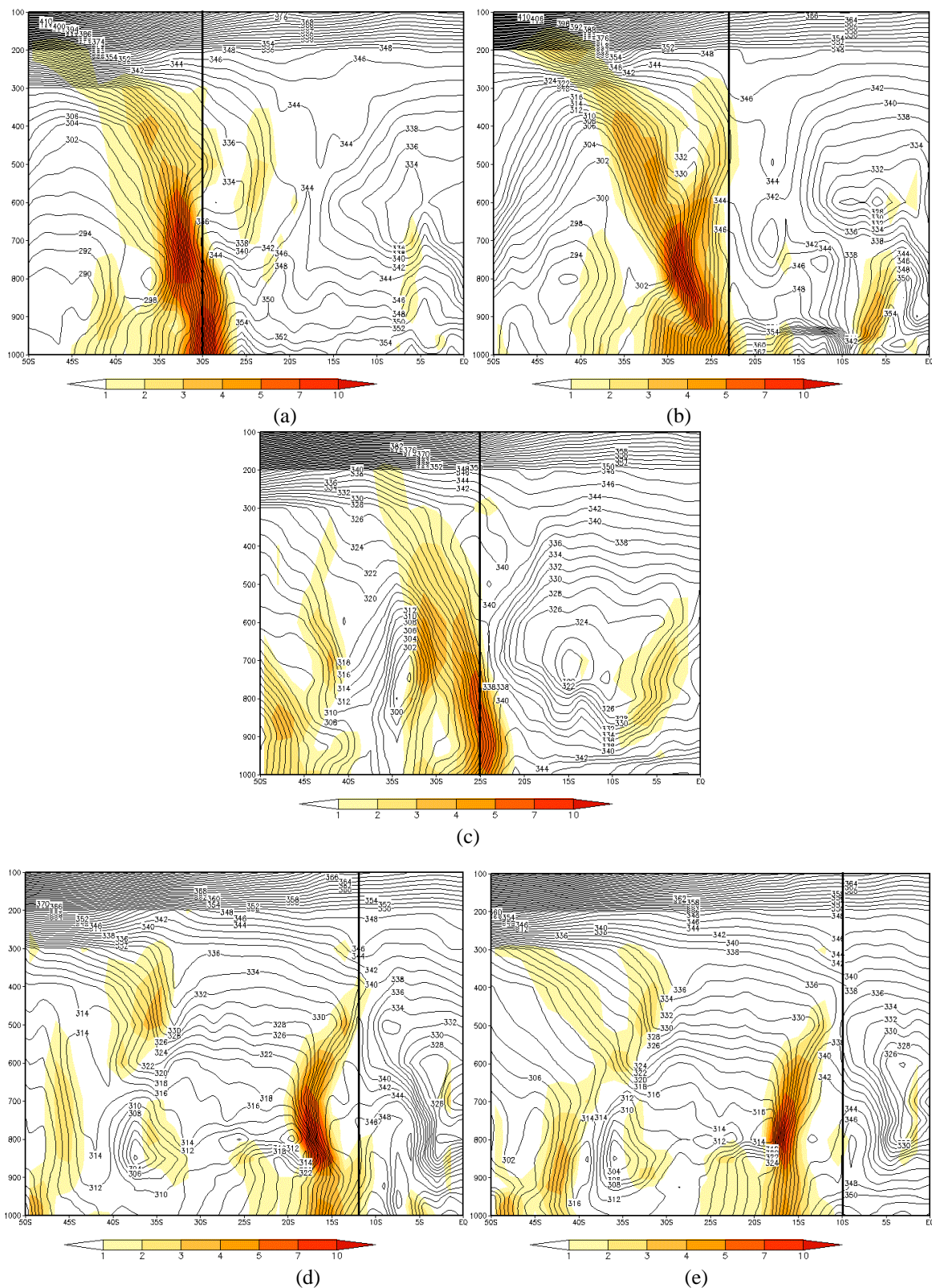
FIGURA 4.59 - Seção Vertical de Temperatura Potencial Equivalente para os dias: a) 01/12/2005 às 12Z (lon 51°W) - POA; b) 02/12/2005 às 0Z (lon 46°W) - SP; c) 04/12/2005 às 00Z (lon 21°W) - regeneração; d) 04/12/2005 às 18Z (lon 38°W) - SALV e e) 05/12/2005 às 00Z (lon 36°W) - MCZ. FONTE: dados de reanálise do ECMWF.
