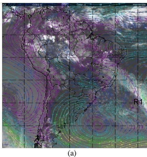
FIGURA 4.67 - Imagens de satélites do campo infravermelho sobrepostos com linhas de correntes para o dia 30/10/2011 às 18Z em: a)925hPa e b)200hPa. FONTE: Adaptada de CPTEC/INPE e ECMWF
