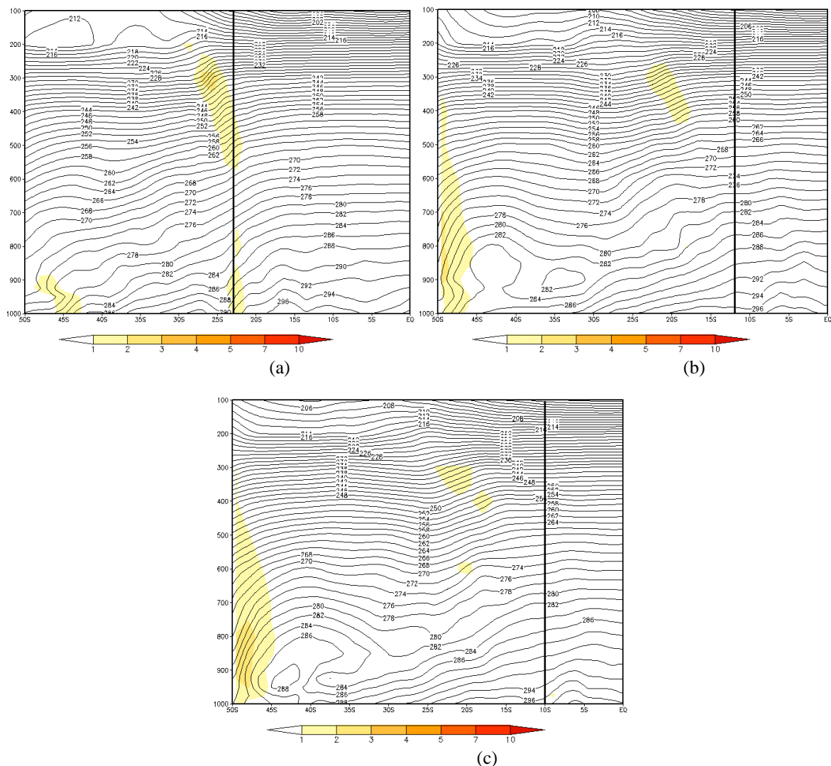
FIGURA 4.73 - Seções Verticais de Temperatura para os dias: a) 30/04/2005 às 12Z (lon 46°W) - SP; b) 02/05/2005 às 06Z (lon 38°W) - SALV; c) 03/05/2005 às 00Z (lon 36°W) - MCZ. FONTE: dados de reanálise do ECMWF
