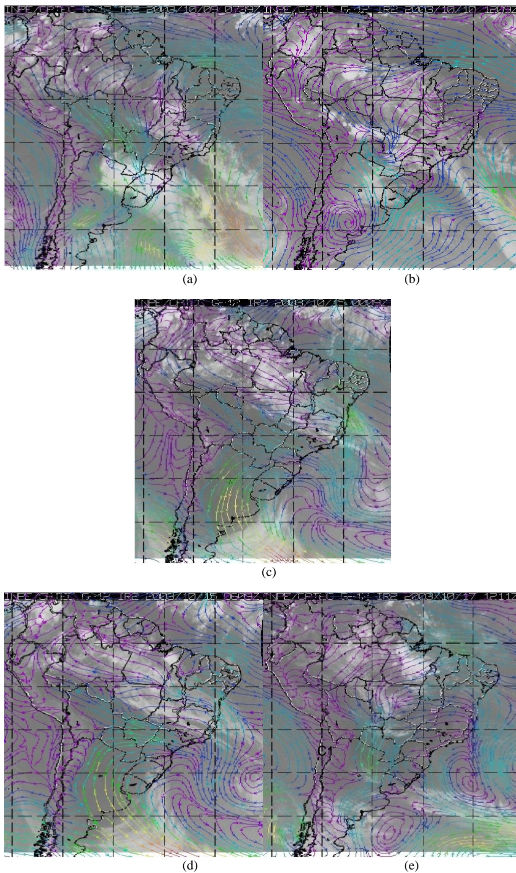
FIGURA 4.38 - Imagem de Satélite do canal infravermelho sobreposto com mapa de linha de corrente de 925hPa para os dias: a) 09/10/2003 às 06Z; b) 10/10/2003 às 12Z; c) 15/10/2003 às 00Z e d) 15/10/2003 às 06Z e e) 17/10/2003 às 12Z. FONTE: Adaptada de CPTEC/INPE e ECMWF
