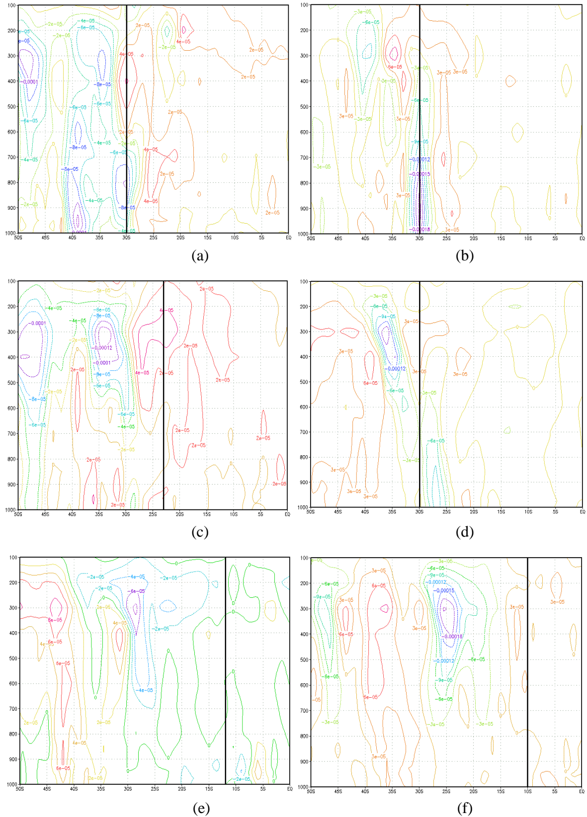
FIGURA 4.22 - Seção Vertical de Vorticidade Relativa para os dias: a) 19/05/2002 às 06Z (lon 51°W) - POA; b) 21/05/2002 às 06Z (lon 47°W) - ciclogênese; c) 21/05/2002 às 12Z (lon 46°W) - SP; d) 23/05/2002 às 12Z (lon 30°W) - regeneração; e) 24/05/2002 às 00Z (lon 38°W) - SALV e f) 26/05/2002 às 00Z (lon 36°W) - MCZ. FONTE: dados de reanálise do ECMWF.
