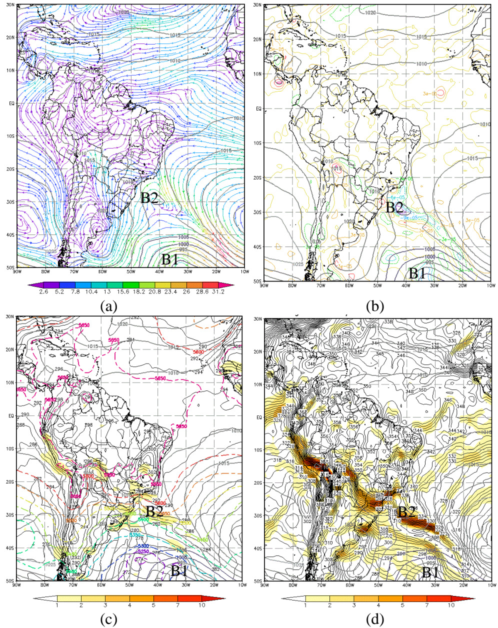
FIGURA 4.17 - Campos meteorológicos em baixos níveis sobrepostos no campo de PNM no dia 30/10/2011 às 18Z: (a) Vento em 925hPa (em cores); (b) Vorticidade Relativa em 925hPa (em cores); (c) Temperatura e Espessura 500/1000hPa (pontilhada) e (d) Temperatura Potencial Equivalente. FONTE: dados de reanálise do ECMWF.
