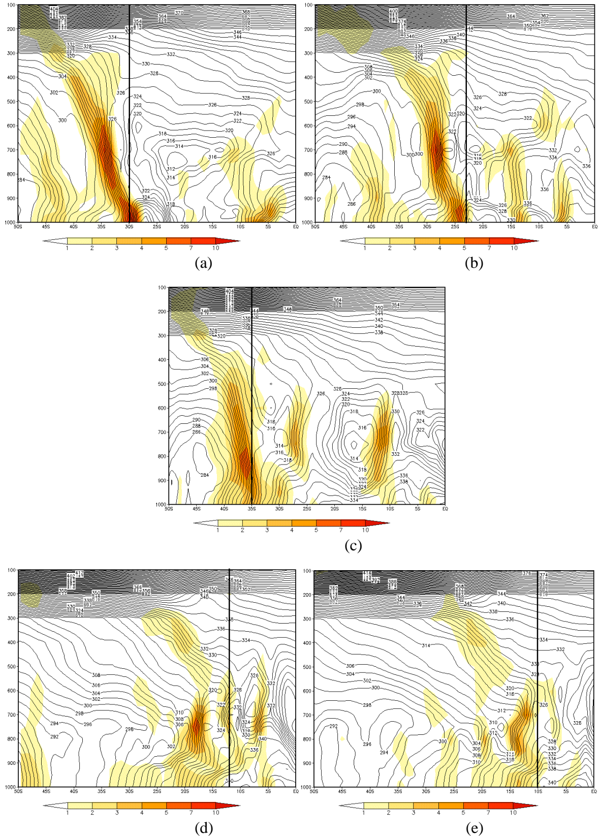
FIGURA 4.28 - Seção Vertical de Temperatura Potencial Equivalente para os dias: a) 06/08/2004 às 12Z (lon 51°W) - POA; b) 08/08/2002 às 00Z (lon 46°W) - SP; c) 08/08/2004 às 06Z (lon 39°W) - ciclogênese; d) 10/08/2004 às 00Z (lon 38°W) - SALV e e) 11/08/2004 às 00Z (lon 36°W) - MCZ. FONTE: dados de reanálise do ECMWF.
