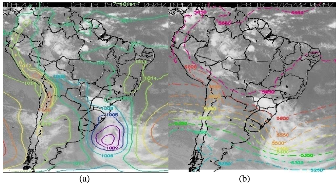
FIGURA 4.2 - Imagem de satélite do canal infravermelho para o dia 19/05/2002 06Z sobreposta com: (a) campo de PNM (b) campo de espessura da camada 500/1000hPa. Fonte: Adaptada de CPTEC/INPE
