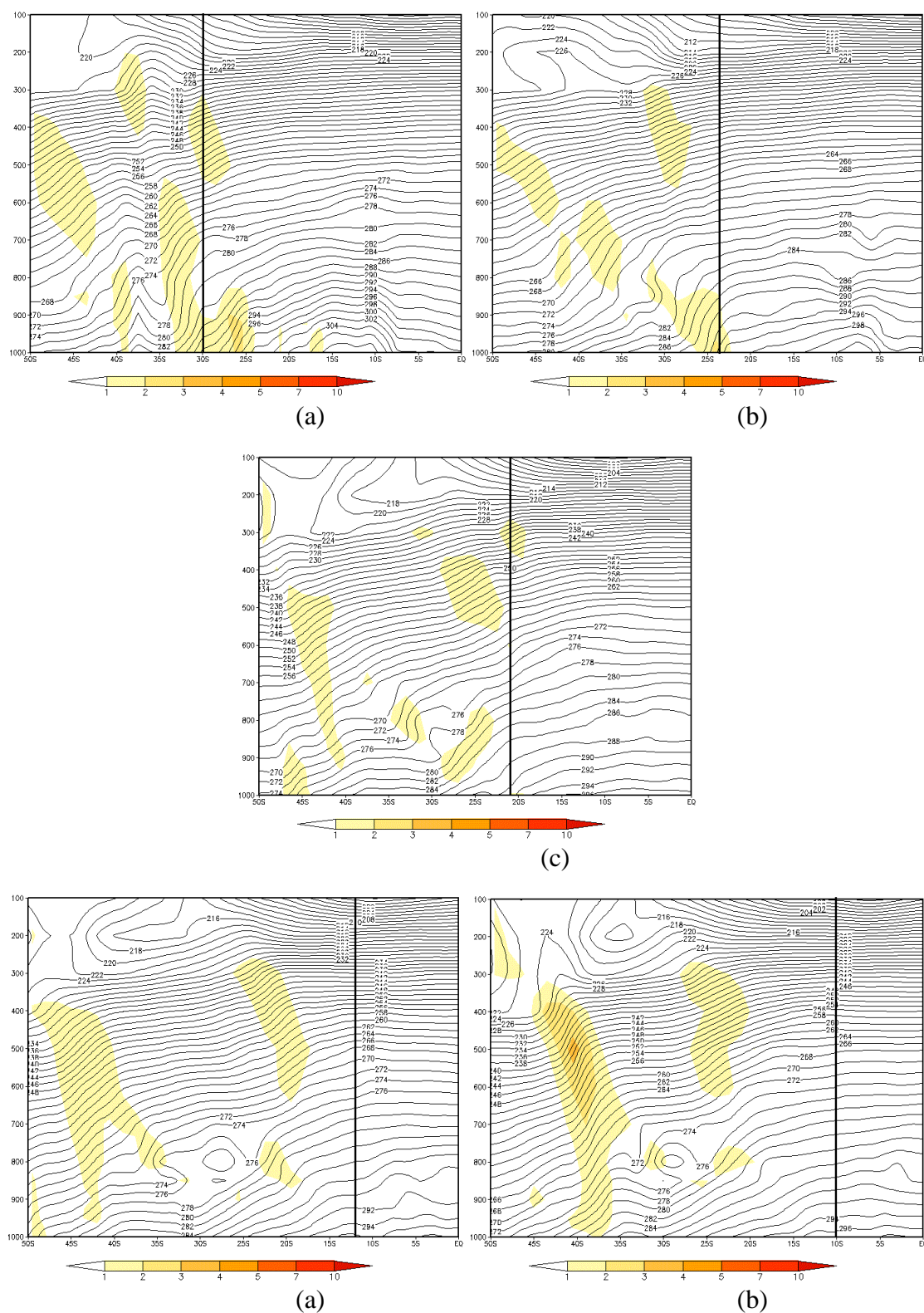
FIGURA 4.56 - Seção Vertical de Temperatura para os dias: a) 31/08/2000 às 12Z (lon 51°W) - POA; b) 01/09/2000 às 12Z (lon 46°W) - SP; c) 05/09/2000 às 00Z (lon 30°W) - regeneração; d) 05/09/2000 às 06Z (lon 38°W) - SALV e e) 06/09/2000 às 06Z (lon 36°W) - MCZ. FONTE: dados de reanálise do ECMWF.
