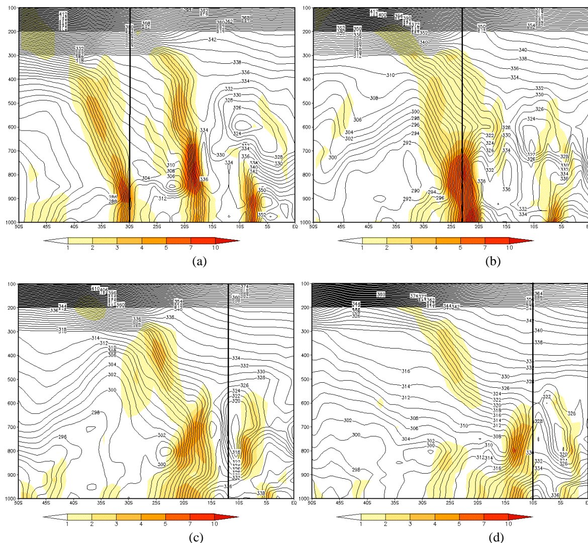
FIGURA 4.64 - Seção Vertical de Temperatura Potencial Equivalente para os dias: a) 27/07/2007 às 18Z (lon 51°W) - POA; b) 29/07/2007 às 00Z (lon 46°W) - SP; c) 30/07/2007 às 00Z (lon 38°W) - SALV e d) 31/07/2007 às 12Z (lon 36°W) - MCZ. FONTE: dados de reanálise do ECMWF.
