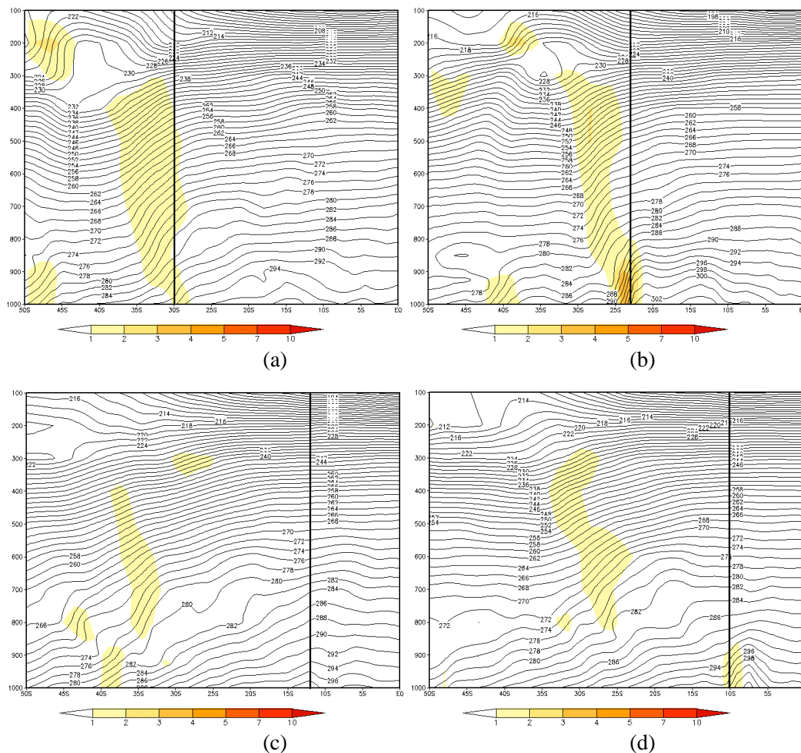
FIGURA 4.34 - Seção Vertical de Temperatura para os dias: a) 30/04/2006 às 12Z (lon 51^{\circ}\text{W} ) - POA; b) 02/05/2006 às 18Z (lon 46^{\circ}\text{W} ) - SP; c) 06/05/2006 às 00Z (lon 38^{\circ}\text{W} ) - SALV e d) 07/05/2006 às 18Z (lon 36^{\circ}\text{W} ) - MCZ. FONTE: Dados de Reanálises do ECMWF.
