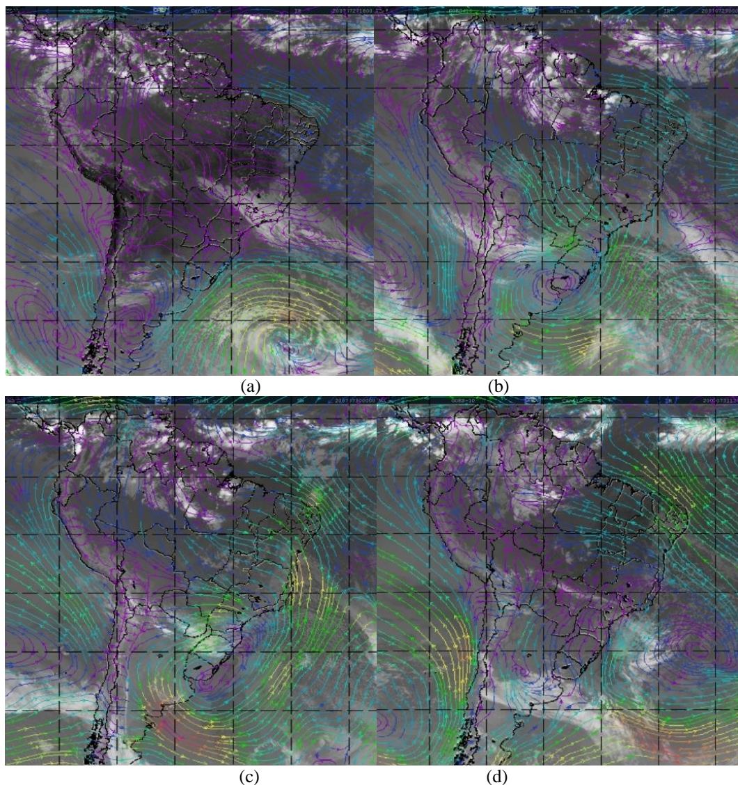
FIGURA 4.60 - Imagem de satélite sobreposta com linhas de correntes em 925hPa para os dias: a) 27/07/2007 às 18Z; b) 29/07/2007 às 00Z; c) 30/07/2007 às 00Z e d) 31/07/2007 às 12Z. FONTE: Adaptada de CPTEC/INPE e ECMWF
