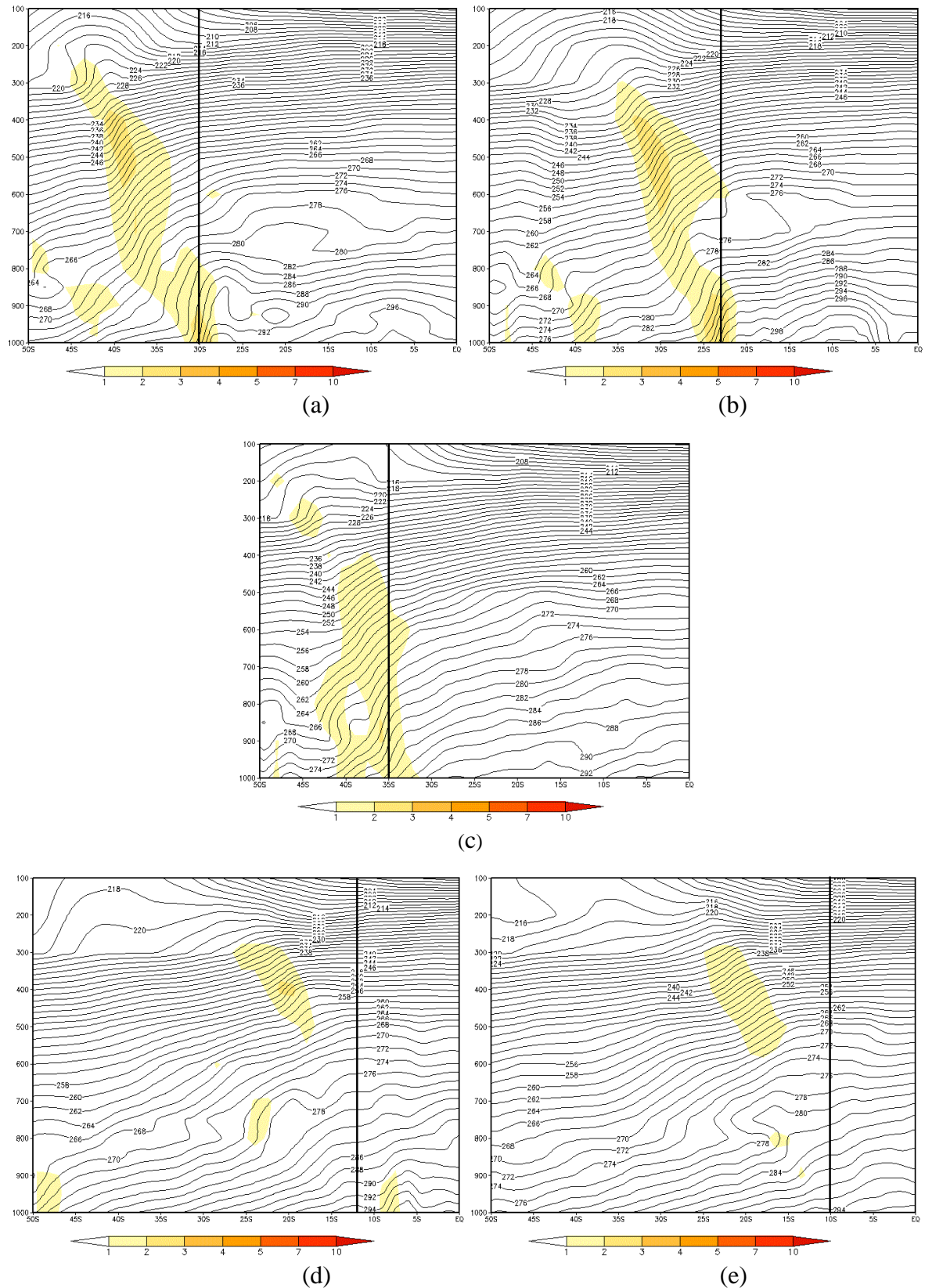
FIGURA 4.27 - Seção Vertical de Temperatura para os dias: a) 06/08/2004 às 12Z (lon 51°W) - POA; b) 08/08/2002 às 00Z (lon 46°W) - SP; c) 08/08/2004 às 06Z (lon 39°W) - ciclogênese; d) 10/08/2004 às 00Z (lon 38°W) - SALV e e) 11/08/2004 às 00Z (lon 36°W) - MCZ. FONTE: dados de reanálise do ECMWF.
