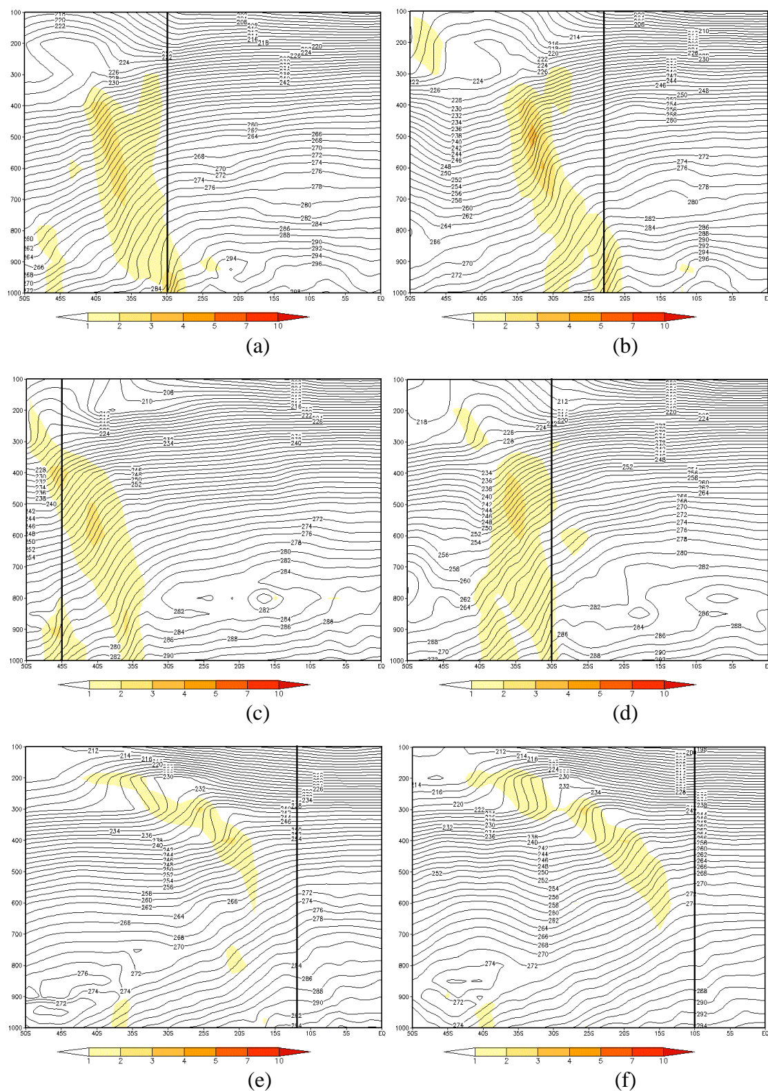
FIGURA 4.45 - Seção Vertical de Temperatura para os dias: a) 15/07/2004 às 12Z (lon 51°W) - POA; b) 17/07/2004 às 06Z (lon 46°W) - SP; c) 17/07/2007 às 12Z (lon 25°W) - regeneração; d) 20/07/2007 às 06Z (lon 12°W) - regeneração; e) 21/07/2004 às 12Z (lon 38°W) - SALV e d) 22/07/2004 às 06Z (lon 36°W) - MCZ. FONTE: dados de reanálise do ECMWF
