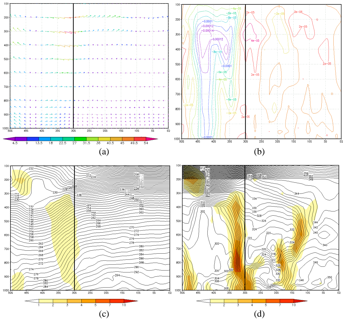
FIGURA 4.6 - Seção Vertical sobre a longitude de Porto Alegre 51^{\circ}\text{W} no dia 30/04/2006 às 12Z de: (a) vento; (b) vorticidade relativa; (c) temperatura e (d) temperatura potencial equivalente. FONTE: de dados de reanálise do ECMWF
