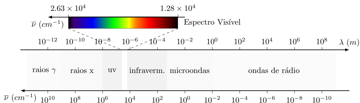
Figura 4.1: Espectro eletromagnético.
