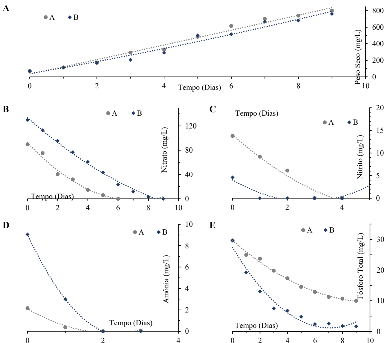
Figura 22 – Análise dos experimentos realizados com efluente subterrâneo real. A) Crescimento celular, B) Concentração de nitrato, C) nitrito, D) amônia e) fósforo total.
