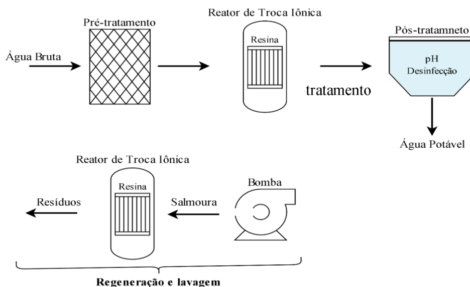
Figura 4 - Esquema de tratamento por troca iônica padrão.
