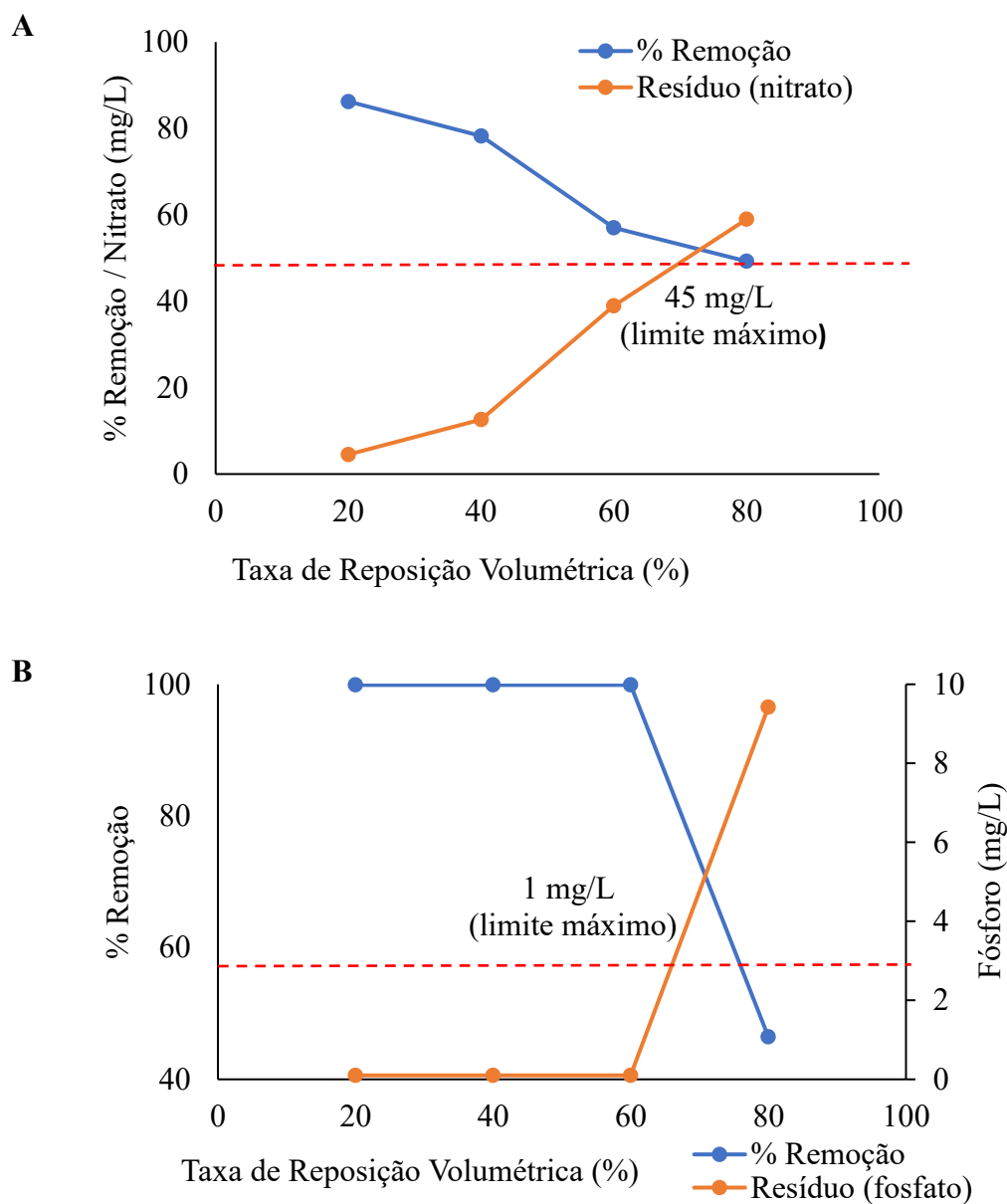
Figura 24 – Remoção de A) nitrato e B) fósforo no sistema semicontínuo.
