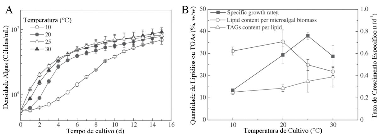
Figura 8 - Curva de crescimento da Tetrademus sp. LX1 (A) e quantidade de lipídio por biomassa para diferentes temperaturas.
