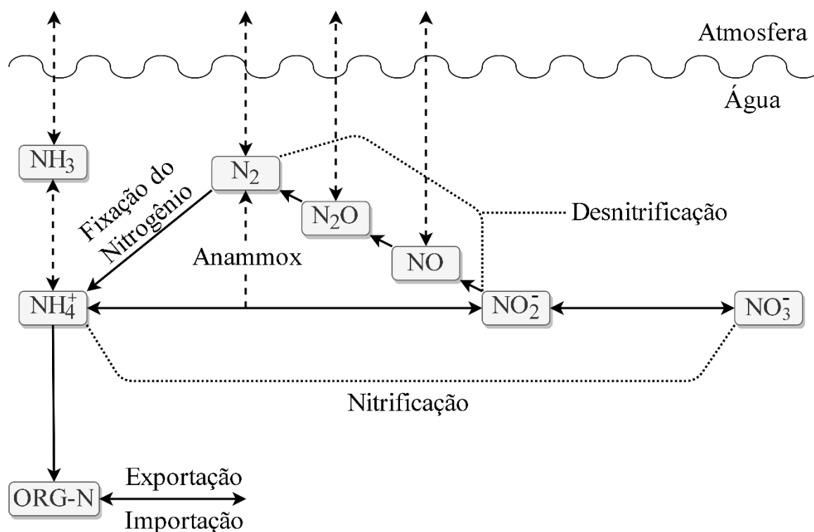
Figura 3 - Rotas de interconversão entre as diferentes formas nitrogenadas.
