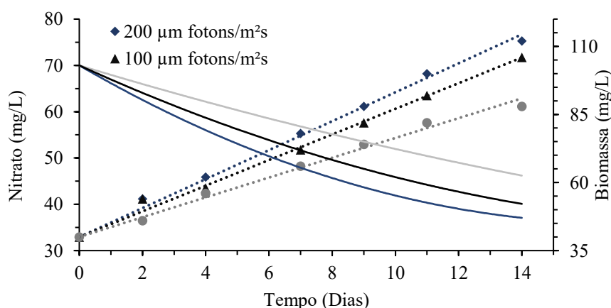
Figura 19 - Crescimento da Tetrademus sp. sob a influência de diferentes luminosidades.
