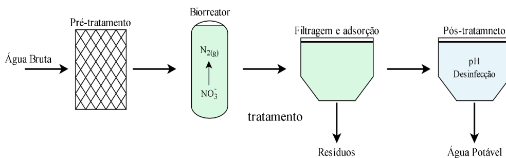
Figura 7 - Esquema padrão do tratamento por desnitrificação biológica.
