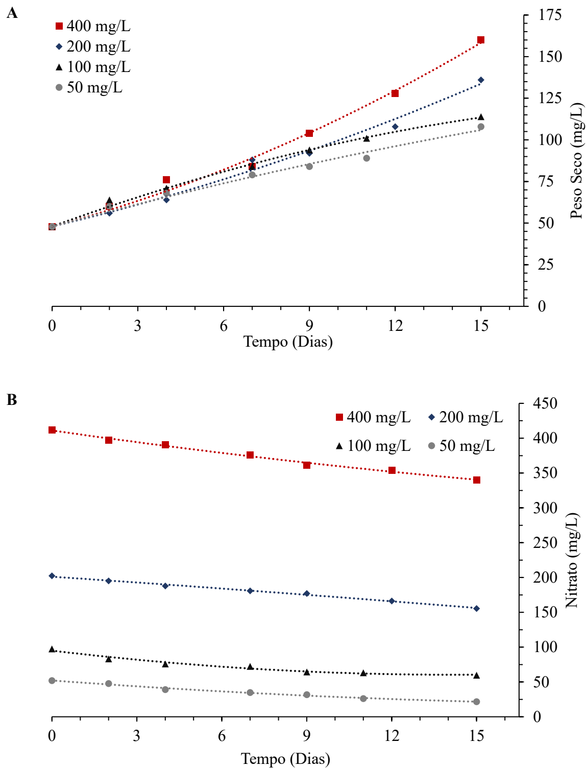
Figura 20 - Crescimento microalgal (A) e remoção de nitrato (B) para diferentes concentrações de nitrato.
