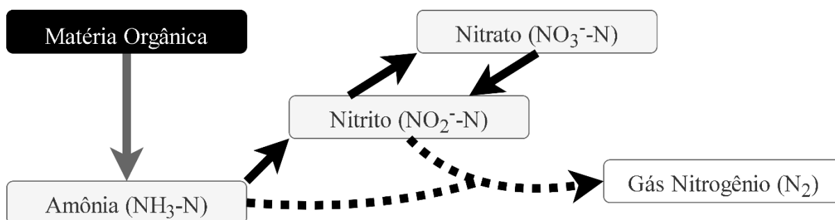
Figura 1 - Degradação da matéria orgânica, nitrificação parcial e desnitrificação.
