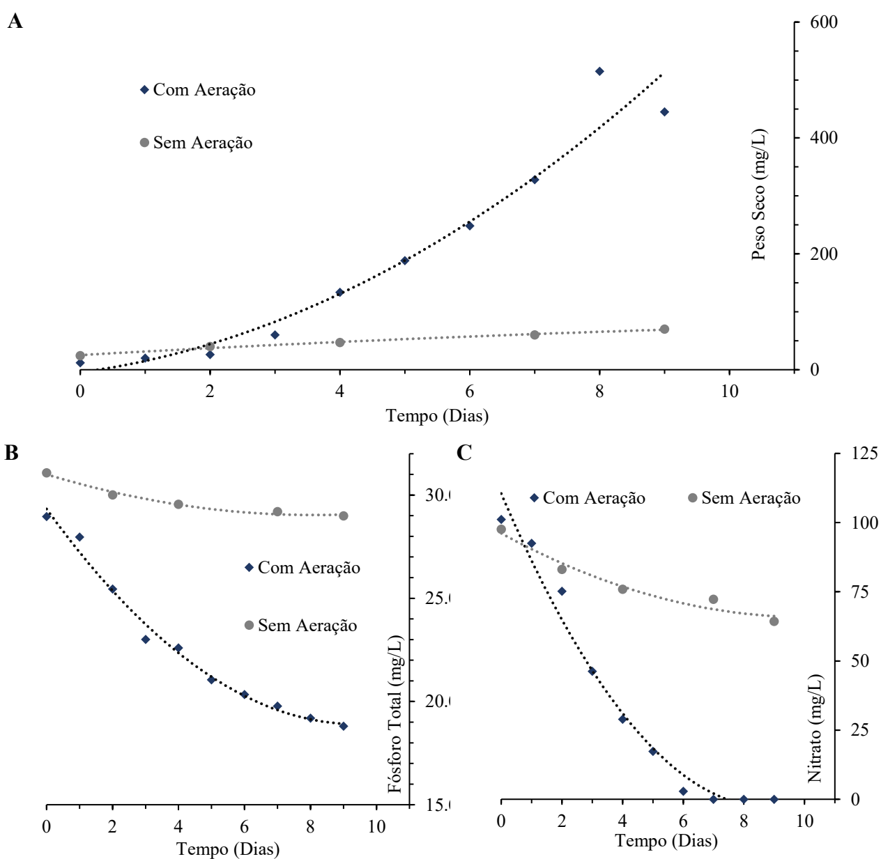
Figura 21 - Comparação de desempenho dos reatores com e sem aeração. A) Crescimento celular, B) Concentração de fósforo e C) Concentração de nitrato com o tempo de tratamento.
