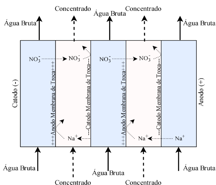
Figura 6 - Esquema padrão de tratamento por eletrodiálise.
