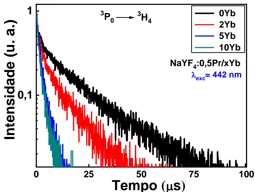
Figura 4.5: Curvas de decaimento do nível 3 P 0 (transição Pr 3+ : 3 P 0 → 3 H 4 - 483 nm) nos nanocristais de NaYF 4 :0,5Pr 3+ /xYb 3+ (x = 0, 2, 5, e 10 mol%), sob excitação em 442 nm.
