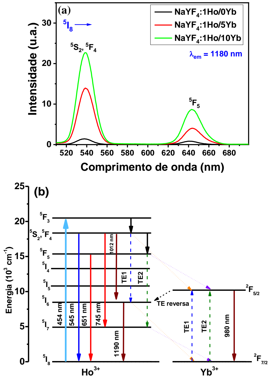
Figura 3.1: (a) Espectros de excitação dos nanocristais de \text{NaYF}_4:1\text{Ho}/x\text{Yb} ( x = 0, 5 e 10 mol.%) referente a emissão em torno de 1180 nm ( \text{Ho}^{3+}: {}^5\text{I}_6 \rightarrow {}^5\text{I}_8 ). (b) Diagrama simplificado dos níveis de energia do sistema \text{Yb}^{3+}/\text{Ho}^{3+} mostrando o processo de quantum cutting envolvido: decaimentos não-radioativos do \text{Ho}^{3+} com subseqüentes transferências de energia para os íons de \text{Yb}^{3+} .
