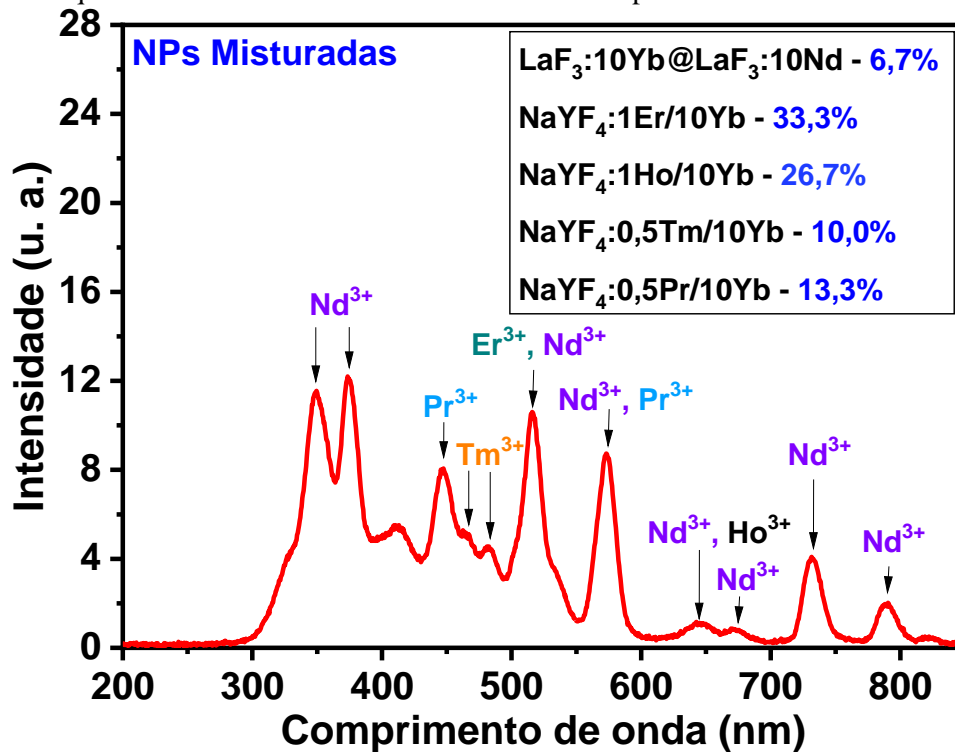
Figura 5.9: Espectro de excitação das NPs misturadas, monitorando a emissão em 980 nm. A proporção em que cada NP foi colocada está discriminada em peso%.
