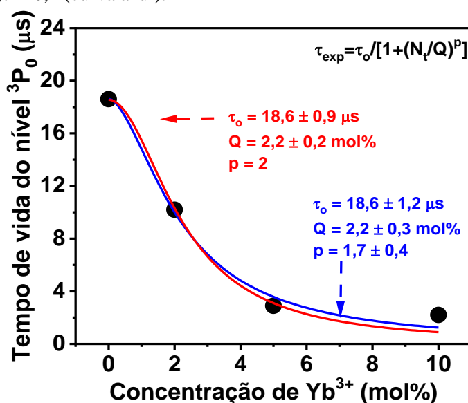
Figura 4.6: Tempo de vida do nível ^3\text{P}_0 do \text{Pr}^{3+} em função da concentração de \text{Yb}^{3+} . As linhas cheias representam o melhor ajuste obtido a partir do uso da Equação 4.1 usando p = 2 (curva vermelha) e p = 1,7 \pm 0,4 (curva azul).
