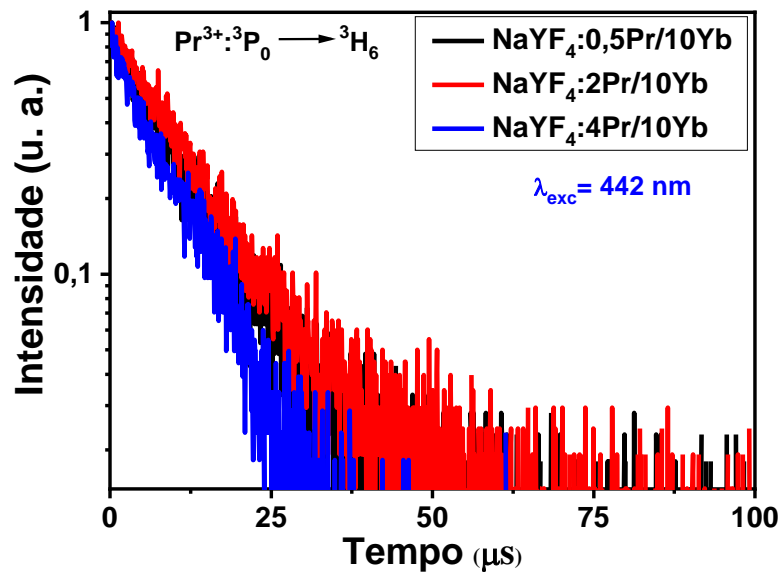
Figura 4.9: Curvas de decaimento da transição \text{Pr}^{3+}:^3\text{P}_0 \rightarrow ^3\text{H}_6 (605 nm) nos nanocristais de \text{NaYF}_4:\text{xPr}^{3+}/10\text{Yb}^{3+} ( x = 0,5; 2,0 e 4,0 mol%), sob excitação em 442 nm.
