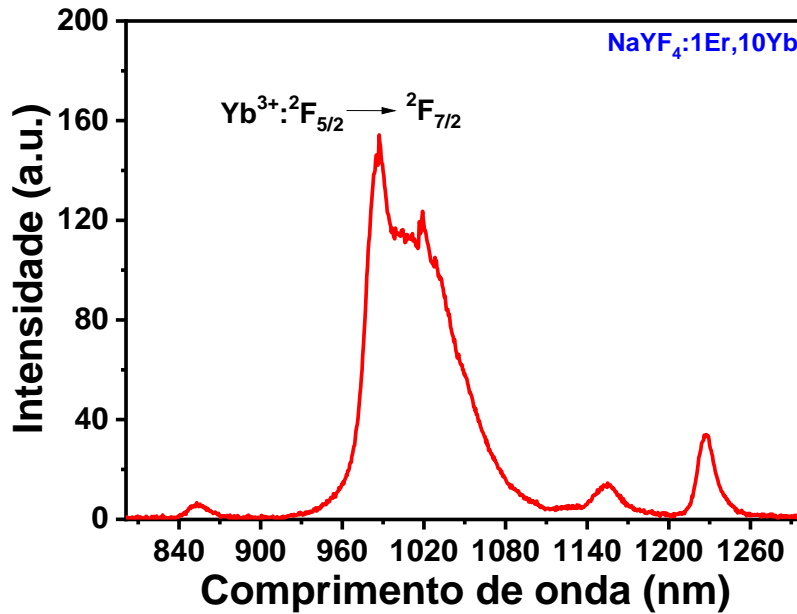
Figura 5.3: Espectro de emissão dos nanocristais de \text{NaYF}_4:1\text{Er}/10\text{Yb} na região do infravermelho próximo, sob excitação de 379 nm.
