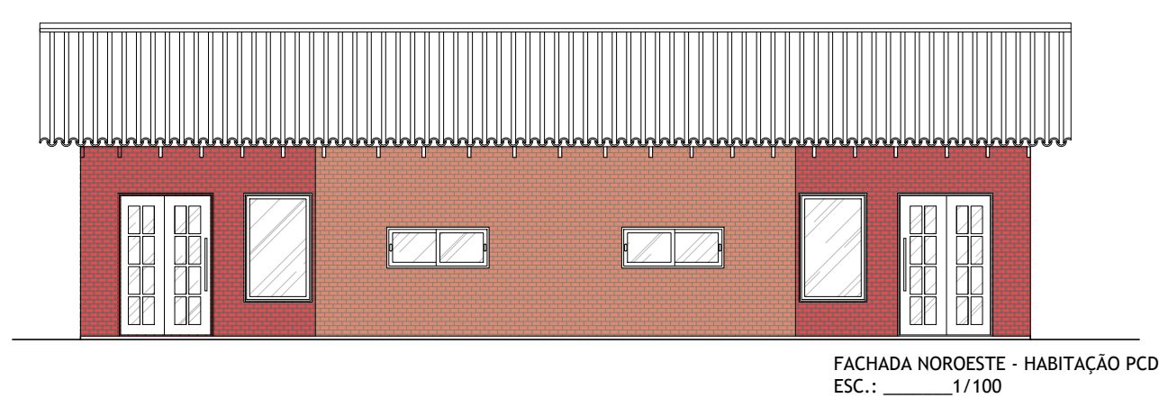
FACHADA NOROESTE - HABITAÇÃO PCO ESC.: 1/100
