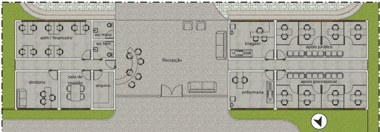
Figura 22: Planta baixa do setor de serviços
