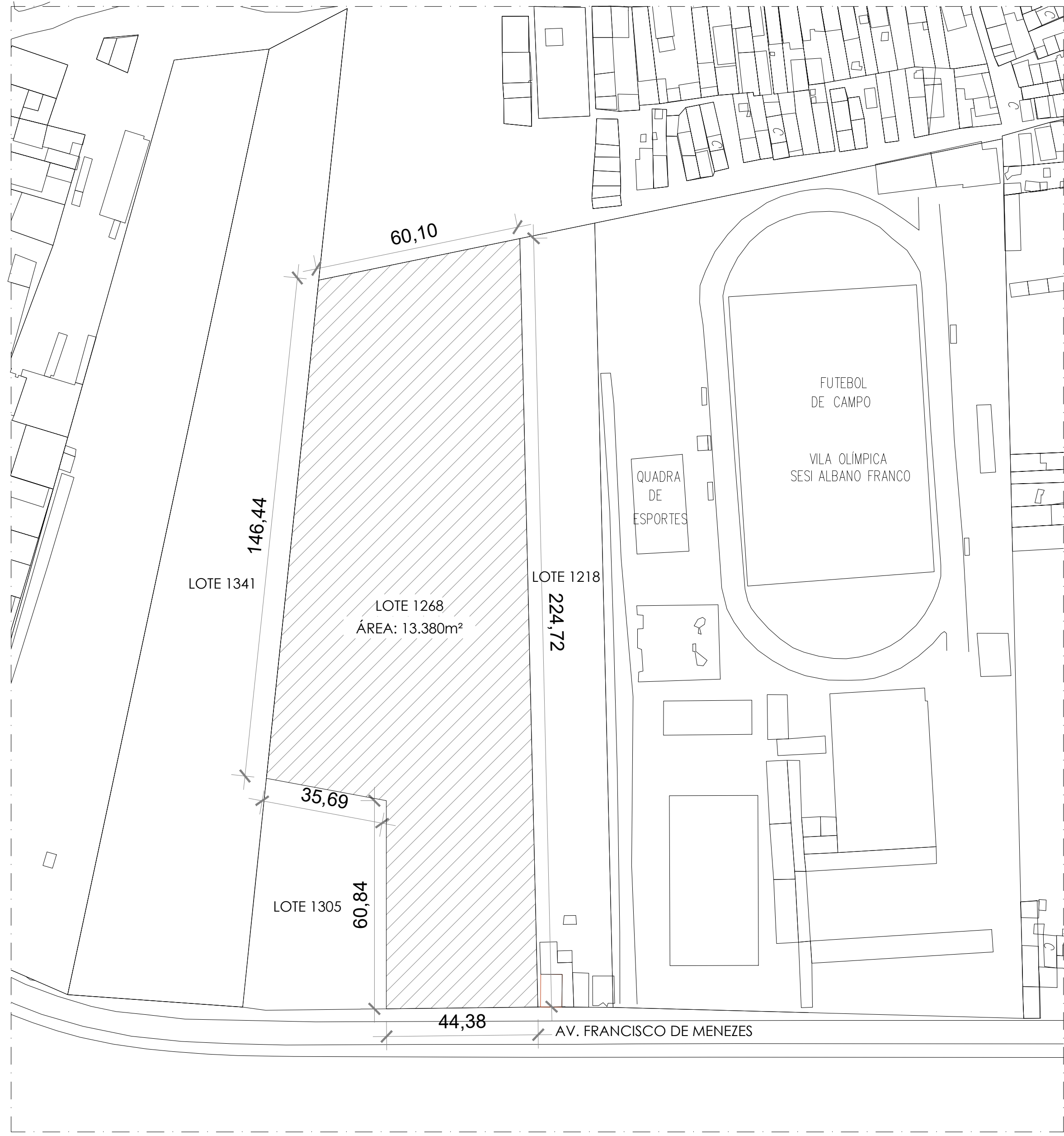
PLANTA DE LOCAÇÃO ESC.: 1/1000
