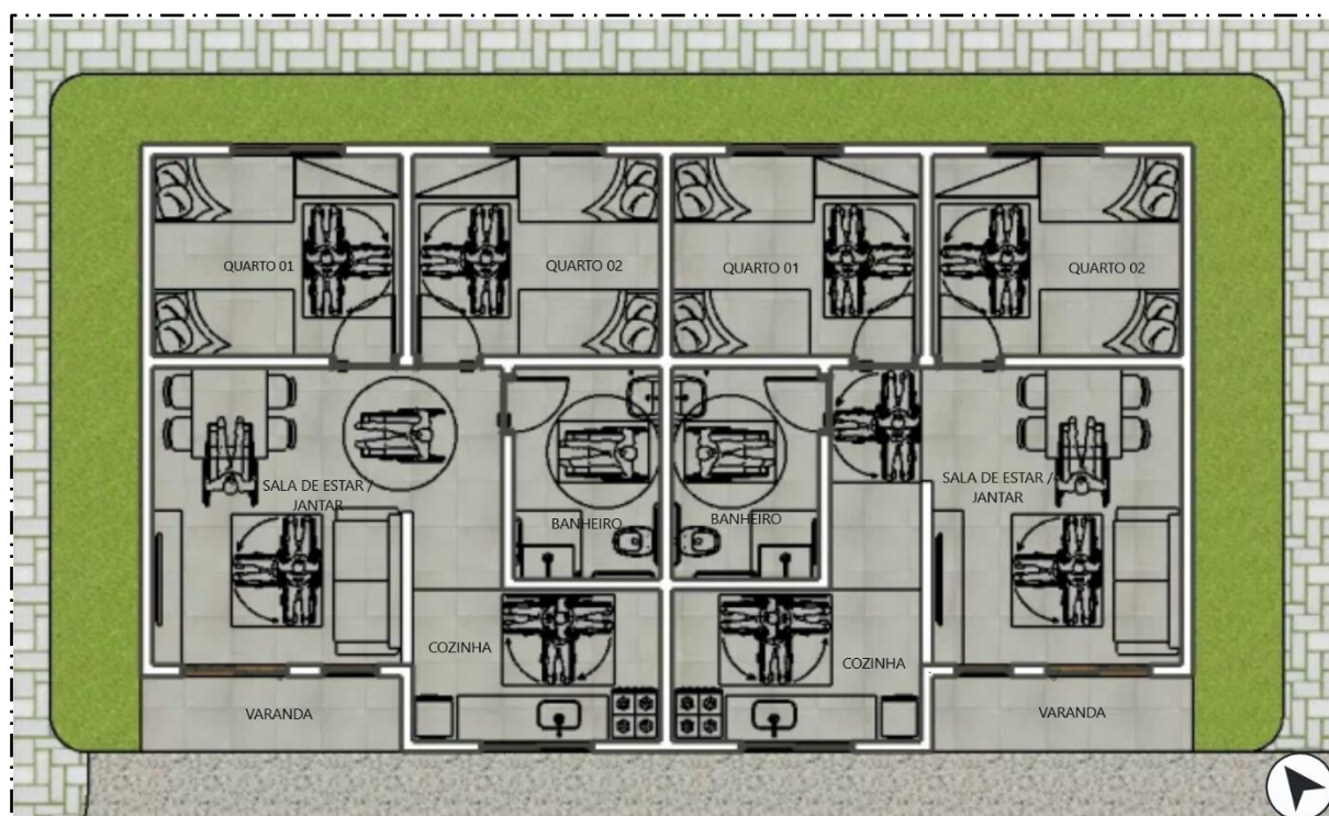
Figura 26: Planta baixa da unidade habitacional PCD
