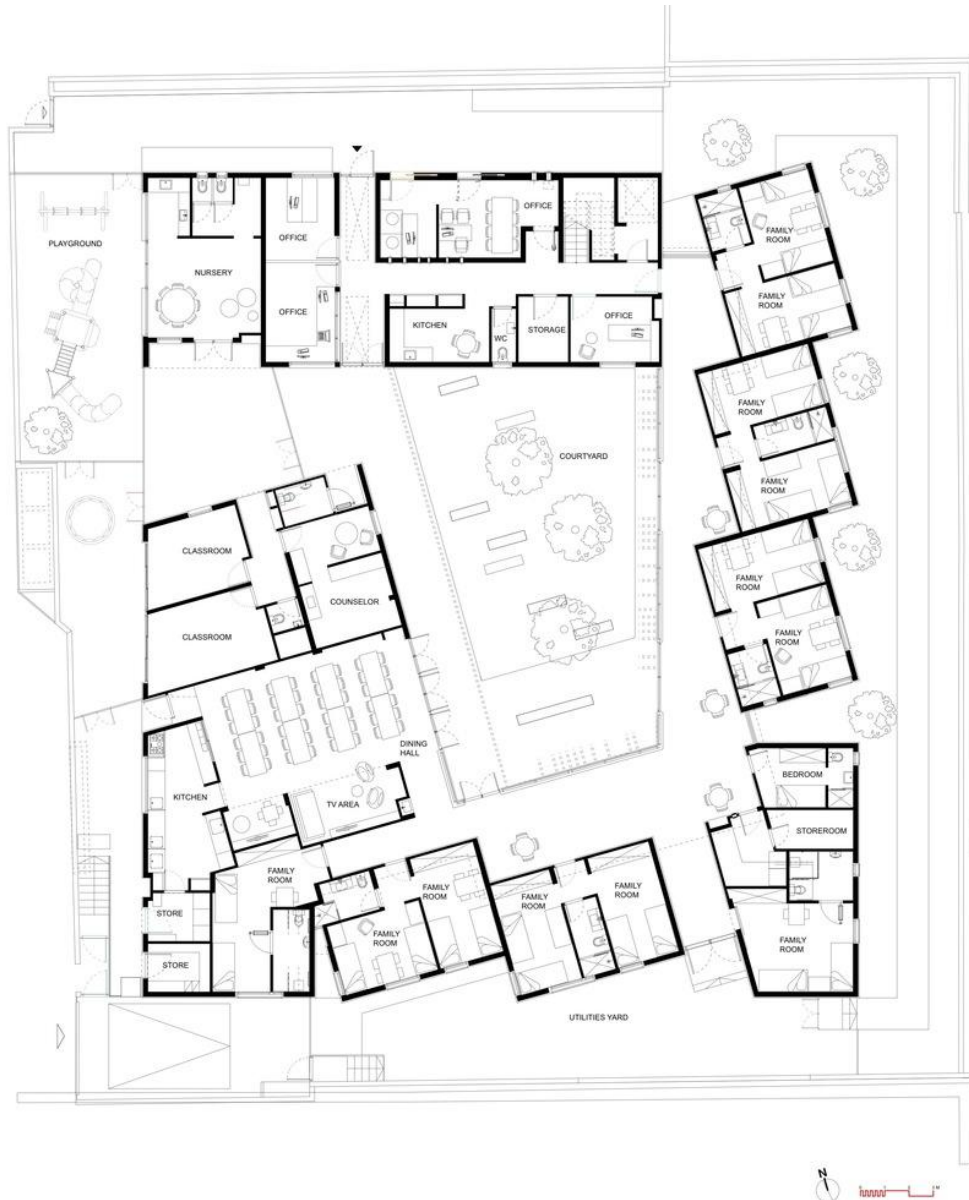
Figura 14: Planta baixa do térreo do edifício.
