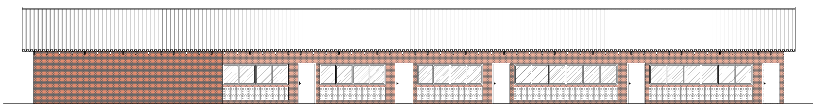
FACHADA NOROESTE - OFICINAS ESC.: 1/100
