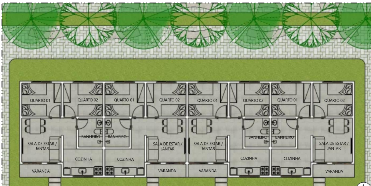
Figura 27: Planta baixa da unidade habitacional.
