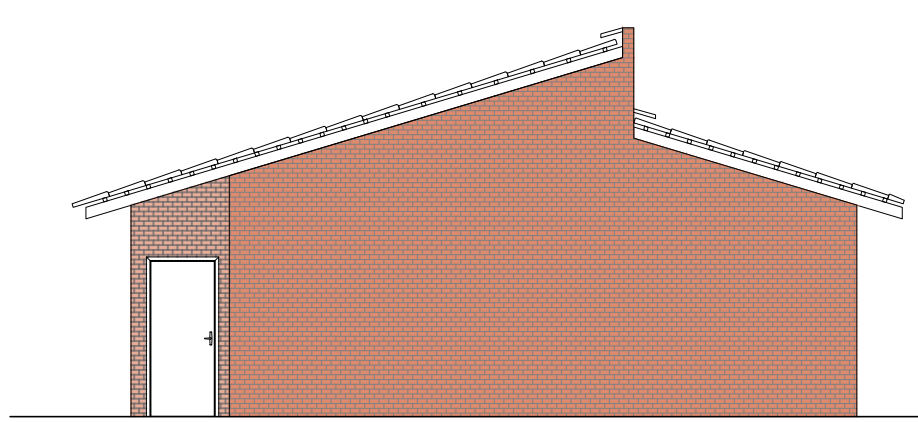
FACHADA SUDESTE - OFICINAS ESC.: 1/100
