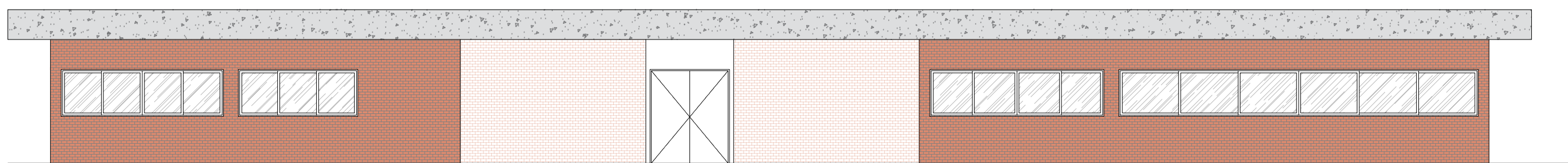
FACHADA NOROESTE - SERVIÇOS ESC.: 1/100
