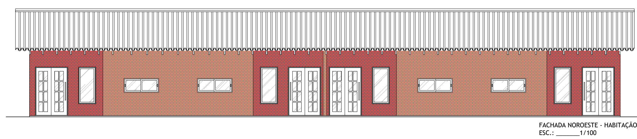
FACHADA NOROESTE - HABITAÇÃO ESC.: 1/100
