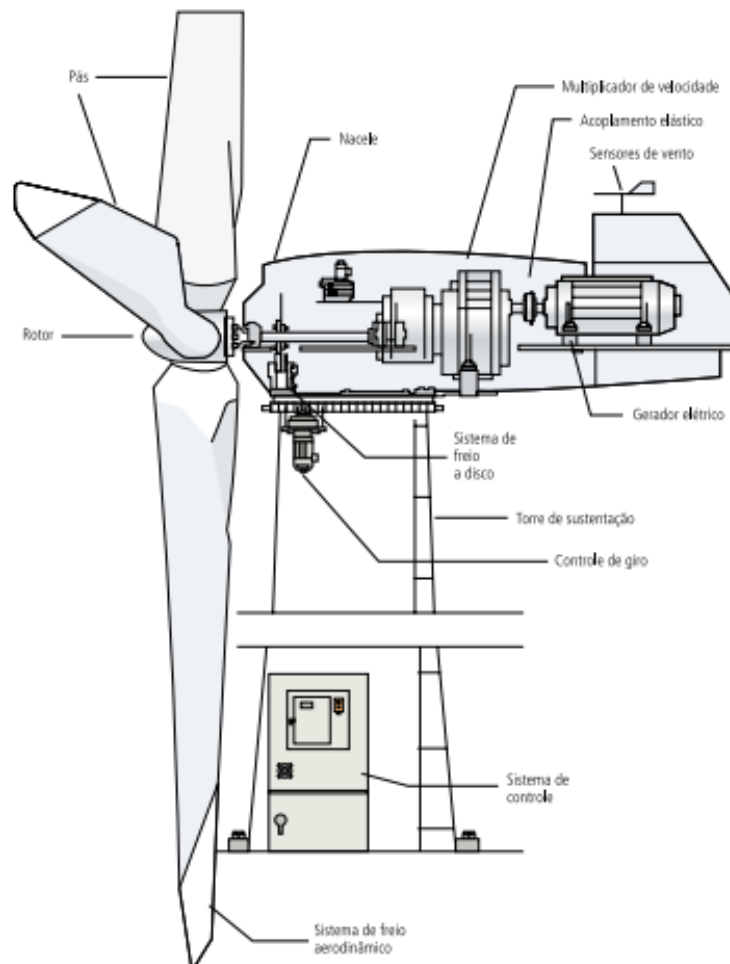
Figura 14: Desenho esquemático da turbina eólica moderna
