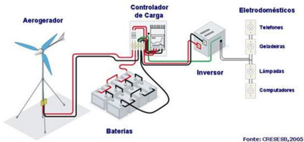
Figura 16: Sistema Eólico Isolado
