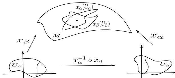
Figura 1 - Variedade diferenciável
