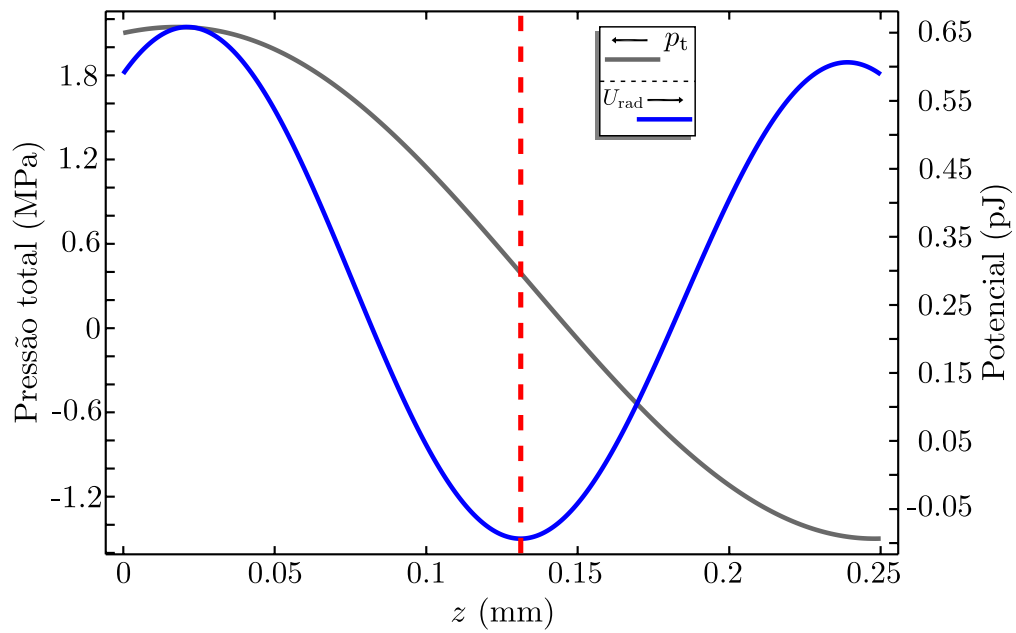
Figura 18 – Pressão total ( p_t ) (curva cinza) e potencial da força de radiação U_{\text{rad}} (curva azul) ao longo do eixo z para x = 0 , a linha trasejada marca a altura do plano de levitação.
