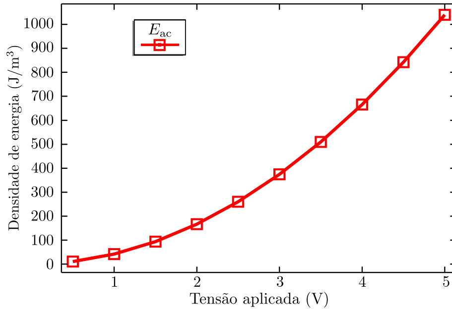
Figura 16 – Densidade de energia acústica média E_{ac} versus a tensão aplicada
