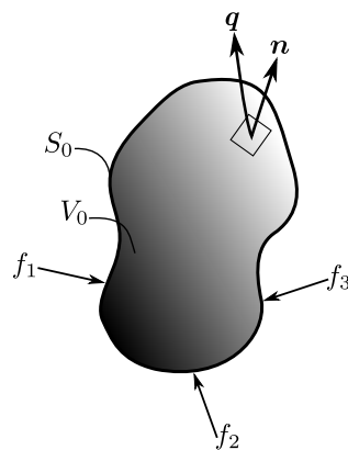
Figura 4 – Vetor tração \mathbf{q} de meio contínuo de volume V_0 e superfície S_0 em virtude das forças externas f_i (i = 1, 2, 3)
