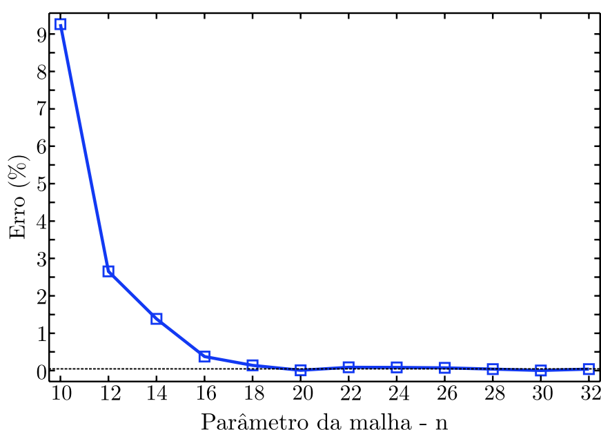
Figura 11 – Gráfico de convergência do modelo, onde a linha tracejada se refere ao valor usado na simulação.
