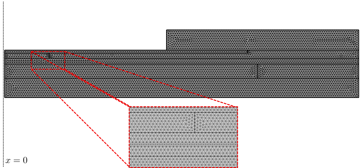
Figura 10 – Discretização da malha no modelo, onde o zoom foi utilizado para a melhor visualização da geometria dos elementos.
