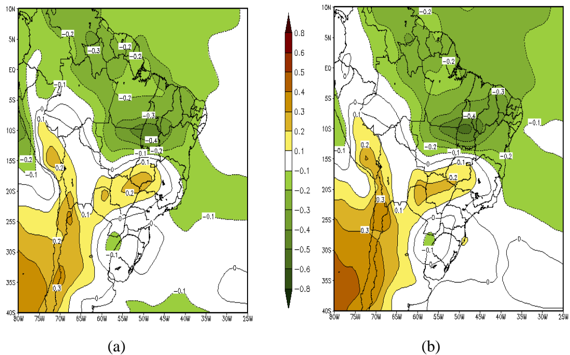
Figura 42: Coeficientes de Correlação entre pressão ao nível do mar e IAS para o período entre 1977-1998 (fase quente), com índice adiantado em (a) 4 meses e (b) 5 meses. Fonte dos dados ESRL/PSD/NOAA.
