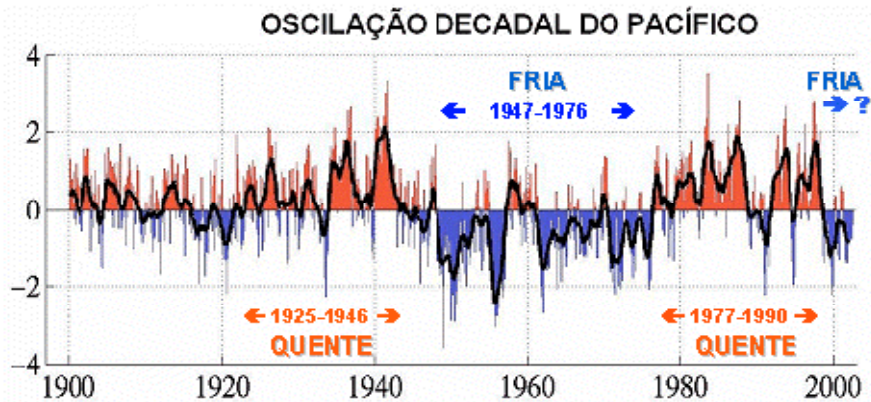
Figura 8: Série temporal do Índice da Oscilação Decadal do Pacífico, adaptada de MANTUA et al(1997).
