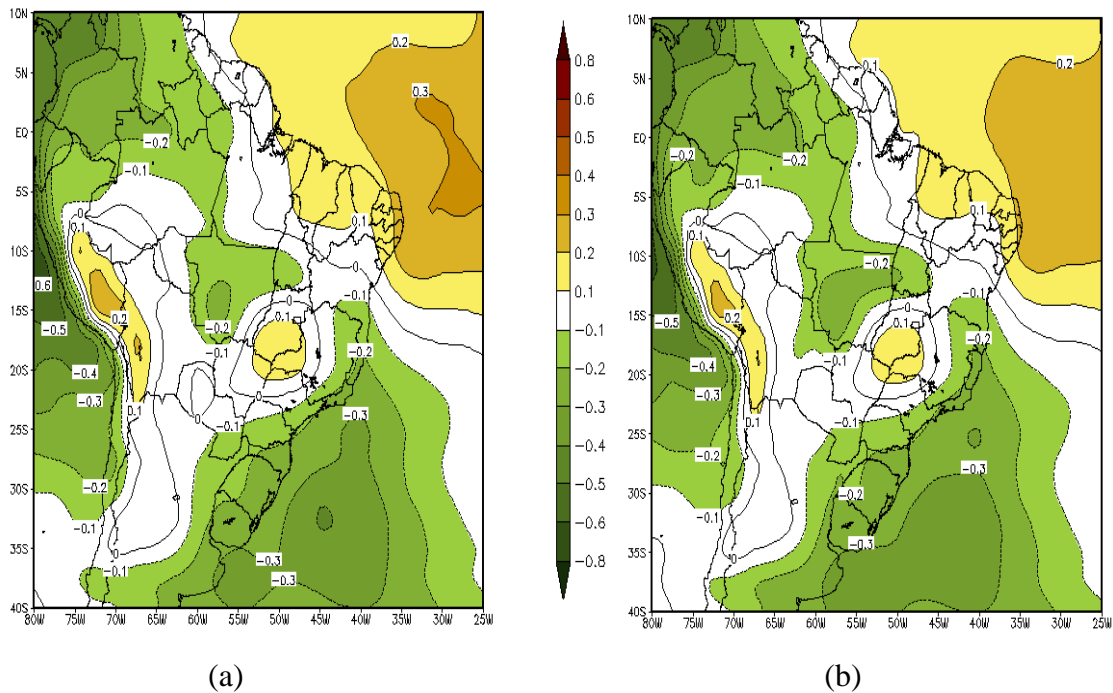
Figura 40: Coeficientes de Correlação entre pressão ao nível do mar e IAS para o período entre 1977-1998 (fase quente), com índice adiantado em (a) simultâneo (b) 1 mês. Fonte dos dados ESRL/PSD/NOAA.
