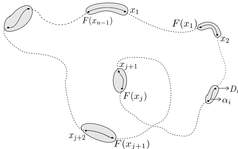
Figura 3.8: Arcos poligonais \alpha_i e discos D_i .
