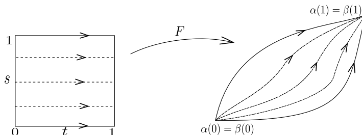
Figura 1.3: Caminhos homotópicos.
