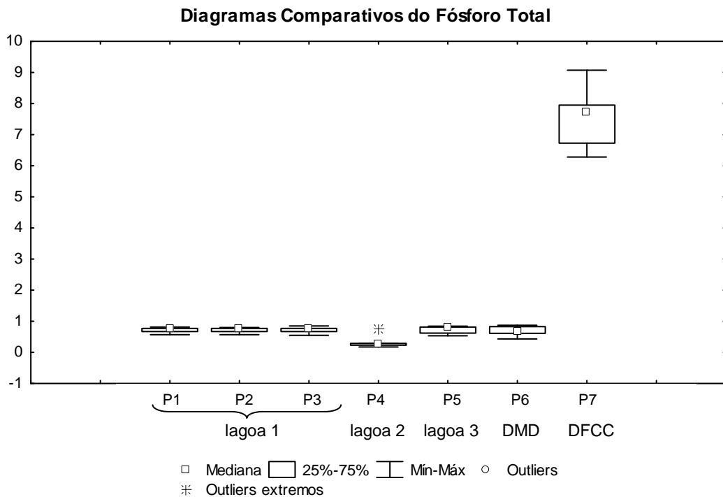
Figura 62 – Diagramas de caixa comparativos de fósforo total (mg/L) nos locais de coleta.
