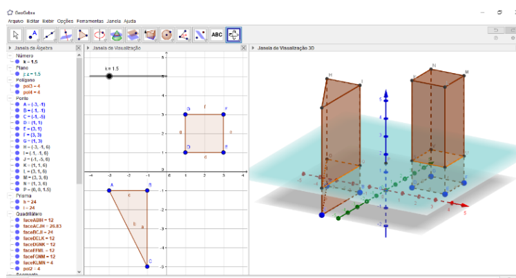
Figura 24: Plano paralelo ao plano das bases seccionando os prismas
