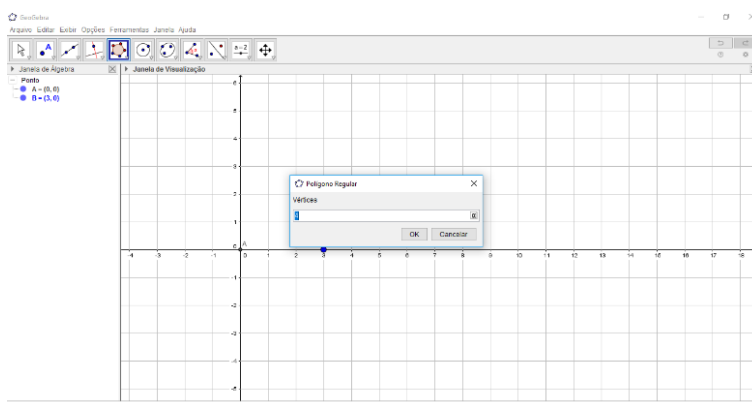
Figura 1: Escolha do número de vértices do polígono regular (4 lados)
