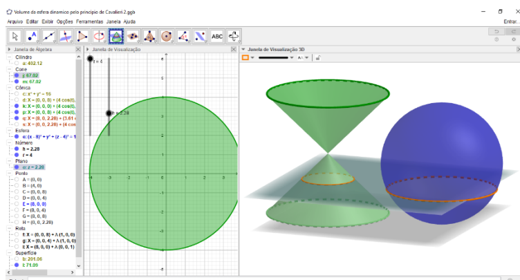
Figura 58: Interseção do plano com a superfície do cone
