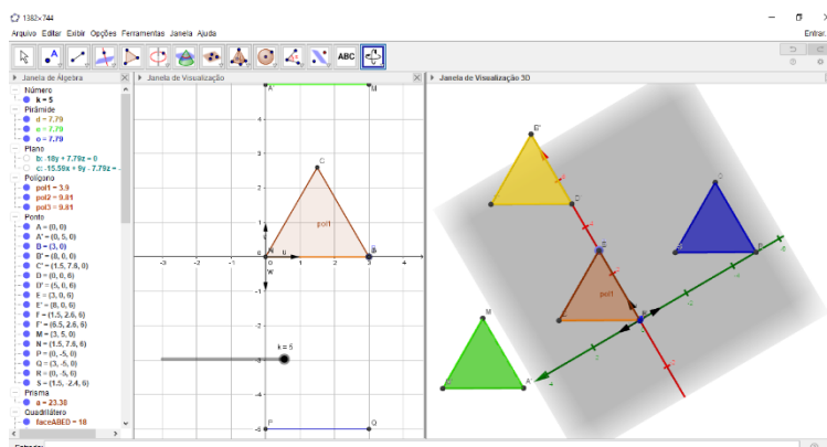
Figura 46: Vista superior das pirâmides que compõem o prisma, separadas
