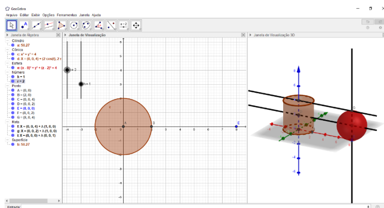
Figura 56: Cilindro equilátero e esfera, ambos de mesmo raio variável
