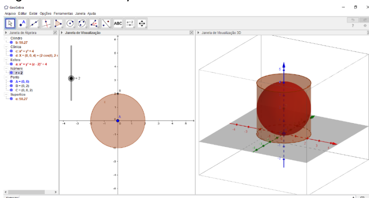
Figura 62: Cilindro equilátero de raio variável e esfera inscrita de mesmo raio
