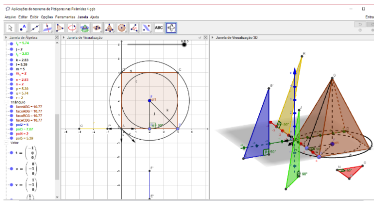
Figura 39: Segundo triângulo retângulo cuja hipotenusa é a aresta da pirâmide
