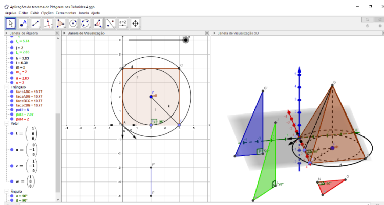
Figura 38: Triângulo retângulo cuja hipotenusa é o raio da base
