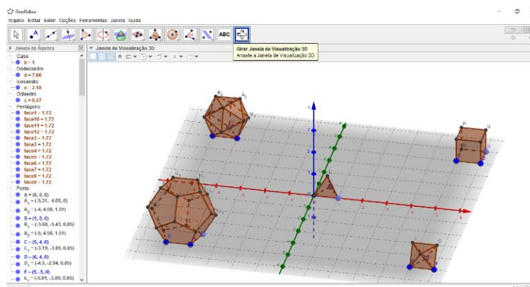
Figura 10: Os cinco poliedros regulares
