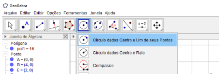
Figura 34: Formação dos círculos
