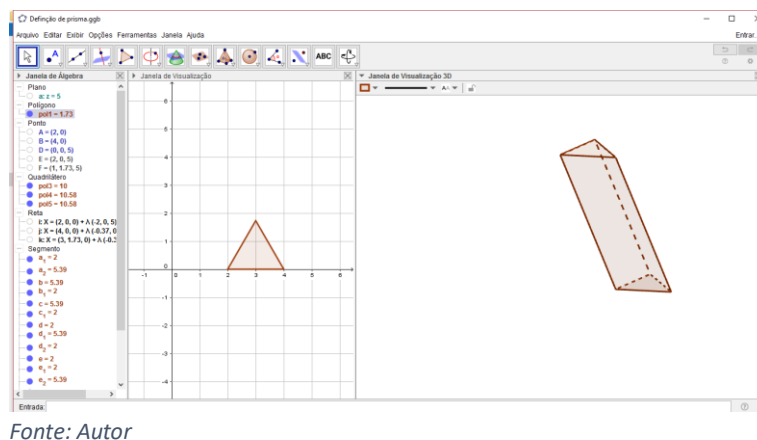
Figura 14: Visualização do prisma oblíquo de base triangular regular
