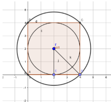
Figura 33: circunferências inscritas e circunscritas ao quadrado
