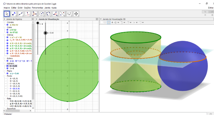
Figura 59: Interseção do plano com as superfícies do cilindro, do cone e da esfera
