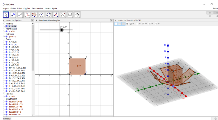
Figura 18: Controle deslizante e animação da planificação do prisma de base quadrada
