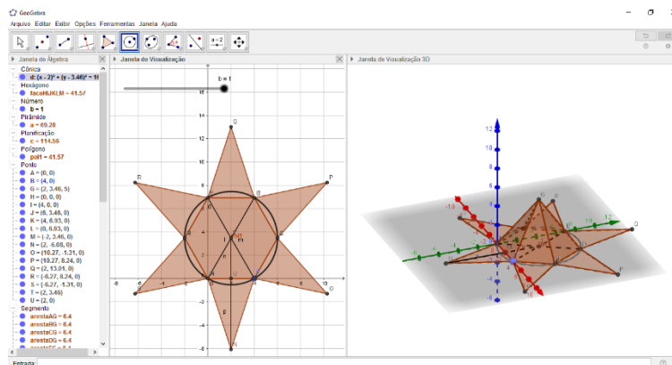
Figura 31: Base hexagonal regular inscrita na circunferência
