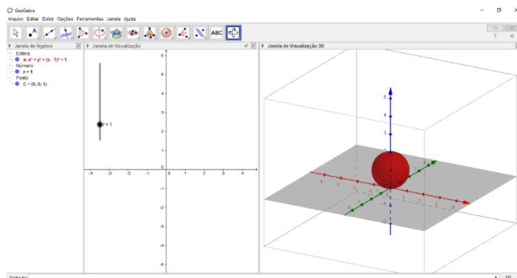
Figura 61: Esfera de raio variável (Teorema de Arquimedes)
