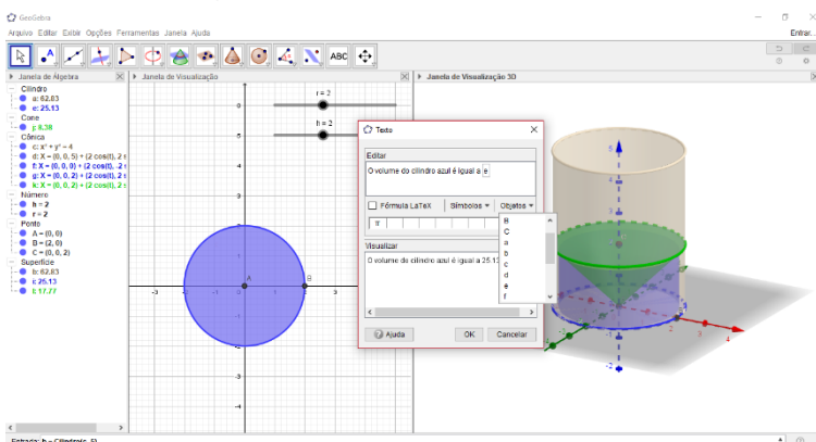
Figura 54: Exibição do valor do volume do cilindro
