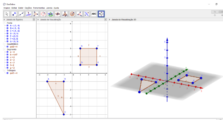
Figura 22: Bases quadrada e triangular retangular
