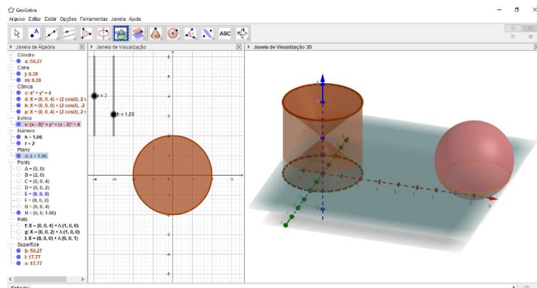
Figura 57: Plano secionando a esfera e o cone duplo interno ao cilindro
