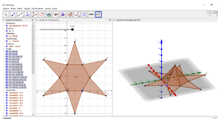
Figura 29: Pirâmide reta de base hexagonal regular, planificada
