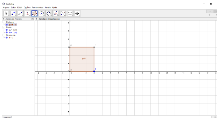
Figura 2: Base quadrada de lado 3
