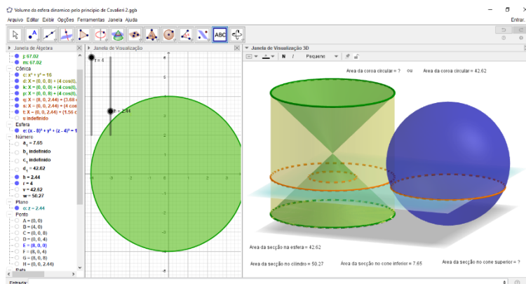
Figura 60: Exibição dos valores das áreas das seções do cilindro, do cone e da esfera
