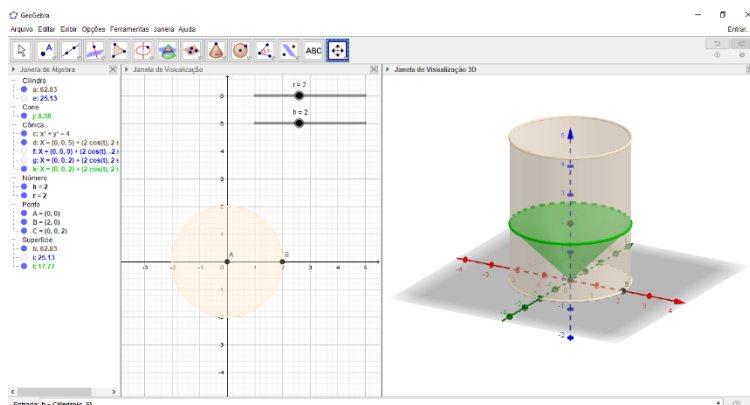
Figura 53: Cone circular reto de raio e altura variáveis
