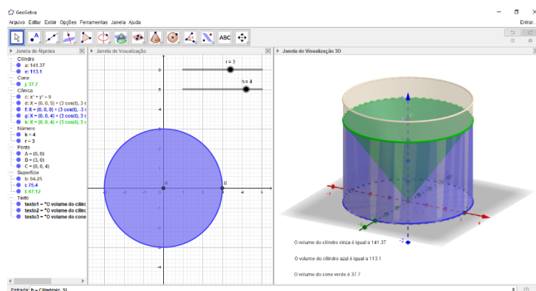
Figura 55: Exibição os valores dos volumes dos dois cilindros e do cone
