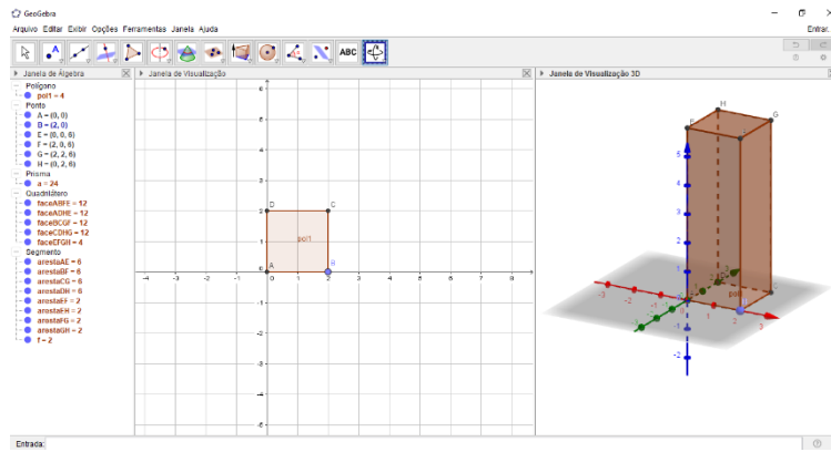
Figura 47: Prisma reto de base quadrada que compõe o tronco de pirâmide
