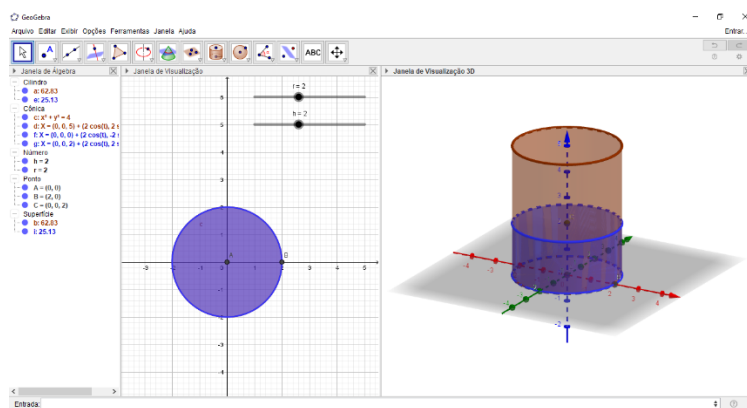
Figura 52: Cilindro circular reto de raio e altura variáveis
