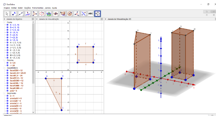
Figura 23: Prismas de bases quadrada e triangular retangular
