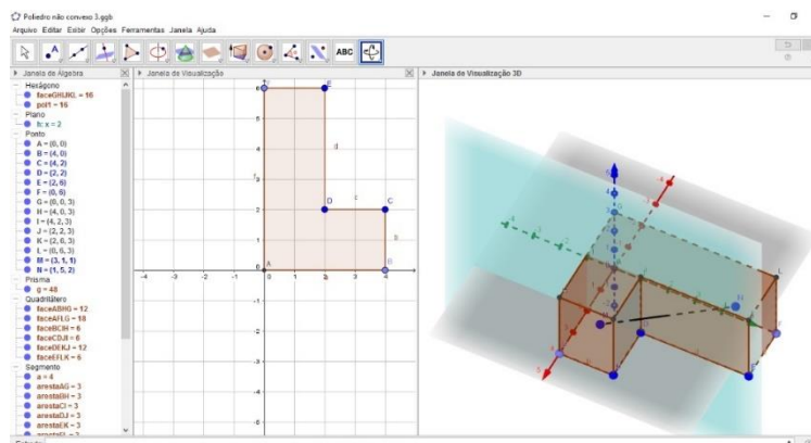
Figura 9: Segmento de reta que caracteriza um poliedro não convexo
