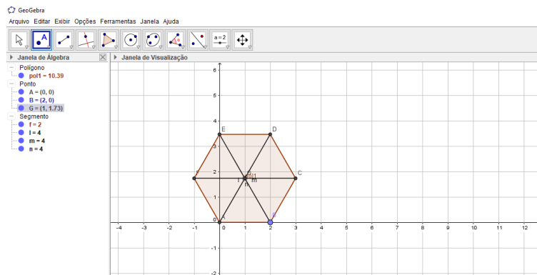
Figura 19: Diagonais e centro da base hexagonal regular
