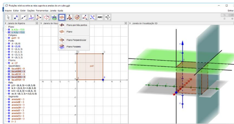
Figura 6: Planos suporte e suas respectivas posições relativas
