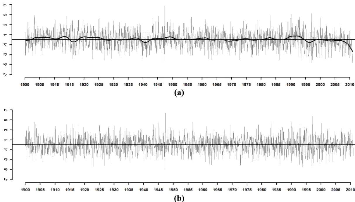
Figura 14- Análise da série temporal dos índices da Oscilação do Atlântico Norte (OAN) em (a) série dos índices da OAN e das tendências (linha suave) e em (b) a parte cíclica/aleatória, extraídas com o filtro Hodrick-Prescott.
