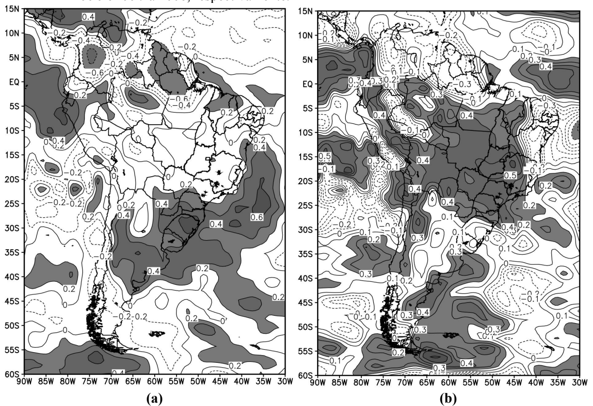
Figura 18- Coeficientes de correlações entre os índices da ODP e OMA e a taxa de precipitação para os períodos de estudo. As figuras da esquerda (a, c, e, g) são os coeficientes de correlações com o índice da ODP e as da direita (b, d, f, h) são os coeficientes de correlações com o índice da OMA para os períodos de 1948 a 1964, 1965 a 1977, 1978 a 1996 e 1997 a 2006, respectivamente.
