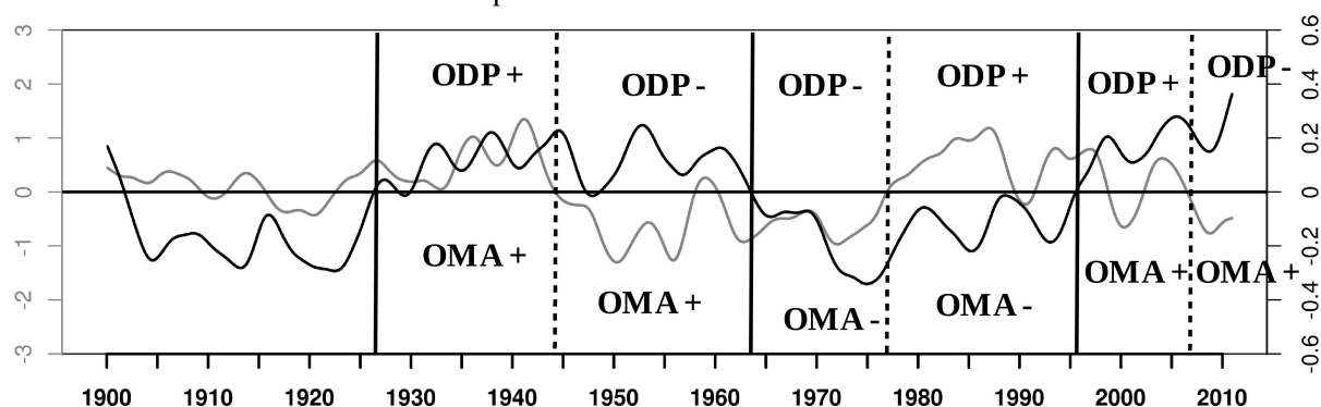
Figura 16- Tendências dos índices da ODP (em cinza) e da OMA (em negro) extraídas com o filtro Hodrick-Prescott do período de janeiro de 1900 a dezembro de 2010. As linhas verticais cheias e tracejadas representam, respectivamente, as divisões do modo positivo e negativo da OMA e as fases fria e quente da ODP.
