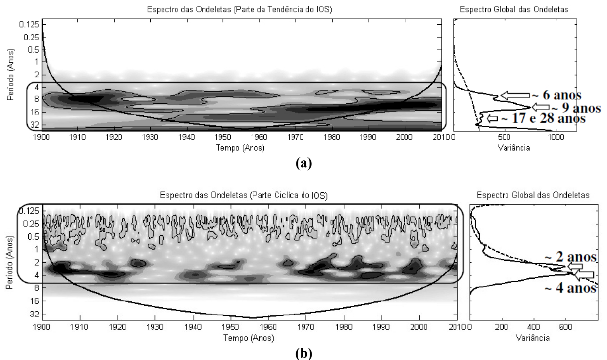
Figura 13- Análise das ondeletas aplicada às séries (a) das tendências e (b) da parte cíclica/aleatória, obtidas após o tratamento da série dos índices da OS com o filtro HP, com respectivos Espectros de Potências (EPO, esquerda) e Espectro Global das Ondeletas (EGO, direita).
