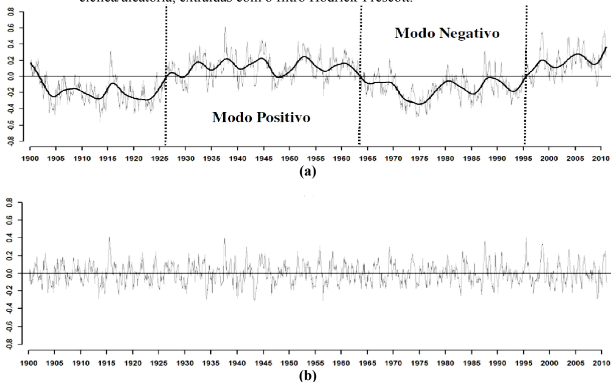
Figura 10- Análise da série temporal dos índices da Oscilação Multidecadal do Atlântico (OMA) em (a) série dos índices da OMA e das tendências (linha suave) e em (b) a parte cíclica/aleatória, extraídas com o filtro Hodrick-Prescott.
