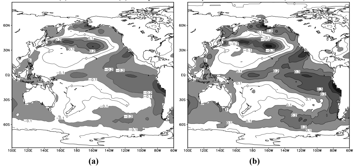
Figura 3- Anomalias da temperatura da superfície do mar (TSM) para a região do oceano Pacífico. Em (a) fase fria e em (b) fase quente da oscilação decadal do Pacífico (ODP).
