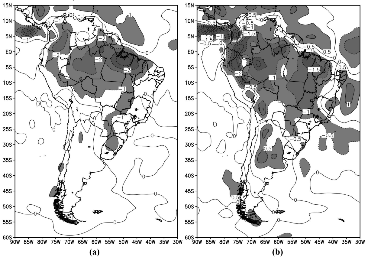
Figura 17: Anomalias anuais da taxa de precipitação ( \text{mm.dia}^{-1} ) sobre a América do Sul em relação ao período de 1981 à 2010. Em (a) 1948 à 1964 (ODP - e OMA +), em (b) 1964 à 1976 (ODP - e OMA -), em (c) 1976 à 1995 (ODP + e OMA -) e em (d) 1995 à 2006 (ODP + e OMA +).
