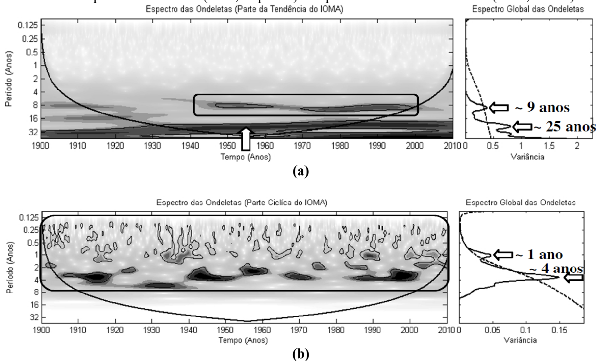
Figura 11- Análise das ondeletas aplicadas às séries (a) das tendências e (b) parte cíclica/aleatória, obtidas após tratamento da série dos índices de OMA com o filtro HP com os respectivos Espectro de Potência (EPO, esquerda) e Espectro Global das Ondeletas (EGO, direita).
