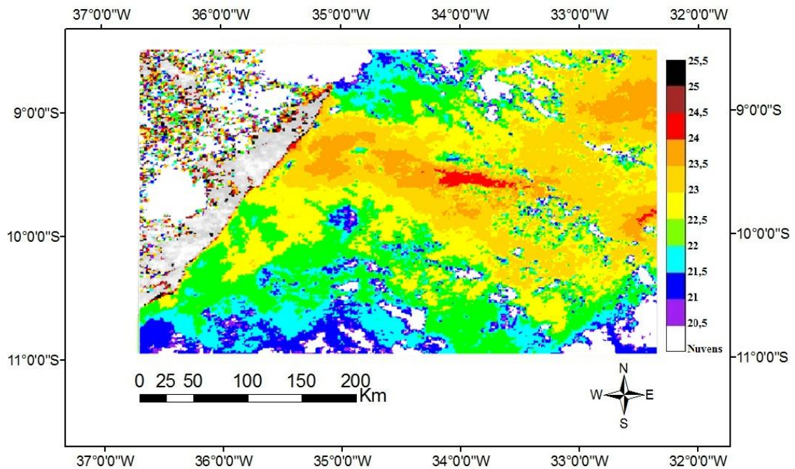
c) (T_b)_{b31} (°C) para o dia 30/01/2009 às 15:40 GMT.
