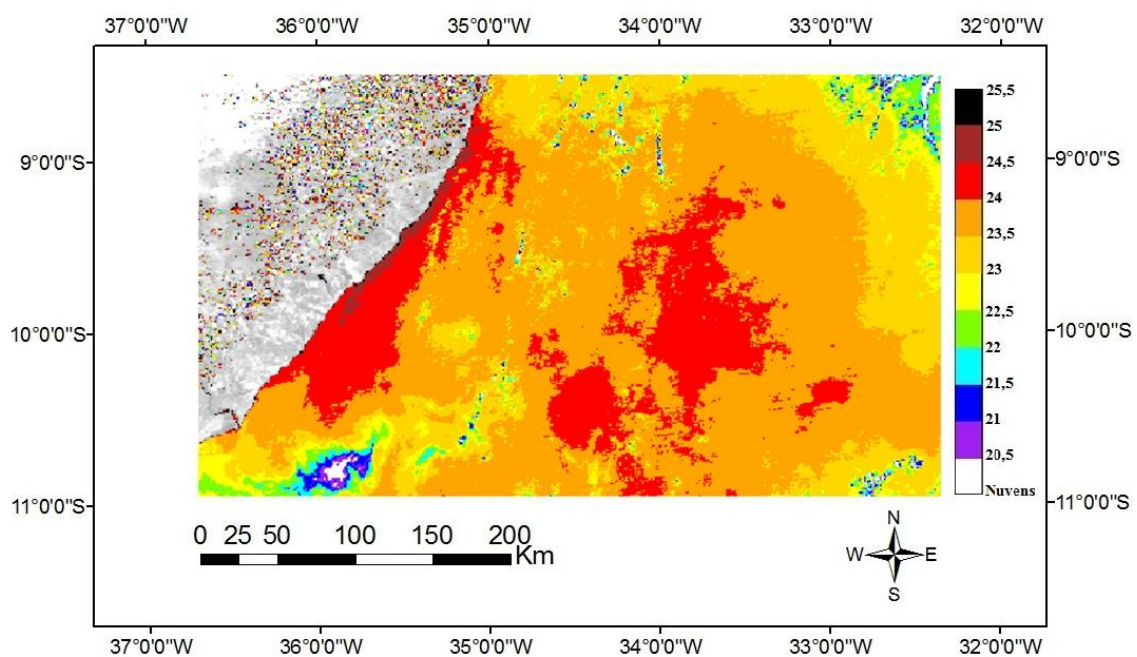
e) (T_b)_{b31} (°C) para o dia 16/11/2011 às 16:00 GMT.
