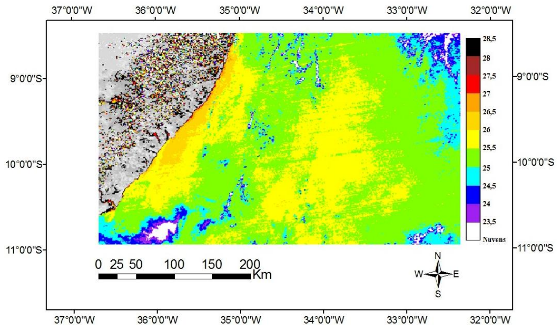
e) TSM (°C) para o dia 16/11/2011 às 16:00 GMT.
