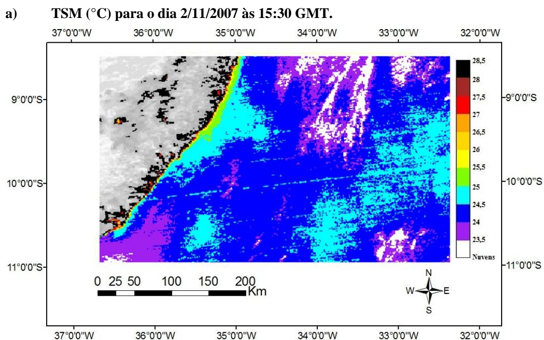
Figura 21 - Mapas temáticos da TSM (°C), utilizando-se dos coeficientes de calibração do algoritmo derivados de radiossondagens.
