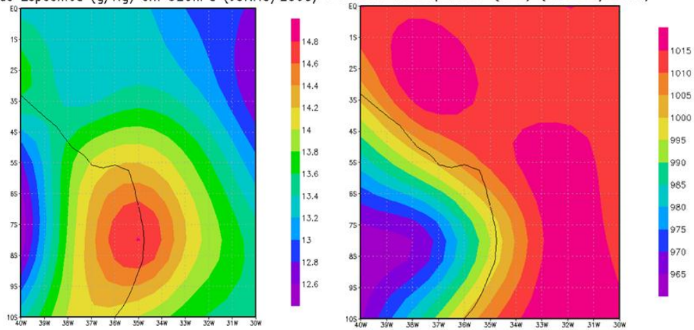
Umidade Específica (g/Kg) em 925hPa (JUNHO/2008) Pressao na Superficie (hPa) (AGOSTO/2010)
