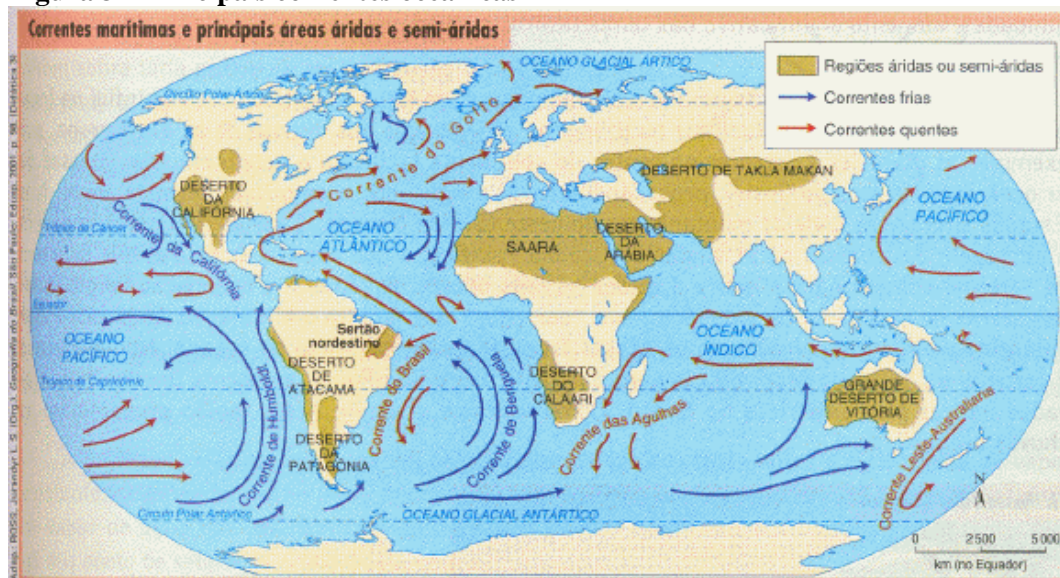
Figura 3 - Principais correntes oceânicas
