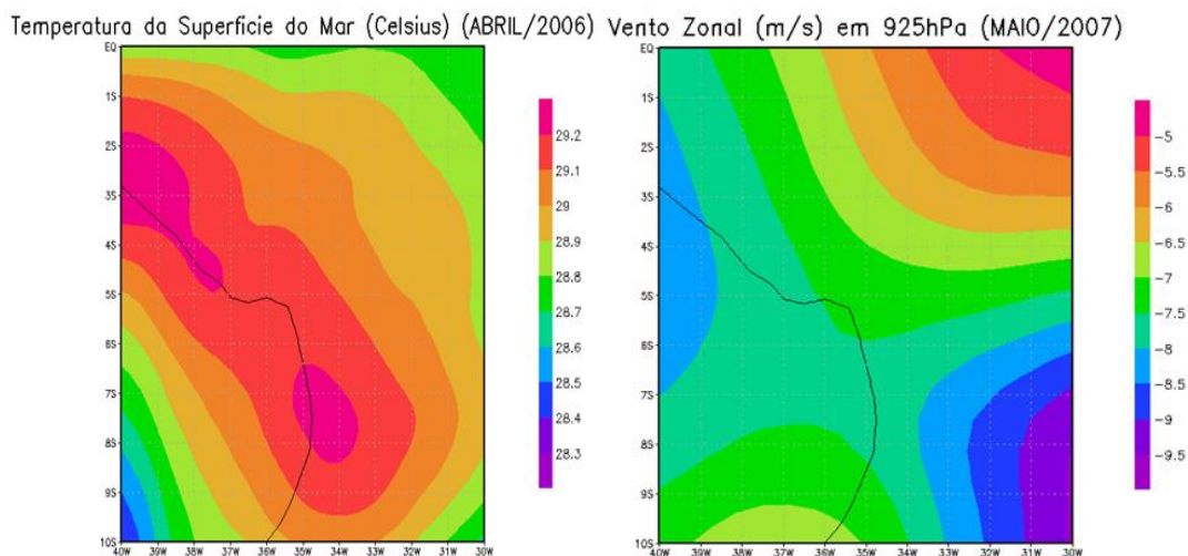
Figura 19 - Composições médias mensais obtidas através de dados de reanálise NCEP.
