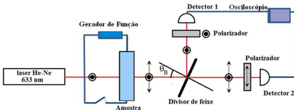
Figura 3.12: Ilustração do aparato experimental para determinar o tempo de comutação óptica das lâminas CL com alinhamento twist.
