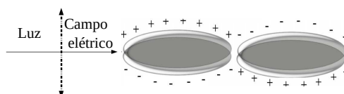
Figura 1.5: Ilustração do deslocamento de cargas elétricas, gerando um dipolo elétrico e a força restauradora criada devido a separação de cargas na partícula.
