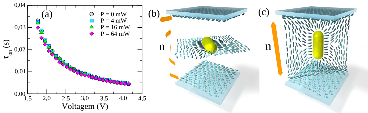
Figura 4.10: (a) Tempo de ativação característico \tau_{on} , em função da tensão aplicada para amostra 8CBNR2, excitada com feixe de laser \lambda = 785 nm. (b) Representação esquemática de nanobastões de ouro em células nemáticas torcidas no estado naturalmente desligado e (c) célula nemática torcida no estado eletricamente ligado.
