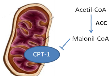
Figura 2. Inibição da Carnitina Palmitoil Transferase 1 (CPT-1) pelo Malonil-CoA. ACC: Acetil-CoA Carboxilase.
