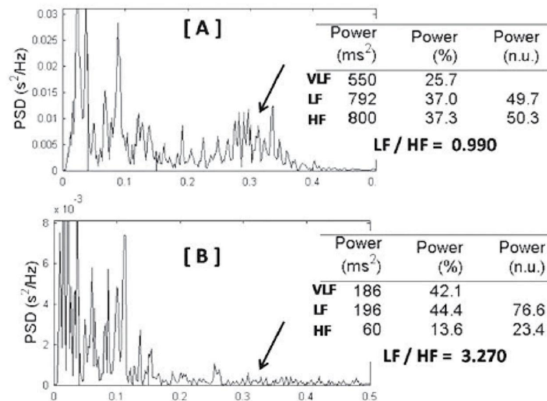
Fig. 5 Análise espectral de frequências ( Fast Fourier Transform ) de um adulto jovem normal (A) e de um recém-nascido normal (B). O componente de alta frequência (HF) está proporcionalmente bem mais reduzido no recém-nascido (setas) assim como a potência total (VANDERLEI et al. (5) ).
