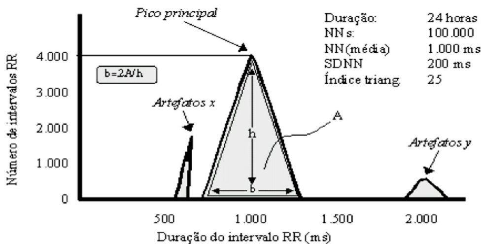
Fig. 2 Exemplo de histograma do intervalo RR (RASSI Jr (27) ).
