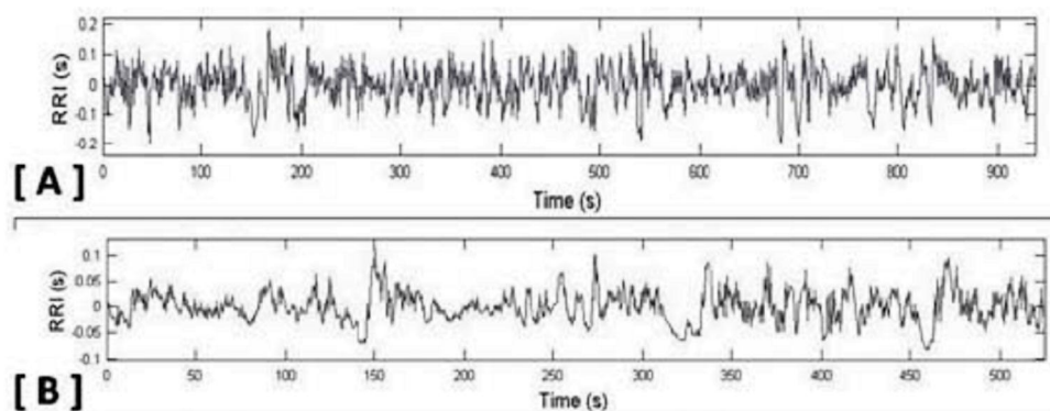
Fig. 1 Tacograma de um adulto jovem normal (A) e de um recém-nascido normal (B). A VFC está bem mais reduzida no painel B do que no painel A (VANDERLEI et al. , 2009)
