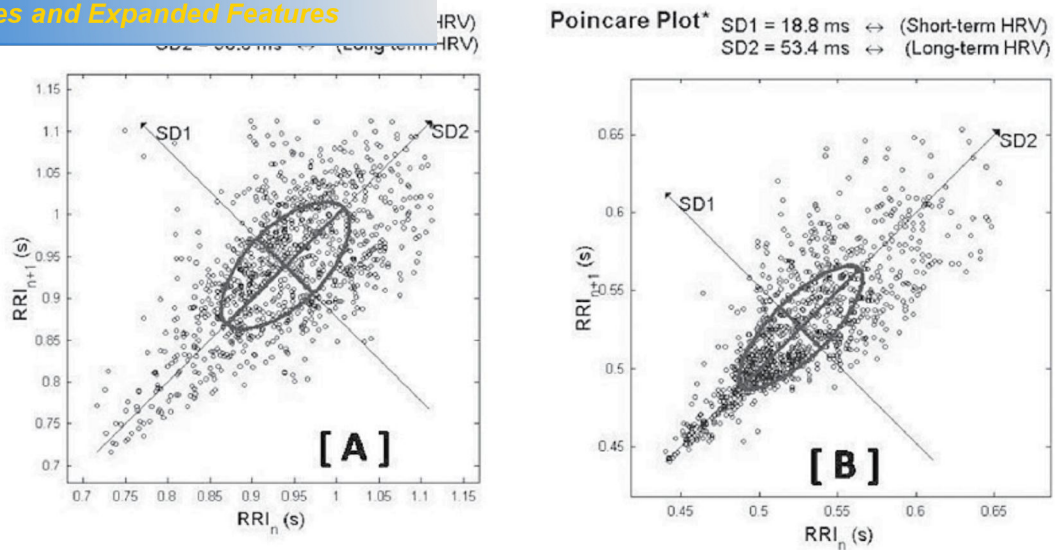
Fig. 3 Poincaré de um adulto jovem normal (A) e de um recém-nascido normal (B). A dispersão tanto de curto (SD1) quanto de longo prazo (SD2) no painel B está menor do que no painel A (VANDERLEI et al. (5) ).
