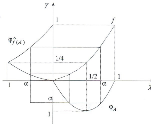
Figura 7 – Subconjunto \widehat{f}(A)
