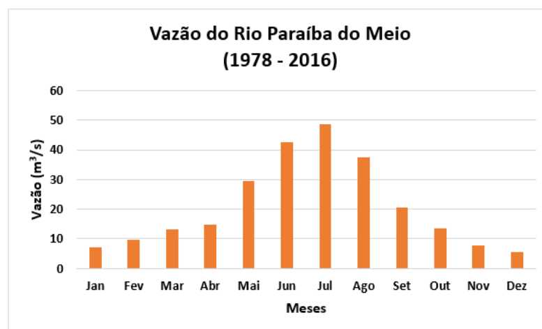
Figura 18: Dados históricos de vazão do Rio Paraíba do Meio da estação 39870000 localizada no município de Atalaia entre as coordenadas: latitude -9.50°; longitude -36.02°.
