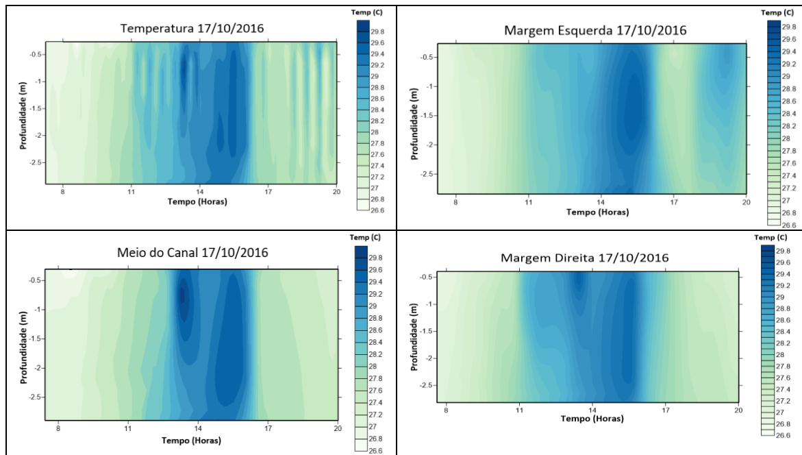
Figura 33: Distribuição espaço/temporal da temperatura no canal principal próximo à desembocadura da laguna Manguaba (Lat. 9° 43'57.27''S; Long. 35°49'20.47''W), durante 1 ciclo de maré, entre às 7:00 e 20:00 horas do dia 17/10/2016.
