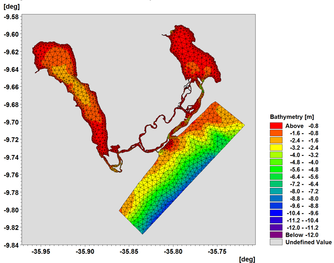
Figura 13: Detalhe da malha de discretização em elementos finitos e batimetria do CELMM
