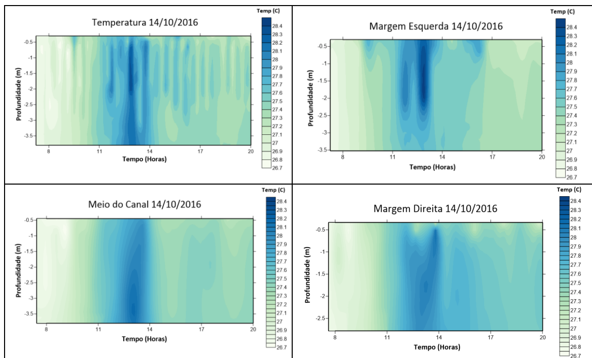
Figura 32: Distribuição espaço/temporal da temperatura no canal principal próximo à desembocadura da laguna Mundaú (Lat. 9° 42'30.58 S; Long. 35°47'47.35''W), durante 1 ciclo de maré, entre às 7:00 e 20:00 horas do dia 14/10/2016.
