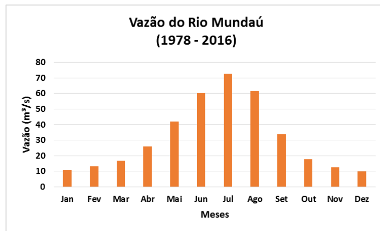
Figura 17: Dados históricos de vazão do Rio Mundaú da estação 39770000 localizada no município de Rio Largo entre as coordenadas: latitude -9.46°; longitude -35.85°.
