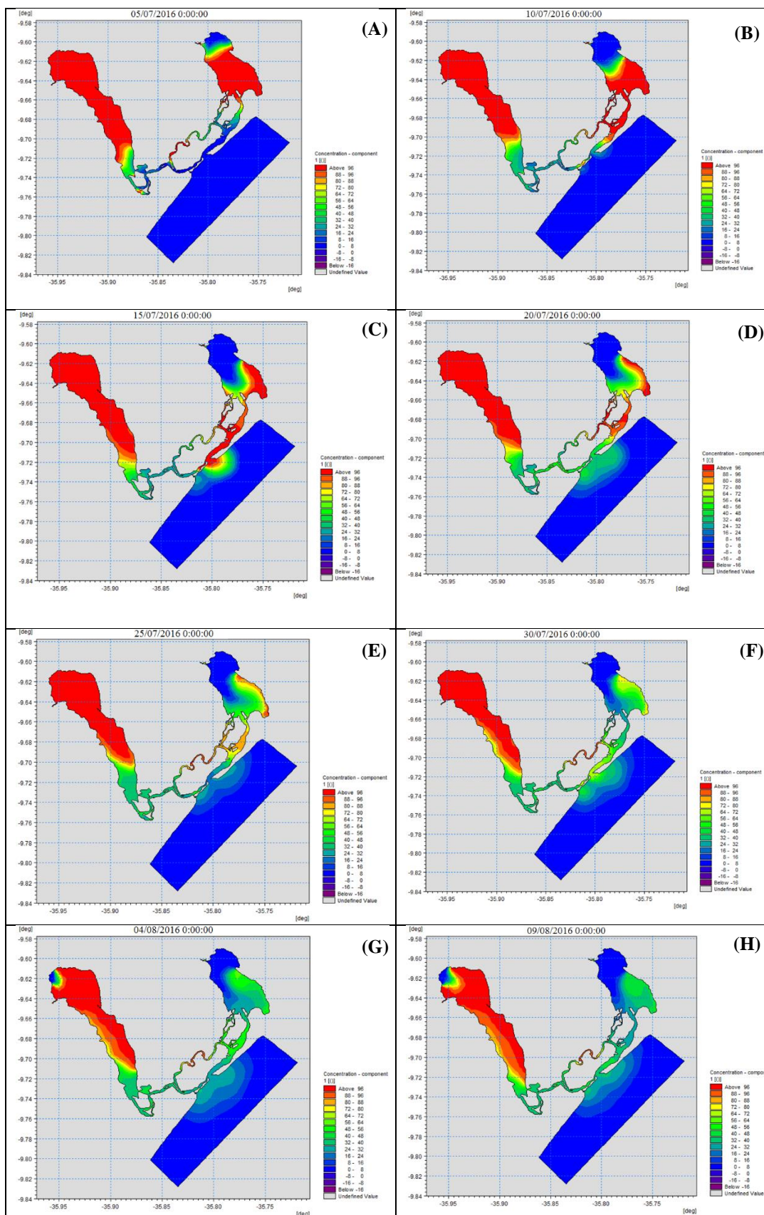
Figura 51: Mapas da distribuição de concentração do traçador calculado para o Complexo Estuarino Lagunar Mundaú Manguaba com dados reais a cada 5 dias.
