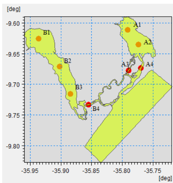
Figura 58: Localização da extração dos dados reais das correntes distribuídos espacialmente em 8 estações no CELMM. Laguna Mundaú: estação A1: Lat. -9.611; Long. -35.791; estação A2: Lat. -9.635; Long. -35.774; estação A3: Lat. -9.677; Long. -35.790; estação A4: Lat. -9.674; Long. -35.770. Laguna Manguaba: estação B1: Lat. -9.625; Long. -35.937; estação B2: Lat. -9.671; Long. -35.902; estação B3: Lat. -9.716; Long. -35.884; estação B4: Lat. -9.733; Long. -35.855.
