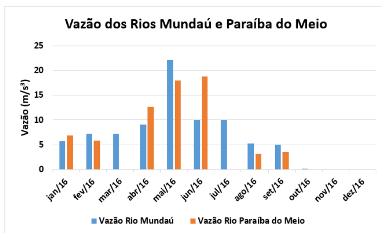
Figura 16: Dados reais de vazão dos Rios Mundaú e Paraíba do Meio para o ano de 2016.
