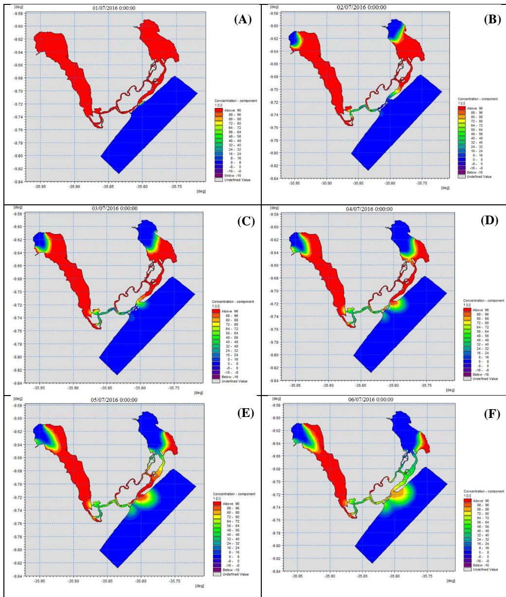
Figura 37: Mapas da distribuição de concentração do traçador calculado para o Complexo Estuarino Lagunar Mundaú Manguaba com dados históricos durante os primeiros dias.
