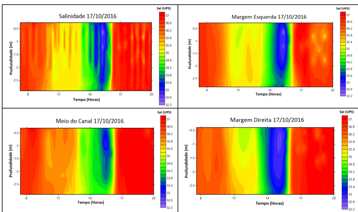
Figura 31: Distribuição espaço/temporal da salinidade no canal principal próximo à desembocadura da laguna Manguaba (Lat. 9° 43'57.27''S; Long. 35°49'20.47''W), durante 1 ciclo de maré, entre às 7:00 e 20:00 horas do dia 17/10/2016.
