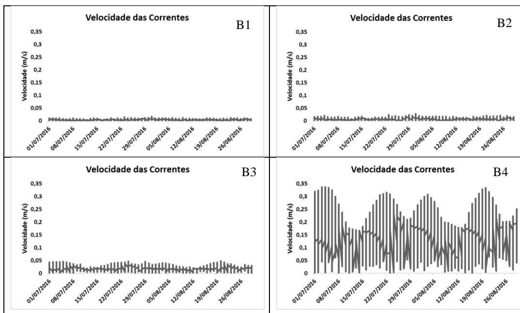
Figura 62: Dados reais de velocidades das correntes da laguna Manguaba e canal de ligação. Estação B1: Lat. -9.625; Long. -35.937; estação B2: Lat. -9.671; Long. -35.902; estação B3: Lat. -9.716; Long. -35.884; estação B4: Lat. -9.733; Long. -35.855.
