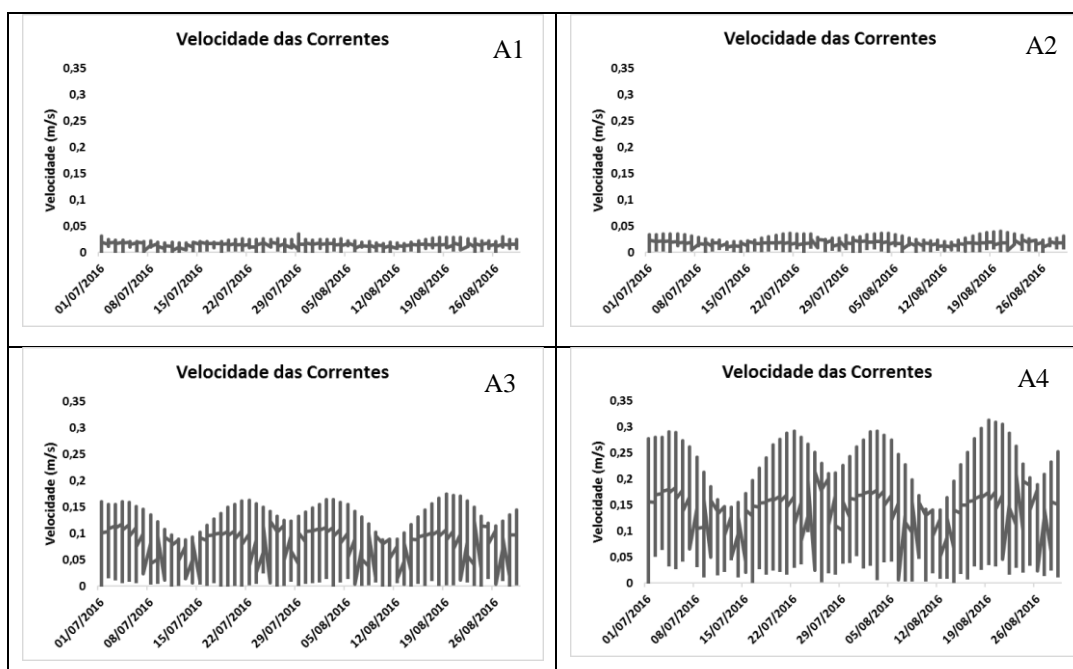
Figura 61: Dados reais de velocidades das correntes da laguna Mundaú e canais de ligação distribuídos espacialmente em 4 estações. Estação A1: Lat. -9.611; Long. -35.791; estação A2: Lat. -9.635; Long. -35.774; estação A3: Lat. -9.677; Long. -35.790; estação A4: Lat. -9.674; Long. -35.770.
