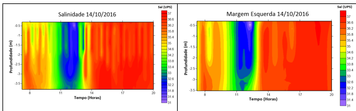
Figuras 30: Distribuição espaço/temporal da salinidade no canal principal próximo à desembocadura da laguna Mundaú (Lat. 9° 42'30.58 S; Long. 35°47'47.35''W), durante 1 ciclo de maré, entre às 7:00 e 20:00 horas do dia 14/10/2016.
