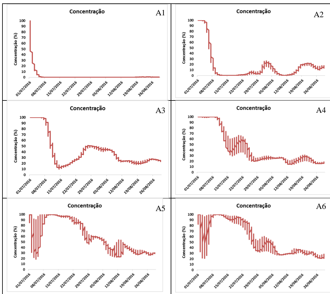
Figura 53: Dados reais de concentração da laguna Mundaú e canais de ligação distribuídos espacialmente em 6 estações. Estação 1: Lat. -9.599; Long. -35.794; estação 2: Lat. -9.616; Long. -35.789; estação 3: Lat. -9.629; Long. -35.778; estação 4: Lat. -9.645; Long. -35.775; estação 5: Lat. -9.677; Long. -35.790; estação 6: Lat. -9.674; Long. -35.770.
