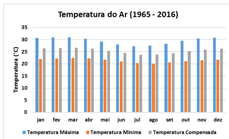
Figura 8: Dados históricos de temperatura da estação 82994 localizada no município de Maceió entre as coordenadas: latitude -9.66; longitude -35.7.
